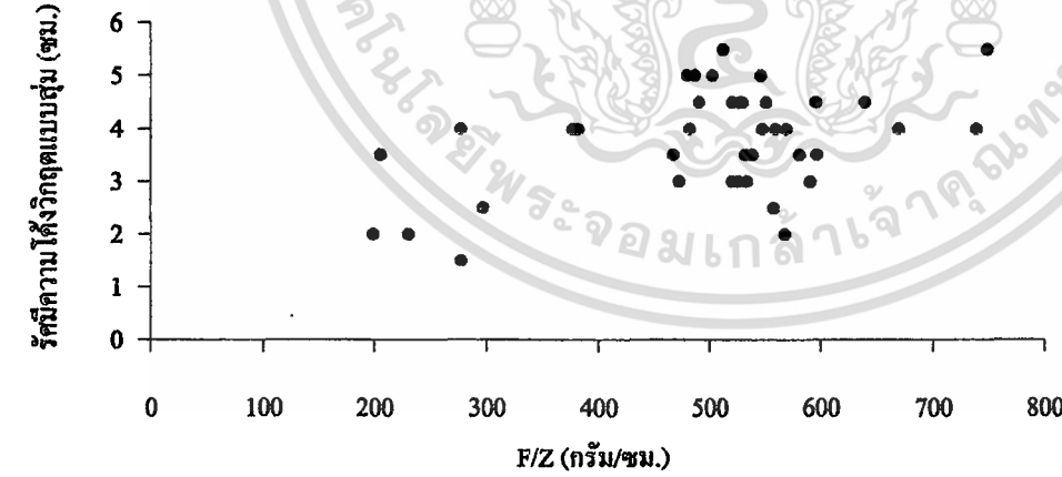
ภาพที่4.2 แสดงความสัมพันธ์ระหว่างรัศมีความโค้งวิกฤตแบบคู่กับค่า Bending Elastic Parameter ( F/Z )
