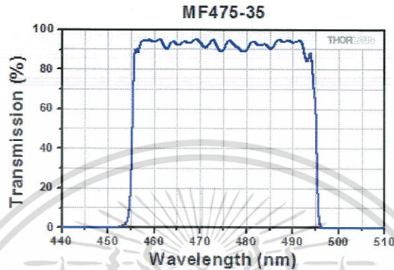
รูปที่ 3.4 ภาพคุณสมบัติการกรองความยาวคลื่นแสงของตัวกรอง MF475-35
