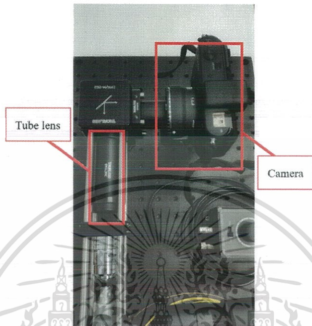
รูปที่ 4.3 รูปส่วนของระบบการรับภาพโดยใช้กล้องดิจิทัล
