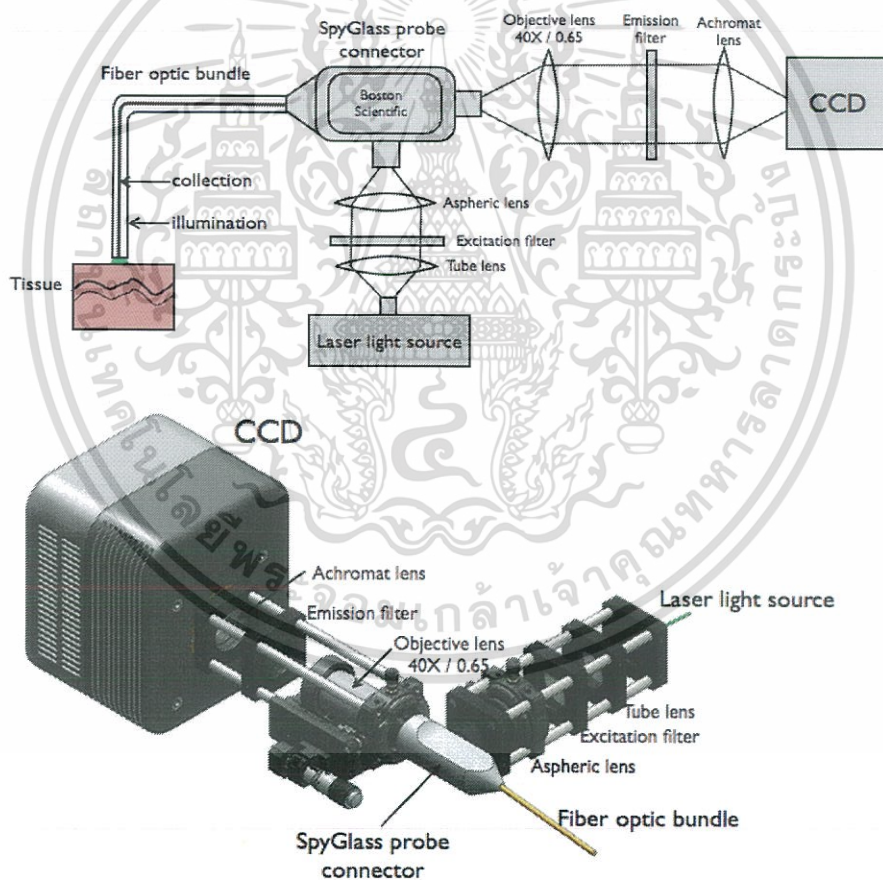
รูปที่ 3.1 ภาพรวมของระบบกล้องจุลทรรศน์แบบหลายความยาวคลื่นแสง
