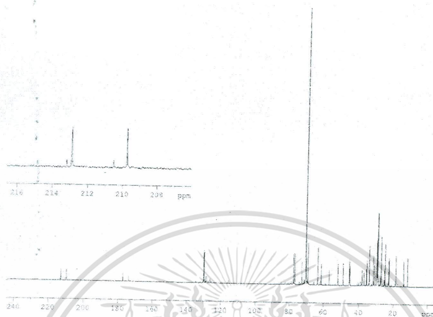
รูปที่ 3.7 สเปกตรัม ^{13}\text{C} NMR ของสารสกัดหยาบจากปฏิกิริยาระหว่างกรดไฮโดรคลอริก 14 และเชื้อรา F. solani TISTR 3436 ในอาหารเหลวสูตร 3% glucose : 1% peptone วันที่ 7
