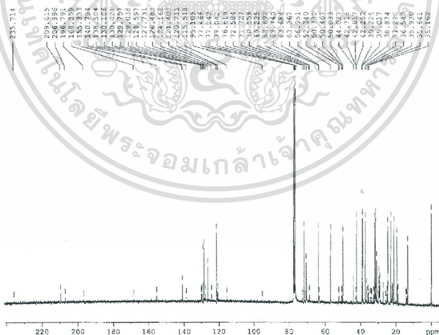
รูปที่ ผ. 10 ^{13}\text{C} NMR สเปกตรัมของสารสกัดหยาบจากปฏิกิริยาระหว่างเพรกนินโนโลน 1 และเชื้อ F. solani TISTR 3436 ในวันที่ 7
