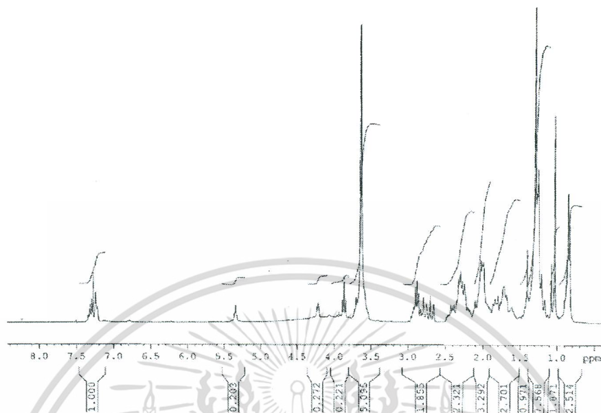
รูปที่ ๕ ^1\text{H} NMR สเปกตรัมของสารสกัดหยาบจากปฏิกิริยาระหว่างกรดไฮโดรโคลิค 14 และเชื้อ F. solani TISTR 3436 ในวันที่ 7
