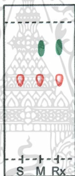
รูปที่ 3.14 แผ่นทินเลเยอร์โครมาโทกราฟีของกรดไฮโดรโคลิก 14 เปรียบเทียบกับสารสกัดหยาบ S หมายถึงสารตั้งต้น; M หมายถึง จุดผสมระหว่างสารตั้งต้นและสารสกัดหยาบ; Rx หมายถึง สารสกัดหยาบจากปฏิกริยาระหว่างกรดไฮโดรโคลิก 14 กับเชื้อรา
