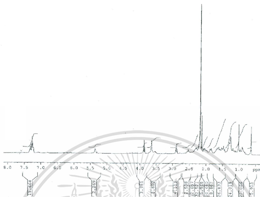
รูปที่ ผ. 9 ^1\text{H} NMR สเปกตรัมของสารสกัดหยาบจากปฏิกิริยาระหว่างเพรกนินโนโลน 1 และเชื้อ F. solani TISTR 3436 ในวันที่ 7
