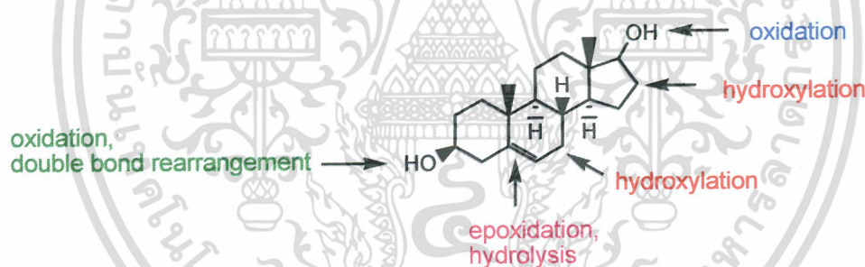
รูปที่ 1.1 แสดงตำแหน่งคาร์บอนของสเตียรอยด์ที่เกิดกระบวนการเปลี่ยนแปลงทางเคมี โดยใช้จุลินทรีย์
