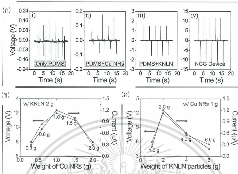
รูปที่ 2.44 (ก) ผลศักย์ไฟฟ้าส่งออกจากอุปกรณ์ที่ถูกสร้างขึ้น (i) ใช้เพียง PDMS (ii) วัสดุผสมแท่งนาโนทองแดง Cu/PDMS (iii) วัสดุผสมที่มีเฉพาะอนุภาคอัลคาไลไนโอเบต (iv) อุปกรณ์ NCG (ข) การเปลี่ยนแปลงของศักย์ไฟฟ้าส่งออกและกระแสจากอุปกรณ์ NCG ภายใต้ปริมาณของอนุภาคอัลคาไลไนโอเบตคงที่ (ค) การเปลี่ยนแปลงของศักย์ไฟฟ้าส่งออกและกระแสจากอุปกรณ์ NCG ภายใต้ปริมาณแท่งนาโนทองแดงคงที่ [21]
