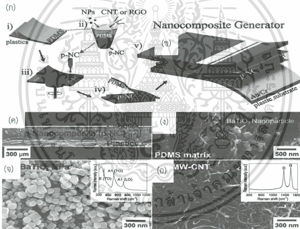
รูปที่ 2.38 (ก) กระบวนการผลิตตัวกำเนิดนาโนคอมโพสิต (ข) ภาพ SEM แบบตัดขวางของตัวกำเนิดนาโนคอมโพสิต (ค) ภาพ SEM แบบตัดขวางที่ขยายแสดงอนุภาคของนาโนคอมโพสิต (ง) ภาพ SEM ของอนุภาคนาโน BT ที่สังเคราะห์ด้วยวิธีไฮโดรเทอร์มอล (Hydrothermal method) (จ) สเปกตรัมรามาน ที่ได้จากอนุภาคนาโน BT (ฉ) MWCNT มีขนาดเส้นผ่าศูนย์กลาง 20 นาโนเมตรและความยาวของ 2 ไมครอน รูปประกอบแสดงให้เห็นถึงการเปลี่ยนแปลงของสเปกตรัมรามานของ MWCNT กับกลุ่ม D ขนาดใหญ่ [20]
