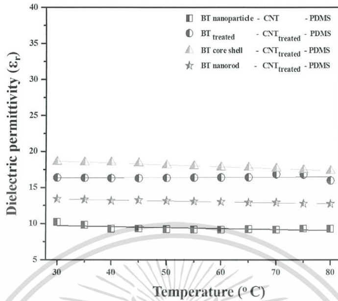
รูปที่ 4.19 ความสัมพันธ์ระหว่างค่าคงที่ไดอิเล็กทริกกับอุณหภูมิของวัสดุผสม BT - CNT - PDMS วัสดุผสม BT treated -CNT treated -PDMS วัสดุผสม BT nanorod -CNT treated -PDMS และวัสดุผสม BT coreshell -CNT treated -PDMS
