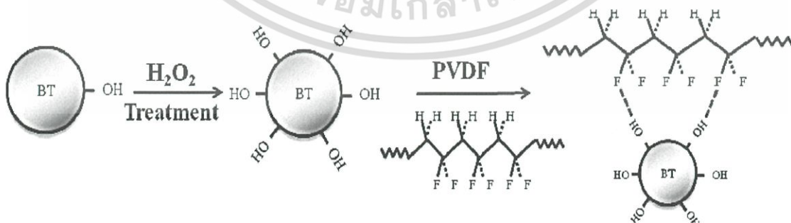
รูปที่ 2.27 การเกิดอันตรกิริยาของ BT ที่ปรับปรุงพื้นผิวด้วย H_2O_2 การเกิดคอมโพสิตกับ PVDF และการก่อตัวของพันธะไฮโดรเจนในนาโนคอมโพสิต BT/PVDF [18]
