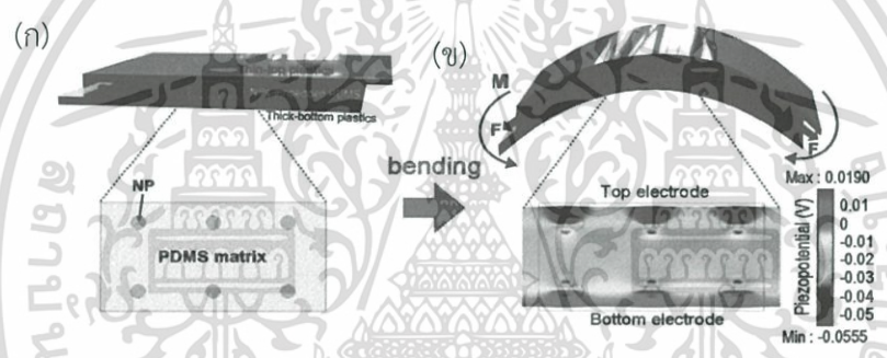
รูปที่ 2.40 (ก) การจำลองรูปแบบของอุปกรณ์ตัวกำเนิดนาโนคอมโพสิต โครงสร้างทั้ง 6 จุด ของ BT ผังตัวบนพอลิเมอร์เมทริกซ์ PDMS (ข) จำลองความแตกต่างภายใน PDMS ระหว่างด้านบนและด้านล่างขั้วไฟฟ้าส่งผลต่อค่าเพียโซอิเล็กทริก [20]
