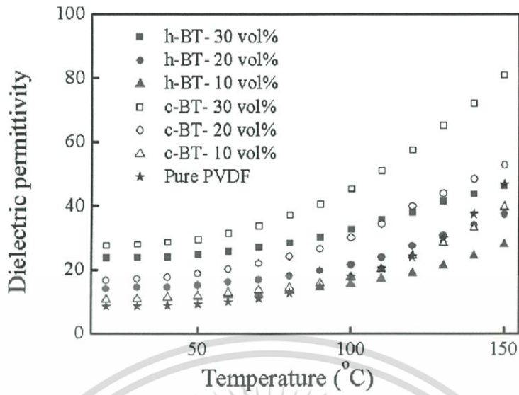
รูปที่ 2.28 ค่าสภาพยอมสัมพันธ์เทียบกับอุณหภูมิระหว่างนาโนคอมโพสิตของ c-BT/PVDF และ BT/PVDF ความเข้มข้นของสารต่างกัน ที่ 100 Hz [18]
