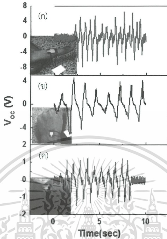
รูปที่ 2.35 การกักเก็บพลังงานการตรวจวัด V_{oc} ตัวกำเนิดเพียโซอิเล็กทริกนาโนคอมโพสิต ที่ความเข้มข้น 40 wt% BT โดยนำตัวกำเนิดเพียโซอิเล็กทริกนาโนคอมโพสิตมาแปะติดกับ (a) นิ้วมือ (b) ข้อมือ (c) ข้อพับ [19]
