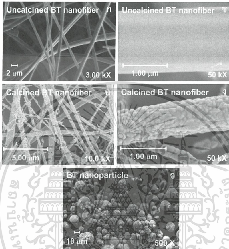
รูปที่ 4.26 ลักษณะทางสัณฐานวิทยาของ (ก) และ (ข) เส้นใยนาโน BT ก่อนเผา (ค) และ (ง) เส้นใยนาโน BT หลังเผา และ (จ) ลักษณะอนุภาคนาโน BT เกรดการค้า
