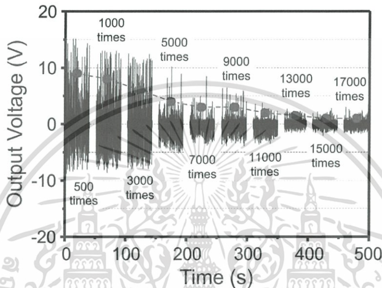
รูปที่ 4.35 แรงดันไฟฟ้าส่งออกของวัสดุผสมเพียโซอิเล็กทริกยึดหยุ่นได้ที่มีวิธการกระจายตัว คือ อนุภาคนาโน BT และเส้นใยนาโน BT ที่อัตราส่วนที่ให้แรงดันไฟฟ้าส่งออกสูงที่สุดคือ 50%:50% โดยให้แรงเชิงกลอย่างต่อเนื่องทั้งหมด 10 รอบ 17000 ครั้ง
