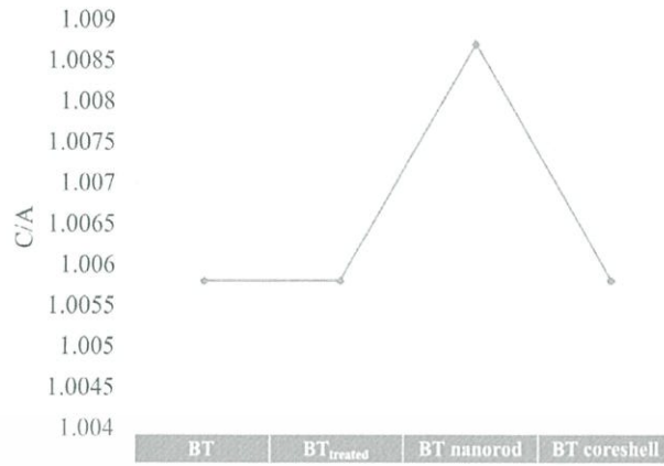
รูปที่ 4.4 แสดงอัตราส่วนระหว่างค่าแลตทิซพารามิเตอร์ c ต่อ a
