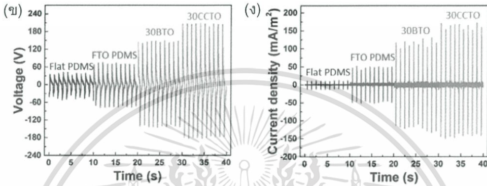
รูปที่ 2.52 (ก) โครงสร้าง FPEH ที่ถูกออกแบบขึ้น และผลทางไฟฟ้าขาออกสำหรับ (ข) แรงดัน และ (ค) กระแสไฟฟ้า (ปรับแต่งจาก [28])
