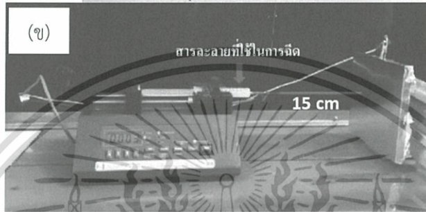
รูปที่ 4.24 ชุดการผลิตเส้นใยด้วยไฟฟ้าสถิต (ก) เครื่องกำเนิดศักย์ไฟฟ้า (ข) ตำแหน่งของการติดตั้งเครื่องมือในการผลิตเส้นใย
