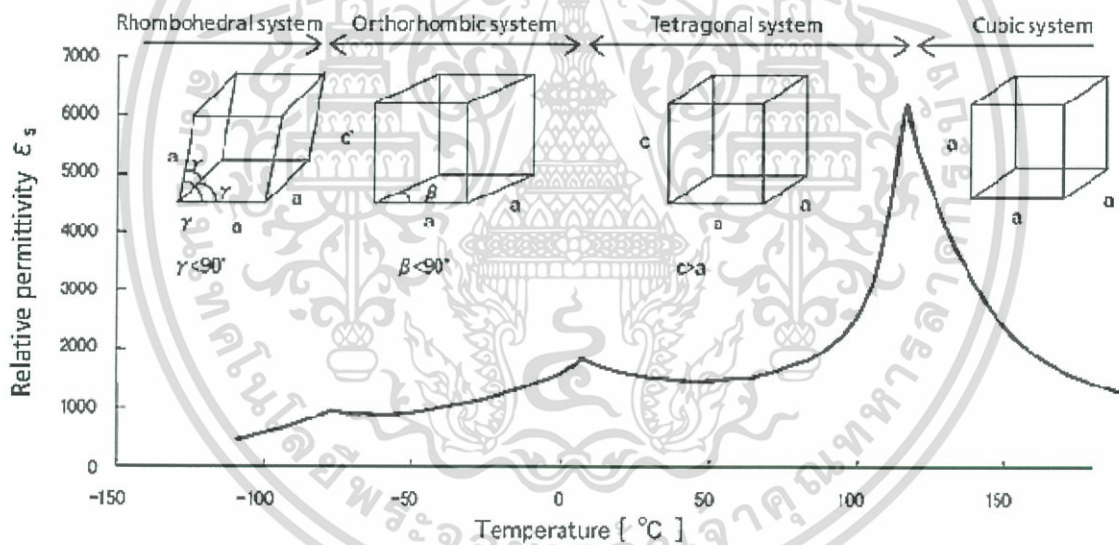
รูปที่ 2.6 ความสัมพันธ์ระหว่างค่าสภาพยอมสัมพัทธ์ กับอุณหภูมิของผลึก BT [1]
