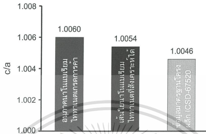
รูปที่ 4.29 อัตราส่วนระหว่างค่าความเป็นเตตระโกนอลของวัสดุกระจายตัวของอนุภาคนาโน BT และเส้นใยนาโน BT
