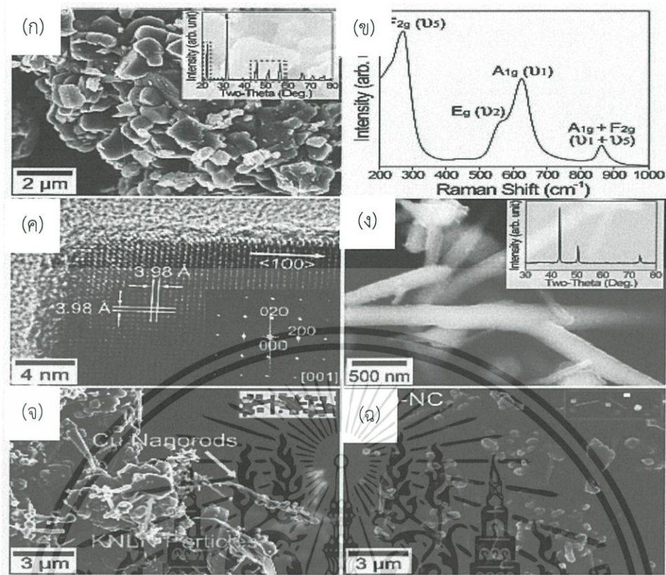
รูปที่ 2.43 (ก) ภาพถ่าย SEM ของอนุภาคอัลคาไลไนโอเบตที่ถูกสังเคราะห์ขึ้นจากปฏิกิริยาสถานะของแข็ง (ข) สเปกตรัมรามานของอนุภาคอัลคาไลไนโอเบตที่แสดงโครงสร้างผลึกเพอรอฟสไกต์ของวัภาคเตตระโกนอล (ค) ภาพ HRTEM ของอนุภาคอัลคาไลไนโอเบต (ง) ภาพแสดง SEM และกราฟ XRD ของแท่งนาโนทองแดง (จ) ภาพขยาย SEM ของวัสดุนาโนประกอบด้วยอนุภาคอัลคาไลไนโอเบต และแท่งนาโนทองแดงก่อนผสม PDMS (ฉ) ภาพแสดง SEM ของภาคตัดขวางของวัสดุผสม [21]
