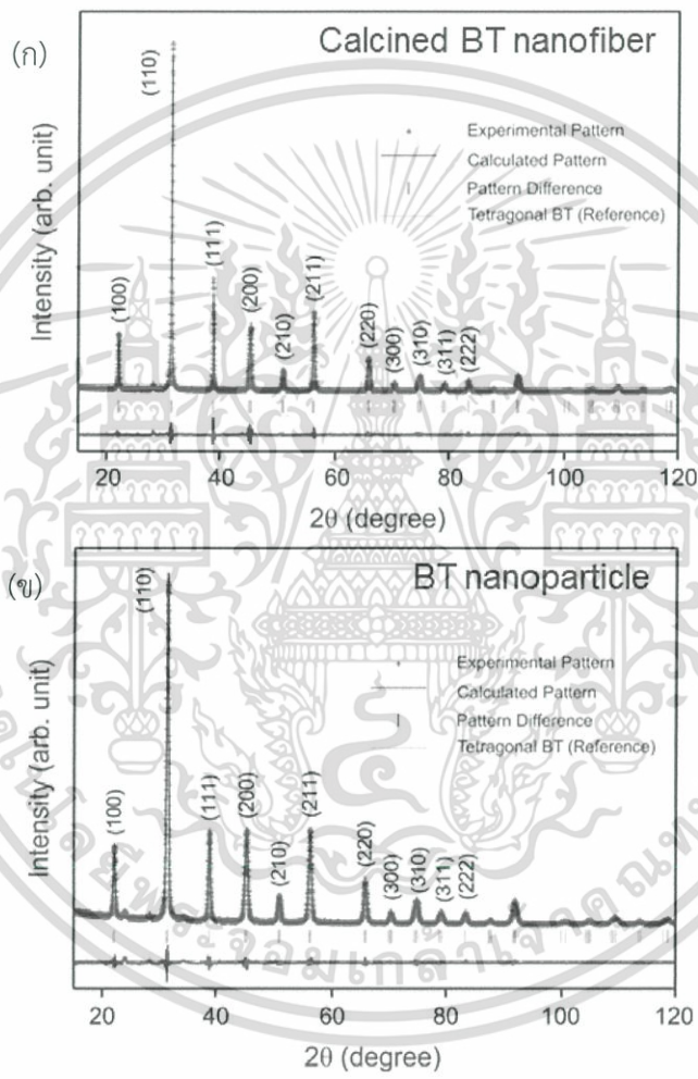
รูปที่ 4.28 รูปแบบการเลี้ยวเบนรังสีเอ็กซ์หลังผ่านการวิเคราะห์โครงสร้างด้วยวิธีรีตเวลดต์โดยการใช้ซอฟต์แวร์ JANA 2006 (ก) เส้นใยนาโน BT (ข) อนุภาคนาโน BT
