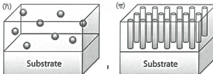
รูปที่ 2.22 วัสดุผสมระหว่างพอลิเมอร์กับเซรามิก (ก) แบบ 0-3 (ข) แบบ 1-3 [9]
