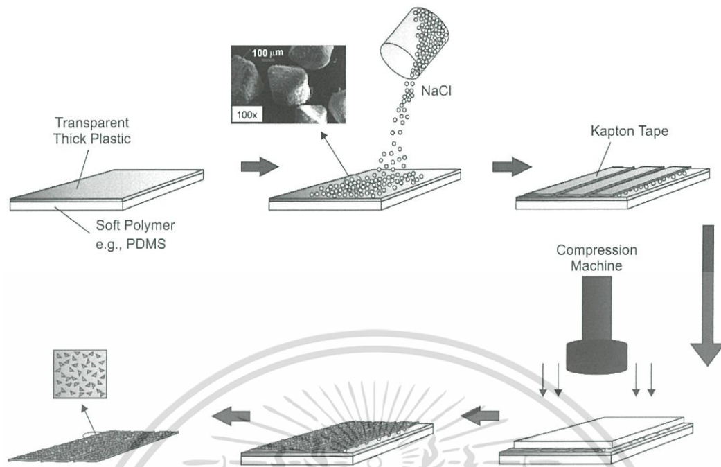
รูปที่ 3.3 กระบวนการสร้างความขรุขระบนพื้นผิววัสดุโพลีเอทิลีนทริกด้วยเทคนิค CC
