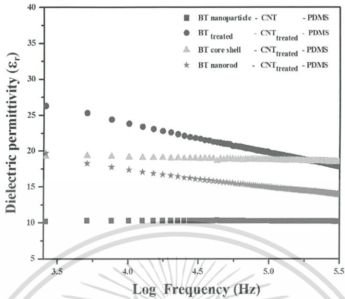
รูปที่ 4.17 ความสัมพันธ์ระหว่างค่าคงที่ได้โอเล็กทริกกับค่าความถี่ของวัสดุผสม BT - CNT - PDMS วัสดุผสม BT treated -CNT treated -PDMS วัสดุผสม BT nanorod -CNT treated -PDMS และวัสดุผสม BT coreshell -CNT treated -PDMS
