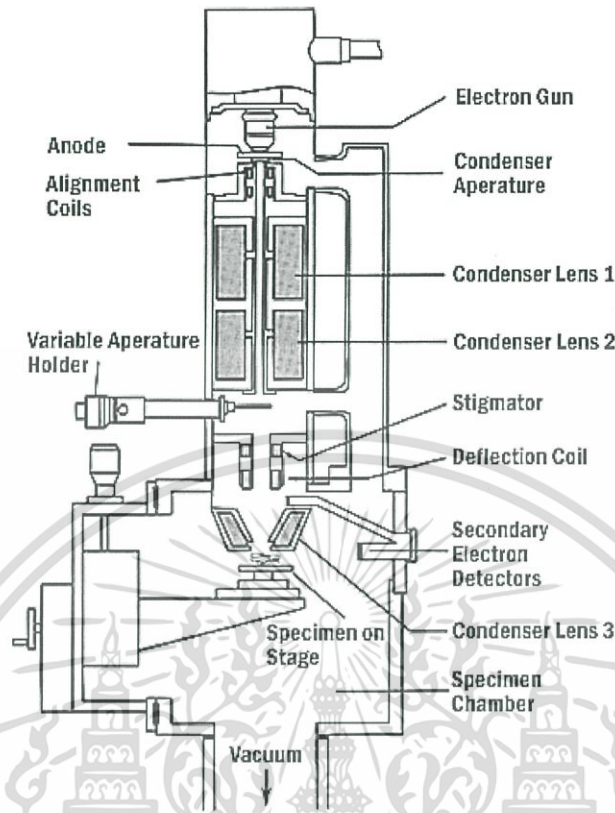
รูปที่ 3.8 แสดงส่วนประกอบของ SEM
