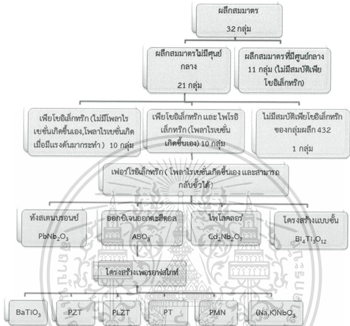
รูปที่ 2.1 การจำแนกกลุ่มของผลึกโดยใช้พื้นฐานของสมมาตรผลึก [1]
