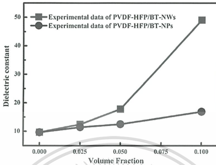
รูปที่ 2.24 ค่าคงที่ไดอิเล็กทริกของวัสดุผสมที่มีเฟสกระจายตัวเป็น BT - NP และวัสดุผสมที่มีเฟสกระจายตัวเป็น BT - NW โดยมีเฟสเนื้อหลักเป็น PVDF - HFP [11]
