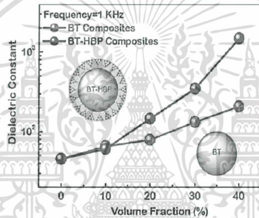
รูปที่ 2.23 ค่าคงที่ไดอิเล็กทริกของวัสดุผสมที่มีเฟสกระจายตัวเป็นอนุภาค BT (BT - NP) และ BT ที่มีโครงสร้างแบบคอร์เชลล์ (BT-HBP) และเฟสเนื้อหลักเป็น PVDF-TrFE-CFE [10]
