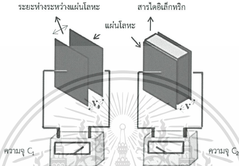
รูปที่ 2.8 การวัดค่าไดอิเล็กทริกสัมภาคระหว่างแผ่นตัวเก็บประจุคู่ขนาน (ก) สัมภาค (ข) สารไดอิเล็กทริกระหว่างแผ่นตัวเก็บประจุคู่ขนาน ตัวเก็บประจุที่มีสารไดอิเล็กทริกมีค่าความต่างศักย์ (V) น้อยกว่าค่าความต่างศักย์ของสัมภาค ( V_0 ) ดัดแปลงจาก [1]
