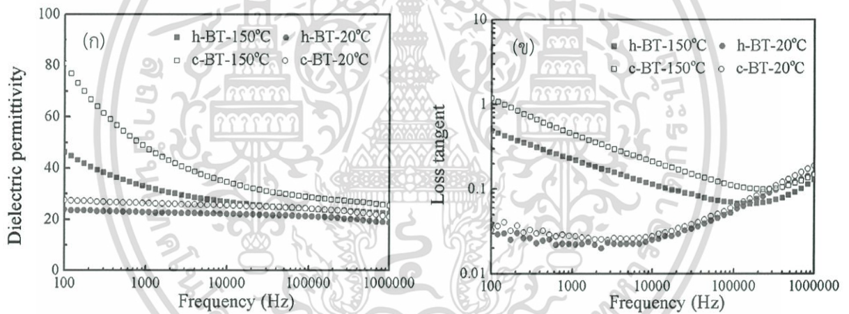
รูปที่ 2.29 (ก) ค่าสภาพยอมสัมพันธ์ (ข) ค่าการสูญเสียไดอิเล็กทริกของนาโนคอมโพสิต c-BT/PVDF และ BT/PVDF ที่ความเข้มข้น 30 vol% BT ที่อุณหภูมิต่างกัน เทียบกับความถี่ [18]
