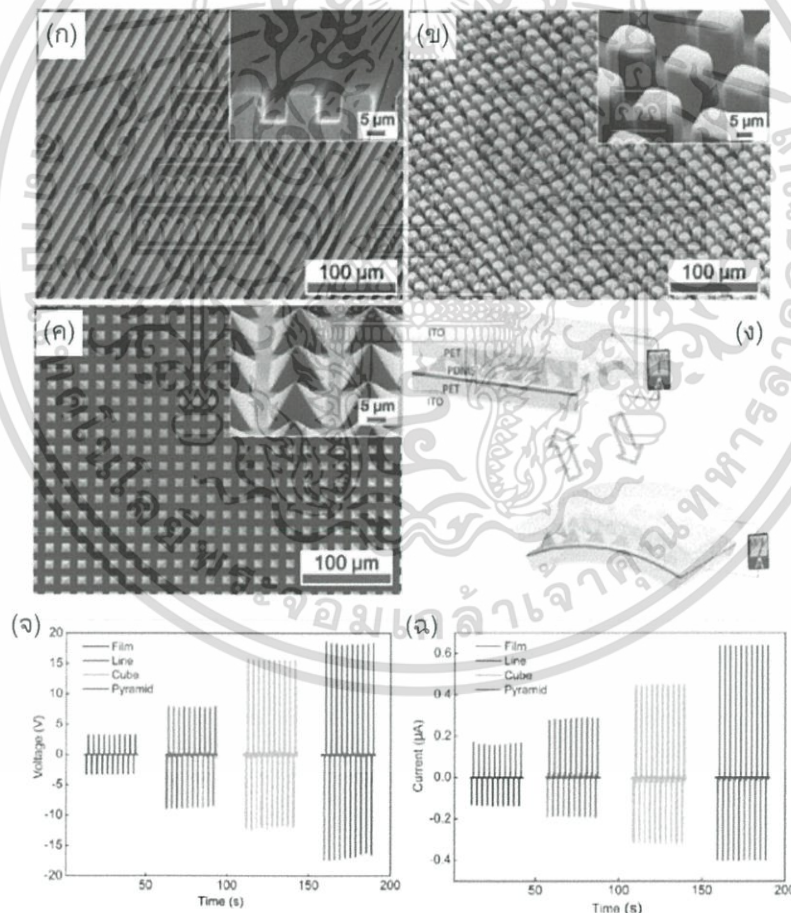
รูปที่ 2.49 ความขรุขระบนพื้นผิว PDMS ที่มีลวดลายเป็น (ก) เส้น (ข) ลูกบาศก์ และ (ค) พีรามิด ส่วน (ง) โครงสร้างของอุปกรณ์ FTEH ผลทางไฟฟ้าขาออก (จ) แรงดัน และ (ฉ) กระแสไฟฟ้า ของ FTEH ที่ผลิตได้ (ปรับแต่งจาก [25])
