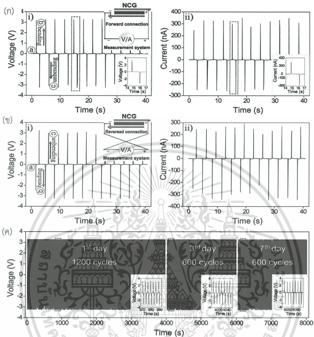
รูปที่ 2.39 (ก) ค่าตรวจวัดการส่งออกของศักย์ไฟฟ้าและกระแสไฟฟ้าของอุปกรณ์ตัวกำเนิดนาโนคอมโพสิตในการเชื่อมต่อไปข้างหน้า ในช่วงที่มีการดัด และไม่มีดัด และ (ข) ในการเชื่อมต่อแบบย้อนกลับ (ค) แสดงระยะเวลาในการทดสอบความทนทานต่อการนำไฟฟ้าเพื่อยืนยันเสถียรภาพของอุปกรณ์ตัวกำเนิดนาโนคอมโพสิต [20]
