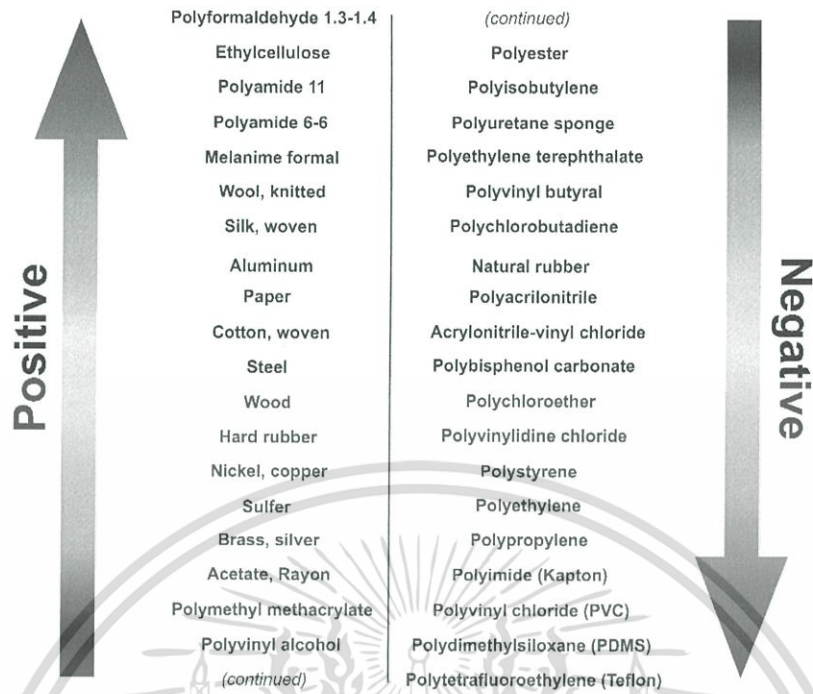
รูปที่ 2.25 แผนภาพแสดงวัสดุโพรไบโอเล็กทริกที่มีแนวโน้มให้อิเล็กตรอน (ประจุบวก) และรับอิเล็กตรอน (ประจุลบ) [13]
