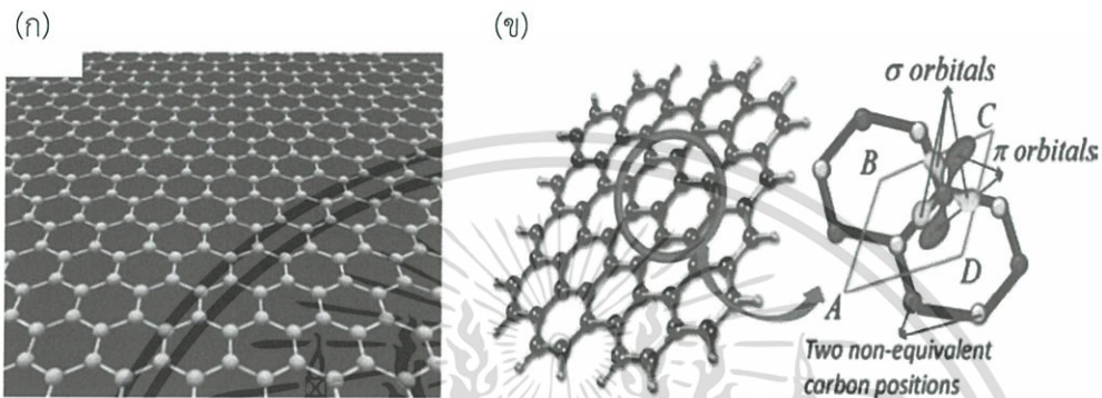
รูปที่ 2.14 (ก) โครงสร้างตาข่ายของแผ่นแกรฟีน (ข) โครงสร้างออร์บิทัลของแผ่นแกรฟีน [5]
