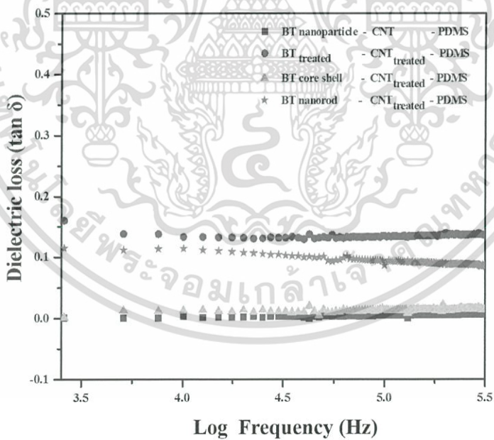
รูปที่ 4.18 ความสัมพันธ์ระหว่างค่าการสูญเสียไดโอเล็กทริกกับค่าความถี่ของวัสดุผสม BT - CNT - PDMS วัสดุผสม BT treated -CNT treated -PDMS วัสดุผสม BT nanorod -CNT treated -PDMS และวัสดุผสม BT coreshell -CNT treated -PDMS
