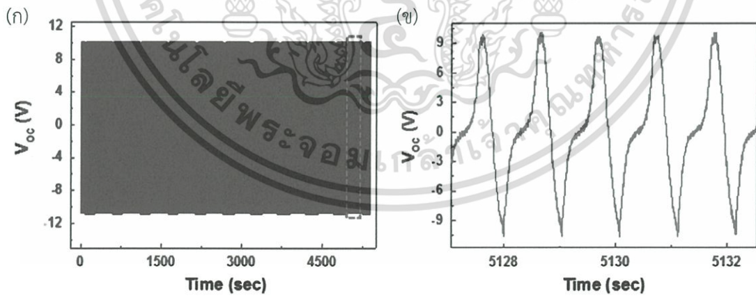
รูปที่ 2.36 (ก) V_{oc} ที่ส่งออกจาก 40 wt% ตัวกำเนิดเพียโซอิเล็กทริกนาโนคอมโพสิตระหว่างการทดสอบความเสถียรโดยการติดตามมากกว่า 5000 รอบ (ข) ขยายสัญญาณที่ส่งออกในรูปบริเวณที่ไฮไลต์ของ (ก) [19]
