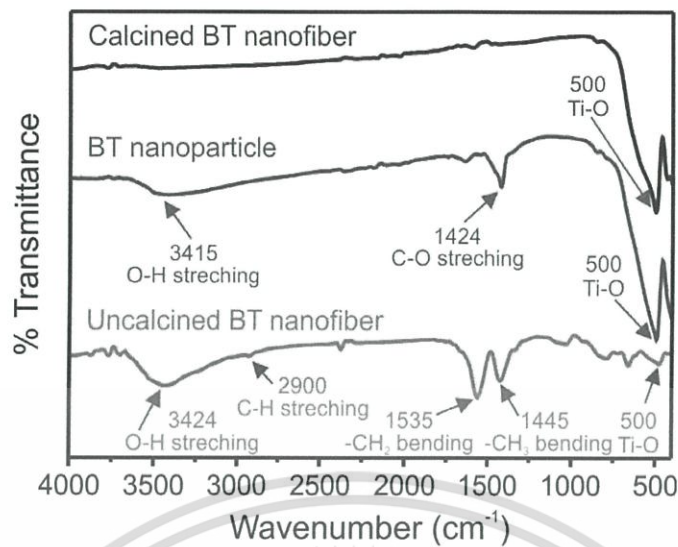
รูปที่ 4.30 ผลการตรวจสอบเอกลักษณ์ของเส้นใยนาโน BT อนุภาคนาโน BT เกรดการค้า และเส้นใยนาโน BT หลังเผา ด้วยเทคนิค FT-IR
