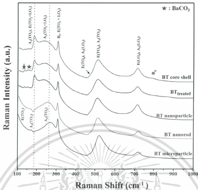
รูปที่ 4.6 รูปแบบรามานสเปกตรัมของอนุภาคนาโน BT อนุภาคนาโน BT ที่ผ่านการปรับปรุงพื้นผิว แท่งนาโน BT และอนุภาคคอร์เชล BT
