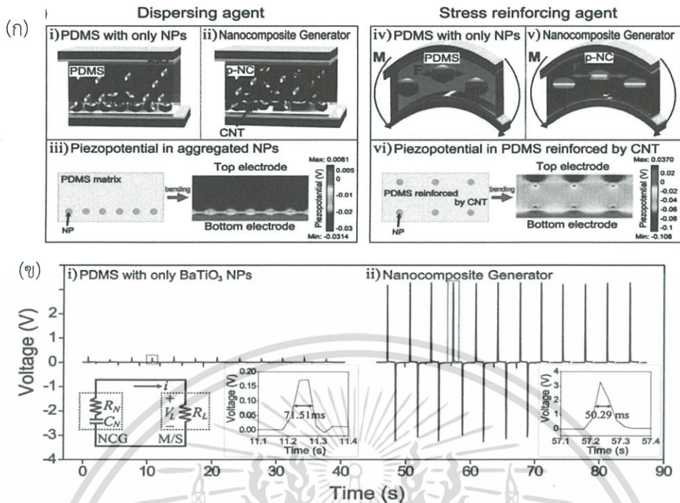
รูปที่ 2.41 (ก) (i) โครงสร้างแบบตัดขวางของอุปกรณ์ตัวกำเนิดนาโนคอมโพสิตและการคำนวณการกระจายศักย์เพื่อโซ่อิเล็กทริกสำหรับอธิบายบทบาทของ CNTs โดยทำหน้าที่กระจายตัว (ii) และตัวเร่งความเร็ว ซึ่งได้รับการรองรับโดยถูกคำนวณจากความแตกต่างของศักย์เพื่อโซ่อิเล็กทริก (iii และ vi) (ข) การส่งออกศักย์ไฟฟ้าที่สร้างขึ้นจากอุปกรณ์ที่มีเพียงอนุภาคนาโน BT และอุปกรณ์ตัวกำเนิดนาโนคอมโพสิต อนุภาคนาโนที่มีการกระจายตัวที่ดีและเพิ่มประสิทธิภาพของความเครียดโดย CNTs ทำให้มีศักย์ไฟฟ้าส่งออกที่สูง รูปด้านล่างขวาแสดงศักย์ที่ส่งออก สร้างโดยการเคลื่อนไหวทางกลโดยการดัด รูปประกอบด้านล่างซ้ายแสดงวงจรมูลของอุปกรณ์ ตัวกำเนิดนาโนคอมโพสิต [20]
