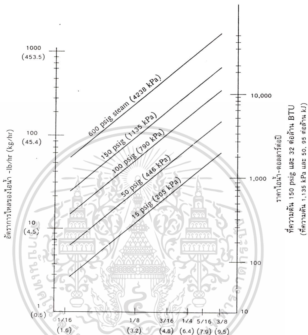
รูปที่ 2.8 ราคาไอน้ำที่รั่วสู่บรรยากาศผ่านรูขนาดต่างๆ
