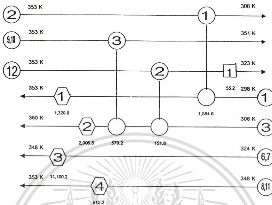
รูปที่ 2.11 แสดงเครือข่ายการเชื่อมโยงของอุปกรณ์แลกเปลี่ยนความร้อน โดยใช้ค่า \Delta T_{\min} เท่ากับ 25 K ซึ่งรูปสี่เหลี่ยมหมายถึงหน่วยที่ต้องการใช้น้ำเย็น รูปหกเหลี่ยมหมายถึงหน่วยที่ต้องการใช้ความร้อนจากภายนอก รูปวงกลมซึ่งเชื่อมระหว่างสายร้อนและเย็นแสดงการจับคู่เพื่อแลกเปลี่ยนความร้อน
