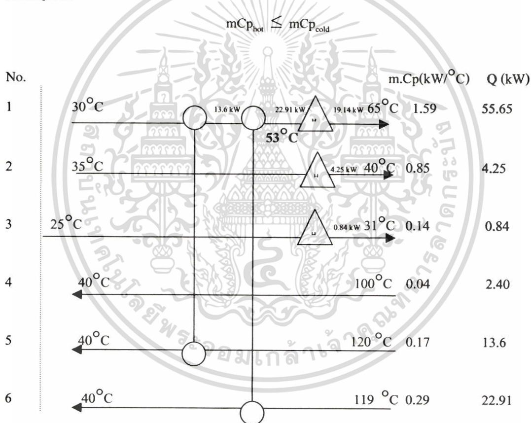
รูปที่ ง.2 การออกแบบเครือข่ายการเชื่อมโยงของอุปกรณ์แลกเปลี่ยนความร้อน
