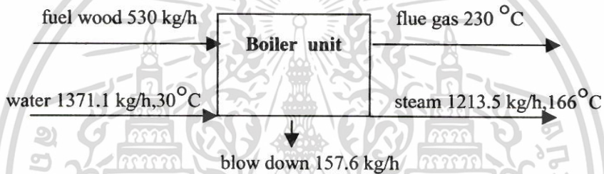
รูปที่ ก.1 แสดงสมดุลมวลส่วนหม้อไอน้ำ
