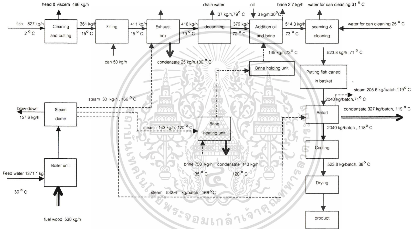
รูปที่ 3.1 แผนภาพแสดงขั้นตอนการผลิตปลาในน้ำเกลือบรรจุกระป๋อง
