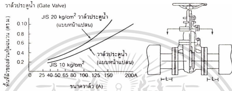
(ก) พื้นที่หุ้มฉนวนของวาล์ว
