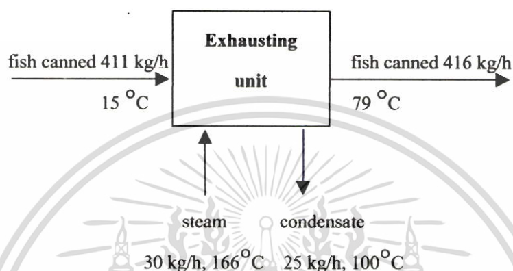
รูปที่ ก.2 แสดงสมดุลมวลของส่วนการนึ่ง
