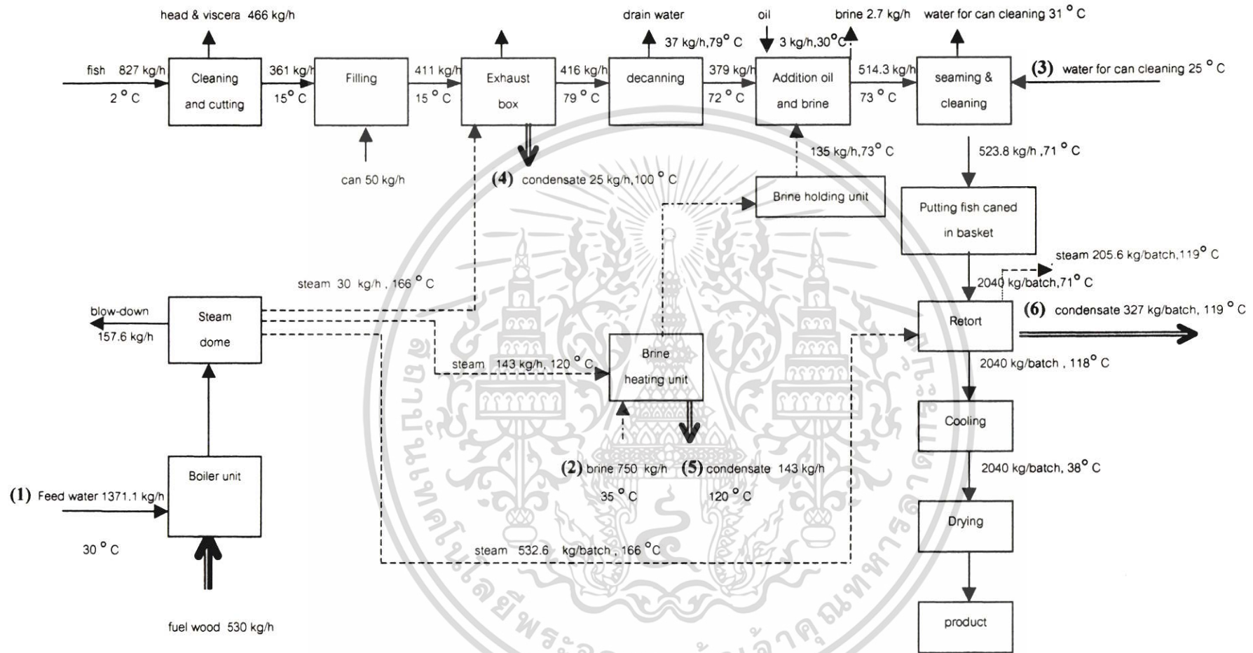
รูปที่ 4.1 แสดงสายร้อนและสายเย็นในกระบวนการผลิตปลาในน้ำเกลือบรรจุกระป๋อง
