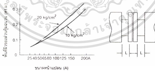
(ข) พื้นที่หุ้มฉนวนของหน้าแปลน
