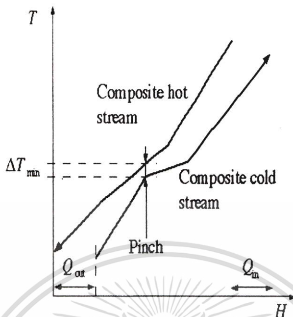
รูปที่ 2.9 Composite curves
