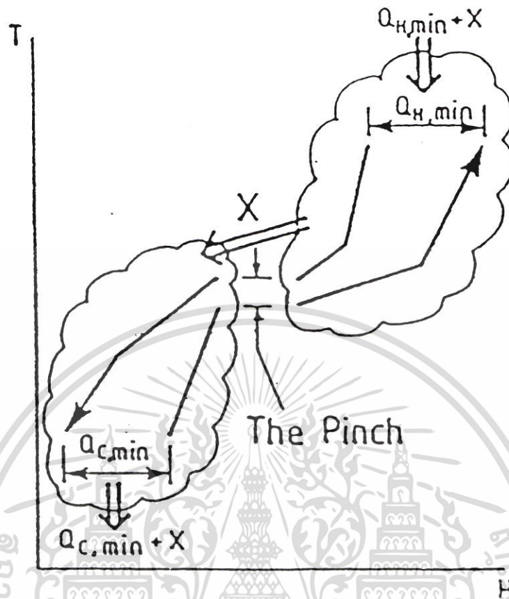
รูปที่ 2.10 แสดงหลักการของพินช์เทคโนโลยี
