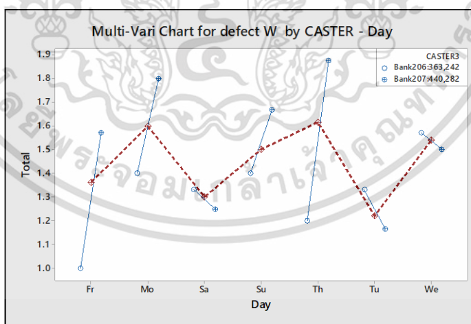
รูปที่ 5.6 Muti-Vari แสดงความสัมพันธ์ระหว่างวันเวลาในการทำงานกับพนักงานหล่อสุขภัณฑ์
