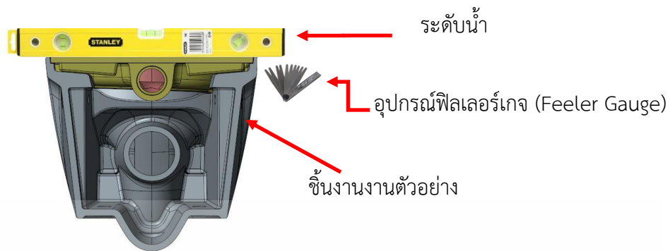
รูปที่ 5.5 แสดงตำแหน่งการวัดความบิดเบี้ยวของสุขภัณฑ์ตัวอย่าง
