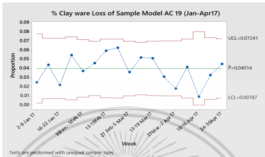
รูปที่ 3.6 กราฟแสดง % Clay Loss ของสุขภรณ์ตัวอย่างรุ่น AC19
