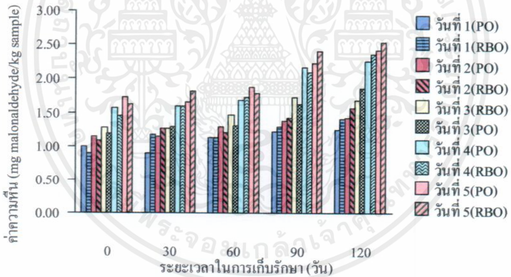
ภาพที่ 4.14 ค่า TBA ของผลิตภัณฑ์มันฝรั่งทอดที่ผ่านการทอดเป็นระยะเวลา 5 วัน ที่อุณหภูมิ 190 องศาเซลเซียส ในน้ำมันปาล์ม (PO) และน้ำมันรำข้าว (RBO)
