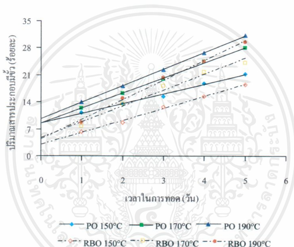
ภาพที่ 4.2 ปริมาณสารประกอบมีขั้วของน้ำมันปาล์ม (PO) และน้ำมันรำข้าว (RBO) จากการทอดมันฝรั่งชิ้นบางที่อุณหภูมิ 150 170 และ 190 องศาเซลเซียส
