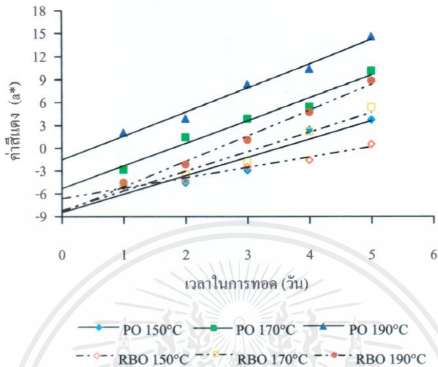
ภาพที่ 4.7 ค่าสีแดง (a*) ของน้ำมันปาล์ม (PO) และน้ำมันรำข้าว (RBO) จากการทอดมันฝรั่งขึ้นบางที่อุณหภูมิ 150 170 และ 190 องศาเซลเซียส
