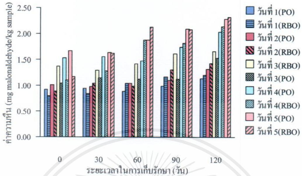
ภาพที่ 4.13 ค่า TBA ของผลิตภัณฑ์มันฝรั่งทอดที่ผ่านการทอดเป็นระยะเวลา 5 วัน ที่อุณหภูมิ 170 องศาเซลเซียส ในน้ำมันปาล์ม (PO) และน้ำมันรำข้าว (RBO)
