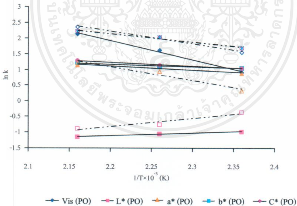
ภาพที่ 4.10 ความสัมพันธ์ของอุณหภูมิต่ออัตราการเกิดปฏิกิริยาของคุณภาพทางเคมีในน้ำมันปาล์ม (PO) และน้ำมันรำข้าว (RBO)
