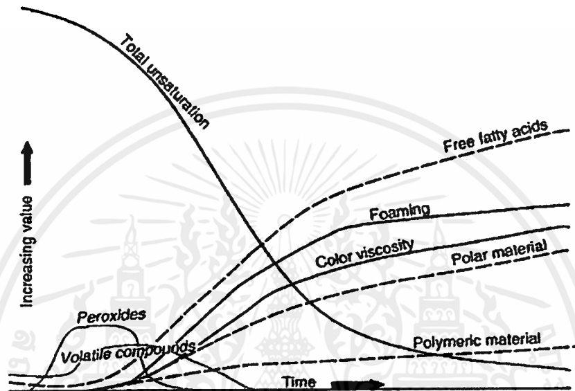
ภาพที่ 2.1 การเปลี่ยนแปลงทางเคมีระหว่างการทอดแบบน้ำมันท่วม
