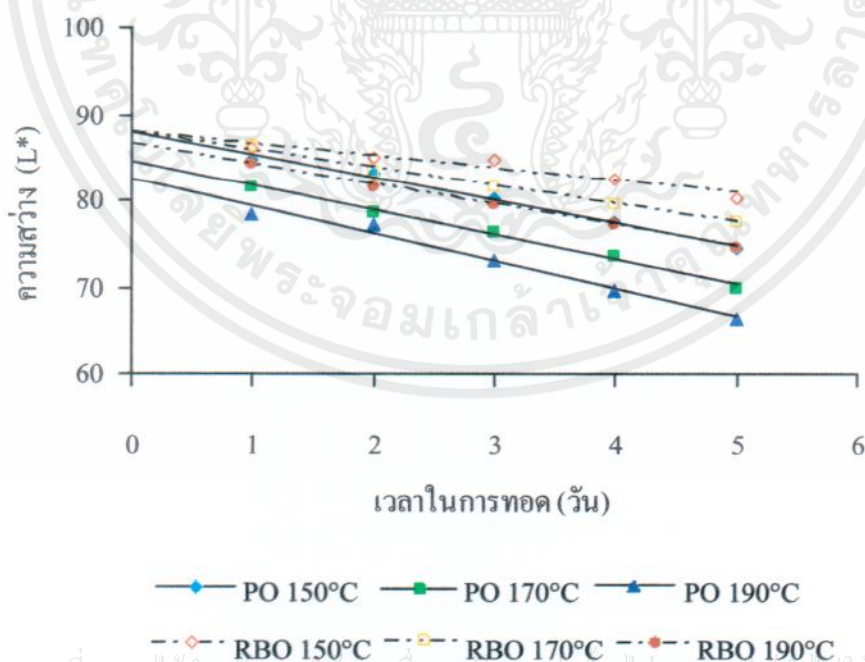
ภาพที่ 4.6 ค่าความสว่าง ( L^* ) ของน้ำมันปาล์ม (PO) และน้ำมันรำข้าว (RBO) จากการทอดมันฝรั่งขึ้น บ่างที่อุณหภูมิ 150 170 และ 190 องศาเซลเซียส
