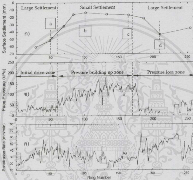
รูปที่ 3.3.1 กราฟแสดงค่าการทรุดตัวของผิวดิน ความดันหน้าหัวเจาะ และความเร็วขุดเจาะ โดยบันทึกระหว่างสถานีศูนย์วัฒนธรรมฯ และสถานีประชาราษฎร์บำเพ็ญ
