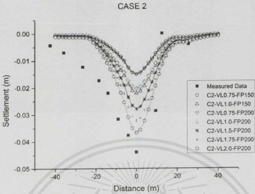
รูปที่ 5.2.2 กราฟแสดงการเปรียบเทียบผลการวิเคราะห์ห้กับค่าการทรุดตัวของดินที่กจากสนาม
