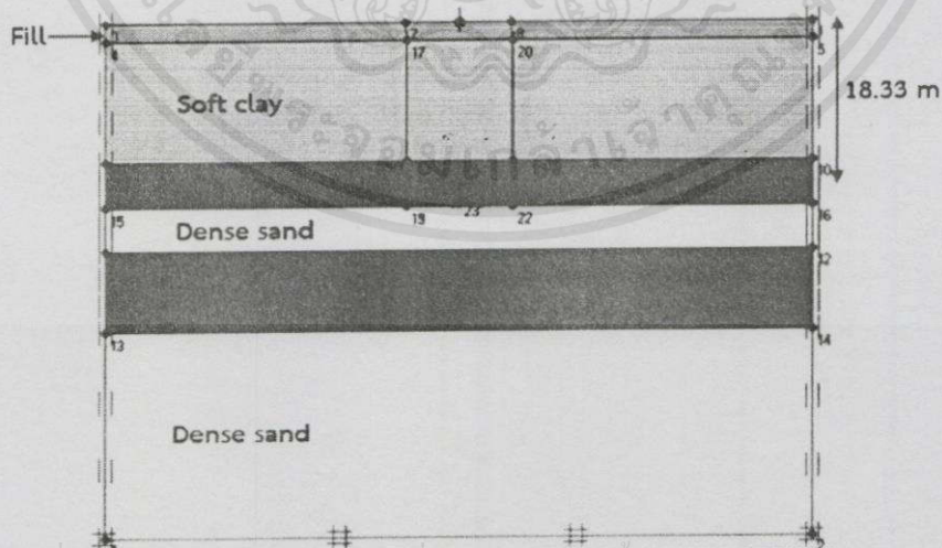
รูปที่ 4.4.2.1 แบบจำลองชั้นดินและการวางตำแหน่งอุโมงค์กรณี 1
