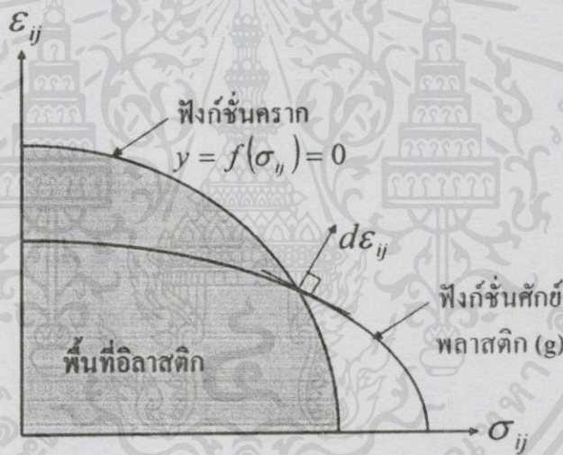
รูปที่ 3.4.8 ภาพจำลองหลักการคำนวณความเครียดพลาสติก
