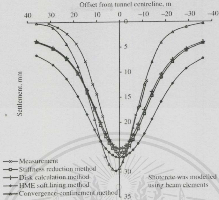
รูปที่ 2.27 ค่าการทรุดตัวจากวิธีการวิเคราะห์ต่างๆของการใช้ชิ้นส่วนแบบคานในแบบจำลองผนังอุโมงค์ Shotcrete (M.Karakus, 2007)
