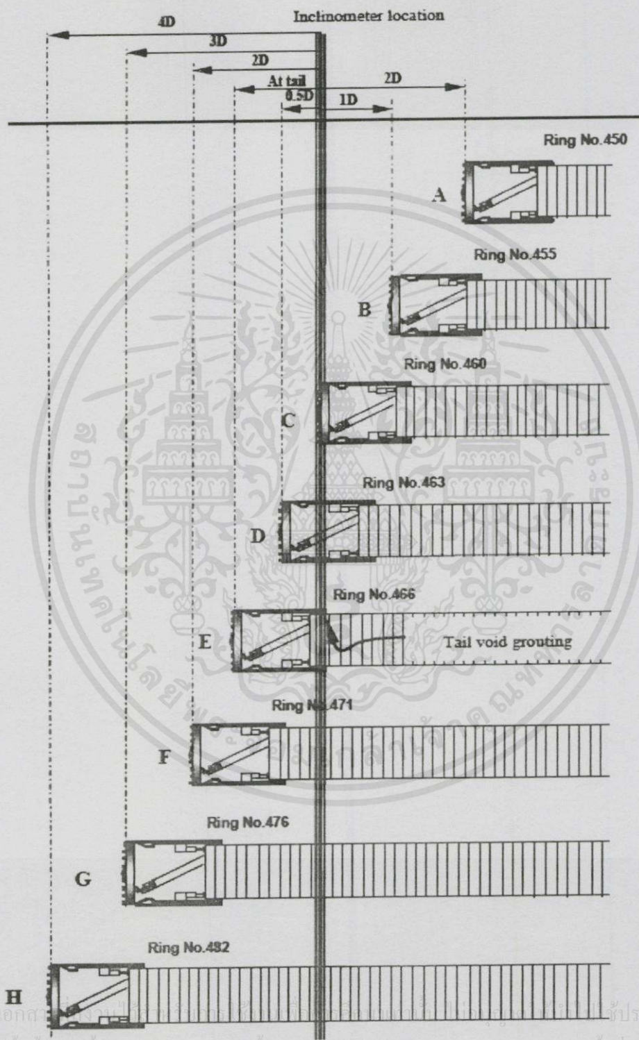
รูปที่ 3.3.18 ตำแหน่งของหัวเจาะอุโมงค์ขณะเคลื่อนที่ผ่านเครื่องมือวัดการเคลื่อนตัวทางด้านข้าง
