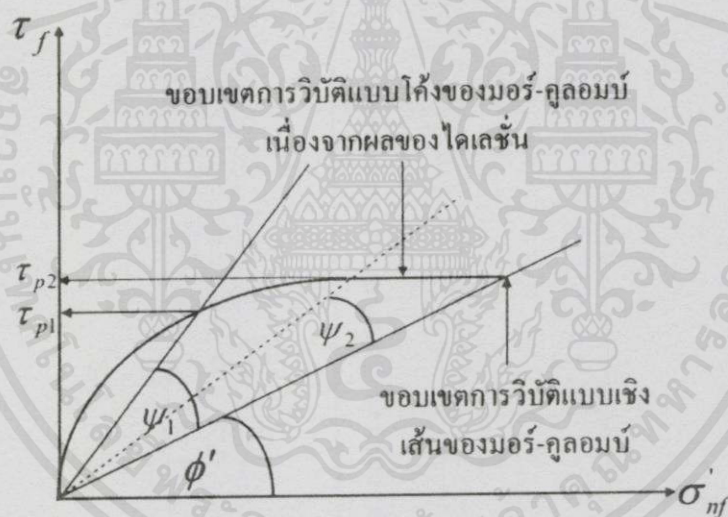
รูปที่ 3.4.10 ผลของมุมไคเลชันต่อพื้นผิวครากแบบมอร์-กูลอมบ์
