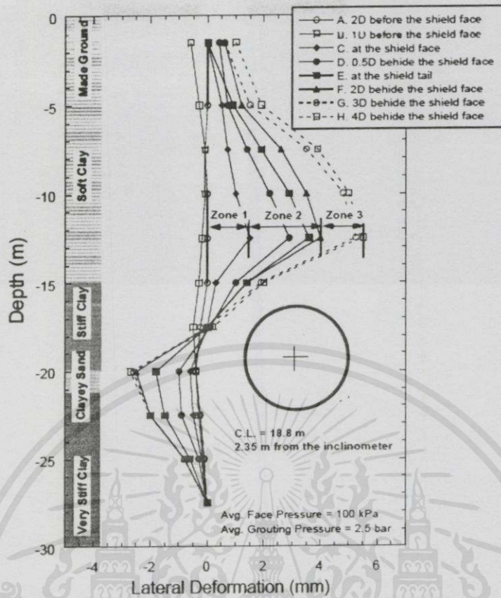
รูปที่ 3.3.17 การเคลื่อนตัวของทางด้านข้างของดินที่ตำแหน่ง IN-T7-04
