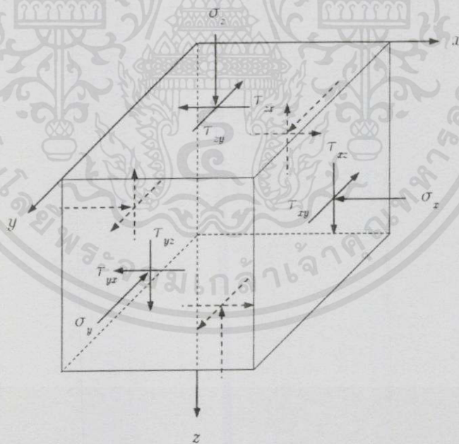
รูปที่ 3.4.1 ส่วนประกอบของความเค้น (Stress components) 3 มิติ
