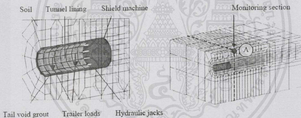
รูปที่ 2.7 แบบจำลองไฟไนต์อีลิเมนต์แบบ 3 มิติและหน้าตัดที่ทำการพิจารณา
