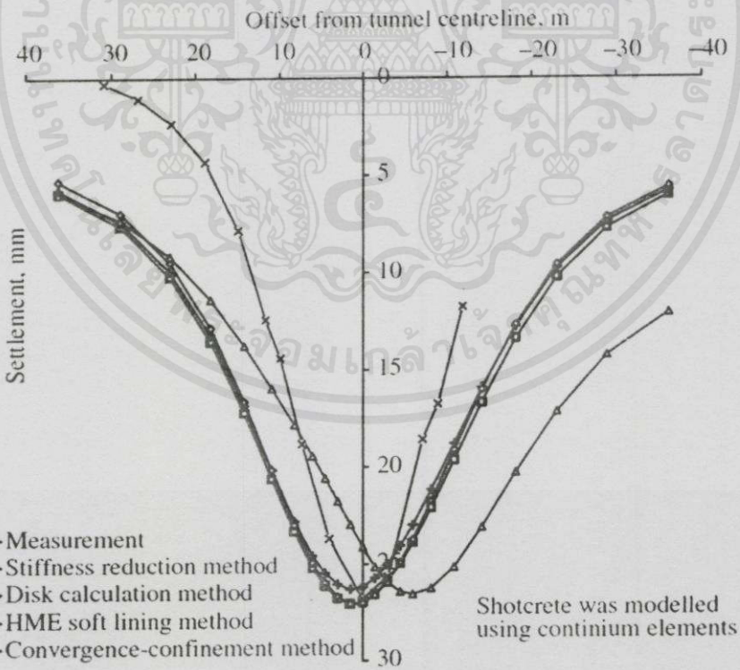
เอกสารนี้เป็นเอกสารที่สงวนไว้สำหรับการใช้งานเพื่อการศึกษาเท่านั้น ไม่อนุญาตให้นำไปใช้ประโยชน์ด้านการค้า ไม่ว่ารูปที่ 2.28 ค่าการทรุดตัวจากวิธีการวิเคราะห์ต่างๆของการใช้ชิ้นส่วนแบบต่อเนื่องในแบบจำลองผนังอุโมงค์ Shotcrete (M.Karakus, 2007)
