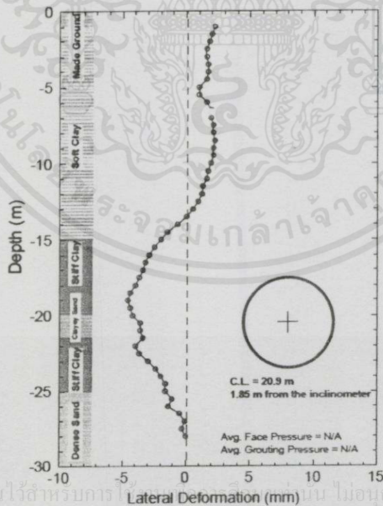
รูปที่ 3.3.16 การเคลื่อนตัวทางด้านข้างของดินที่ตำแหน่ง IN-T7-03 รังที่มีการนำไปใช้
