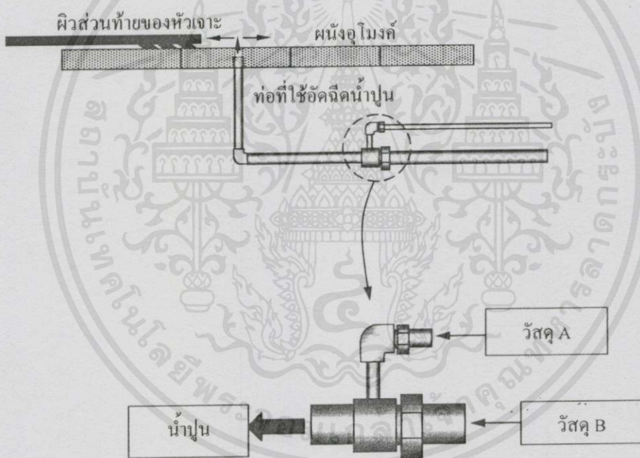
รูปที่ 3.1.19 การอัดฉีดน้ำปูนโดยการผสมวัสดุ A และ B เข้าด้วยกัน
