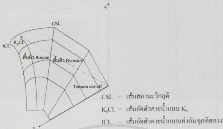
รูปที่ 3.4.12 ขอบเขตการวิบัติ (State boundary surface, SBS)
