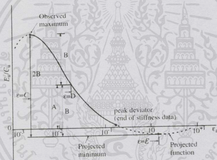
รูปที่ 2.17 Curve fitting ของข้อมูลสตรีเฟนเสสของความเครียด (Jardine et al., 1986)
