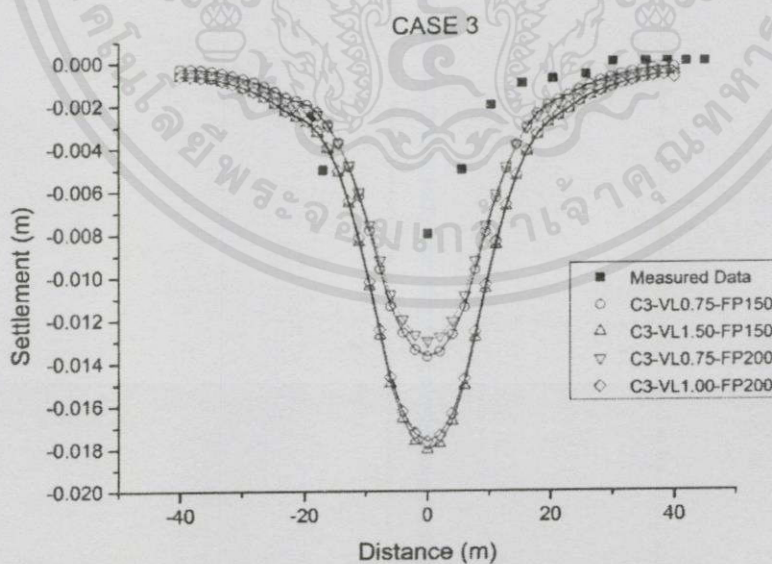
รูปที่ 5.2.8 กราฟแสดงการเปรียบเทียบผลการวิเคราะห์ห้กับค่าการทรุดตัวที่บันทึกจากสนาม
