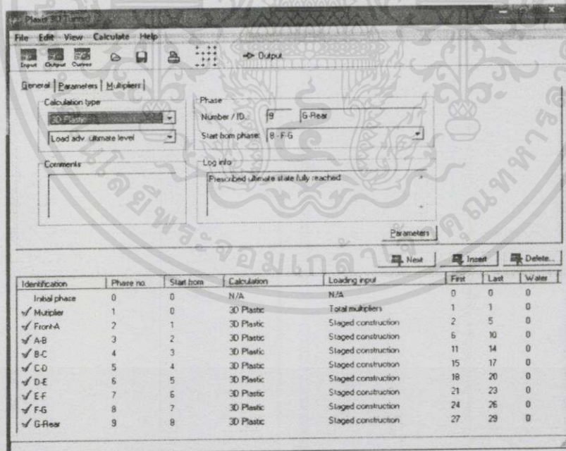
รูปที่ 4.4.1.7 แสดง phase การขุดเจาะอุโมงค์
