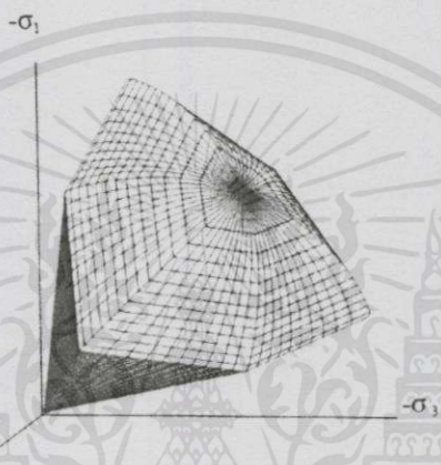
รูปที่ 3.4.13 ความสัมพันธ์ของแบบจำลองชนิด Hardening Soil
