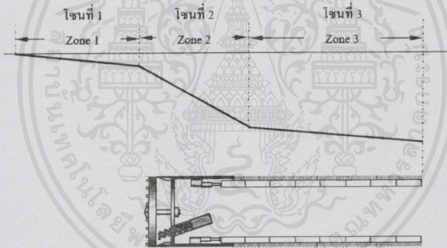
รูปที่ 3.3.12 แผนภาพแสดงรูปตัดการทรุดตัวผิวดินตามแนวยาวที่เกิดจากการก่อสร้างอุโมงค์
