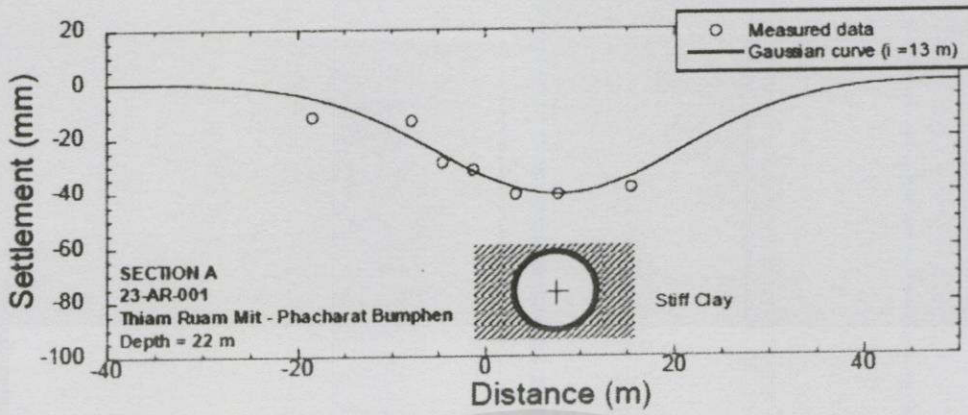
รูปที่ 5.2.1 กราฟแสดงการทรุดตัวที่ผิวดินที่บันทึกจากสนาม
