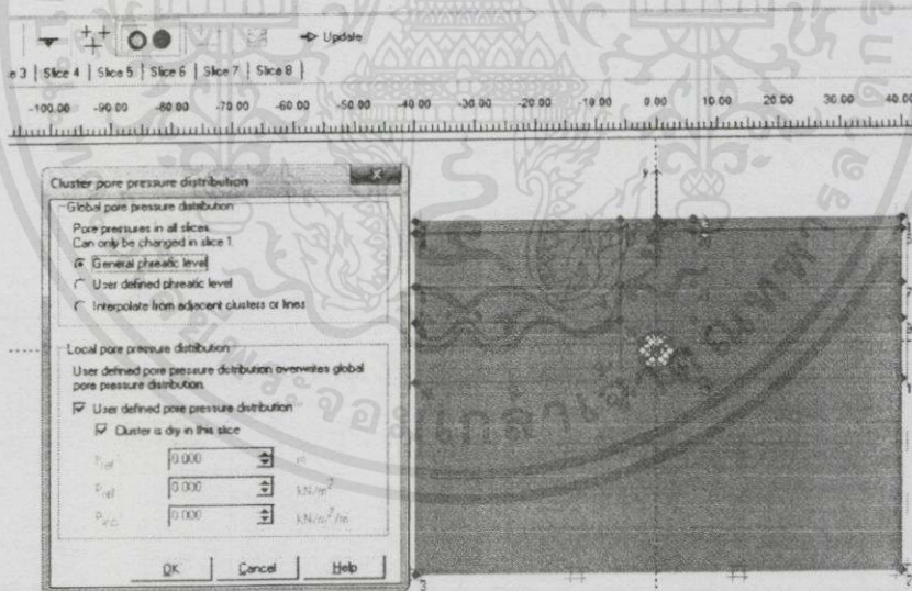
รูปที่ 4.4.2.7 แสดงการกำหนด Cluster pore pressure distribution
