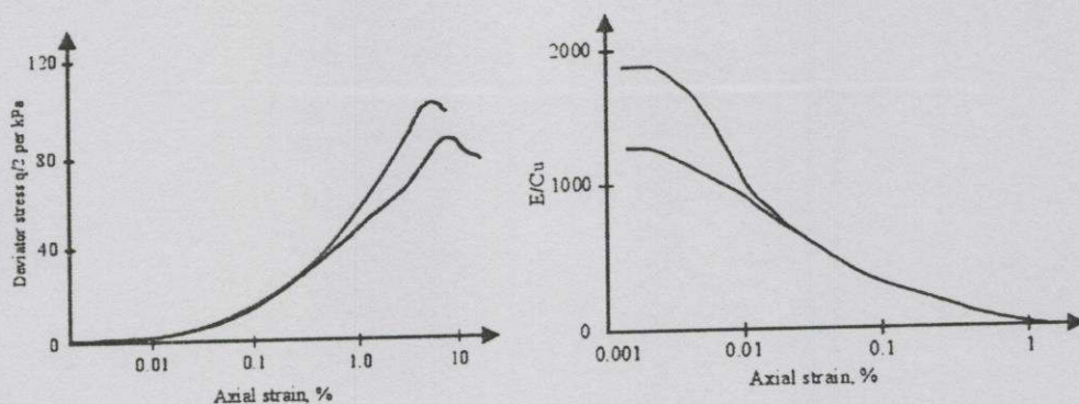
รูปที่ 2.18 ข้อมูลค่าสติเฟนสที่สภาวะความเครียดต่ำของดิน London clay (Jardine et al., 1984)
