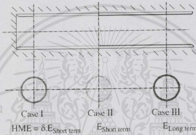
รูปที่ 2.14 พื้นฐานทฤษฎีของวิธี Hypothetical modulus of elasticity soft lining (HME) (Karakus and Fowell, 2003)
