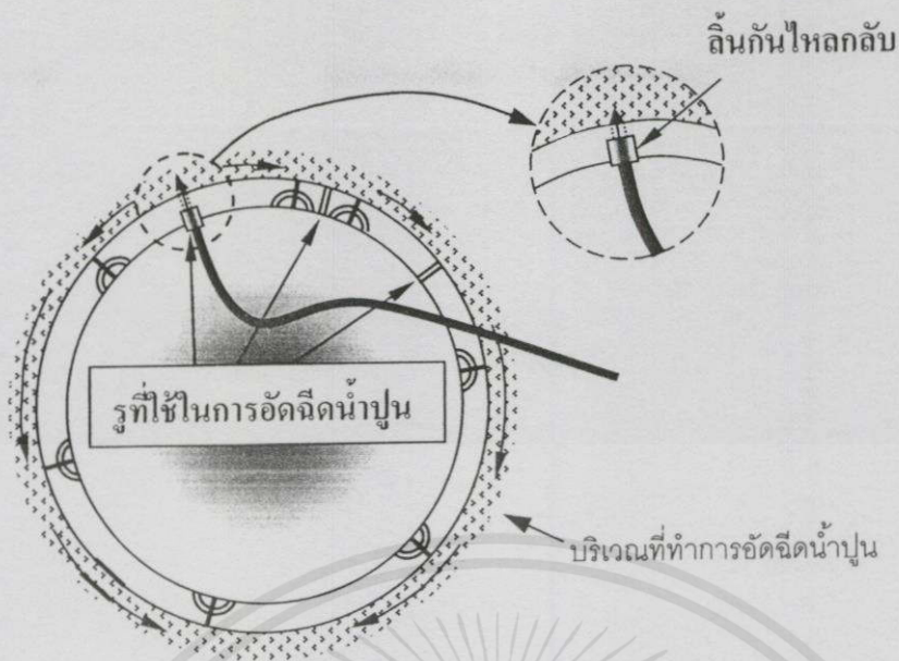
รูปที่ 3.1.18 การอัดฉนวนน้ำปูนผ่านรูภายในชั้นส่วนประกอบผนังอุโมงค์
