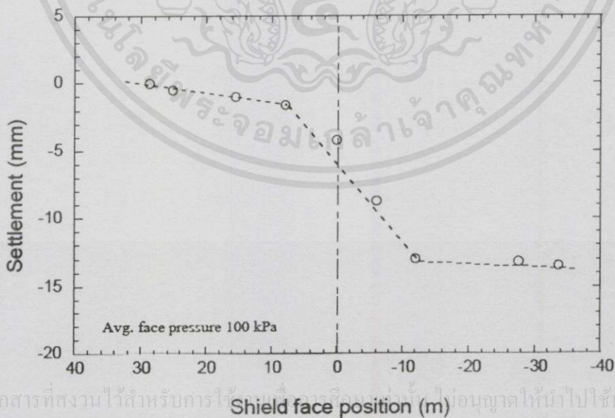
รูปที่ 3.3.10 การทรุดตัวตามแนวยาวของดินวัด ณ ตำแหน่ง b (ผนังอุโมงค์วงที่ 101)
