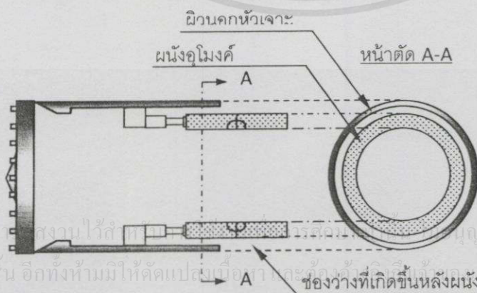
รูปที่ 3.1.11 ช่องว่างที่เกิดขึ้นระหว่างผนังอุโมงค์และหัวเจาะ
