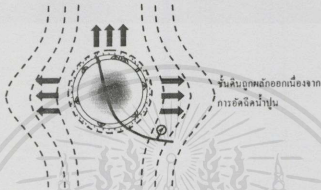
รูปที่ 3.2.20 อิทธิพลจากการอัดดินน้ำปูนที่ส่งผลกระทบต่อ การเคลื่อนตัวทางด้านข้างของดิน
