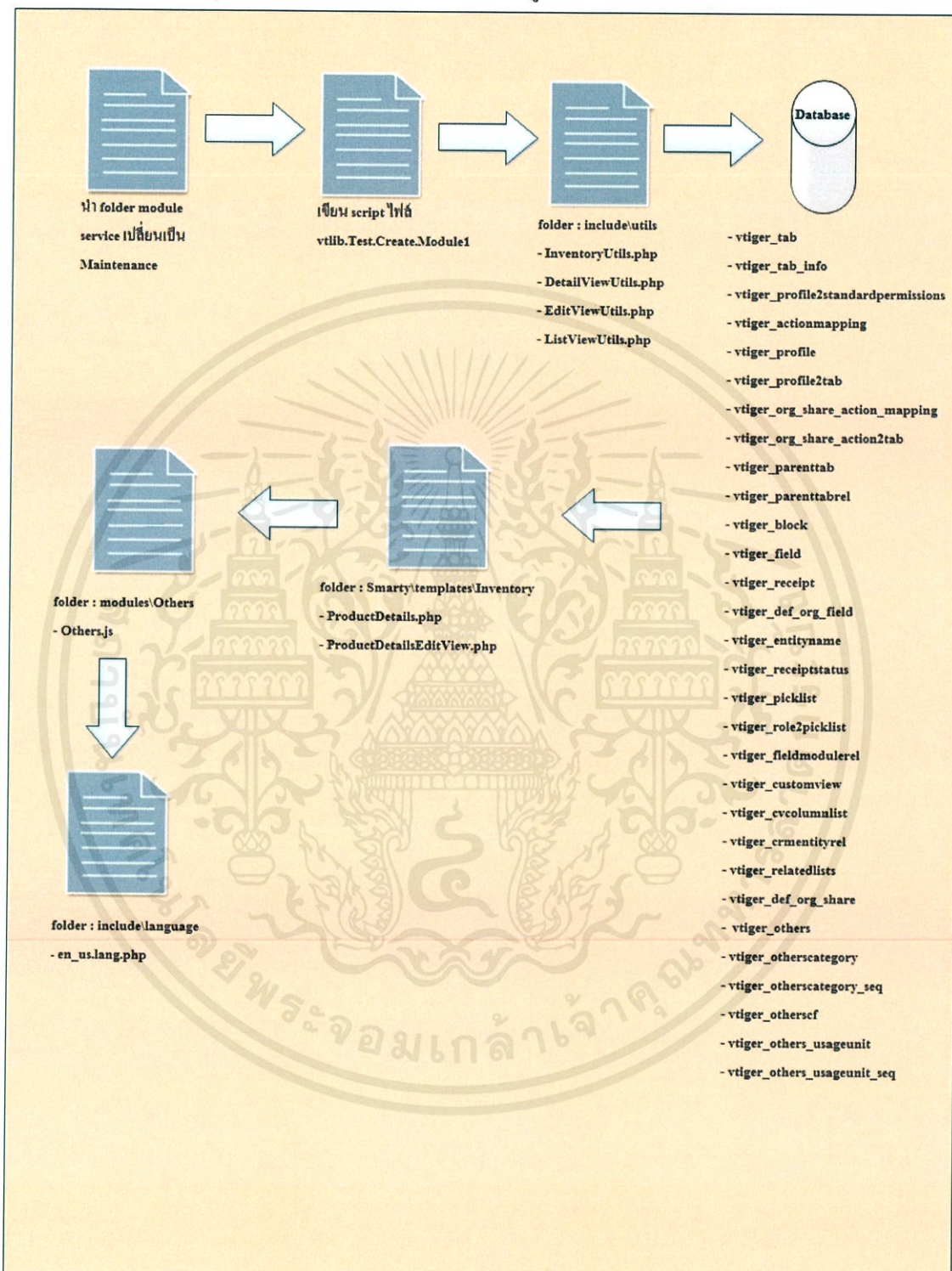
รูปที่ 4.30 ไฟล์ที่เกี่ยวข้องในการสร้างโมดูล Others
