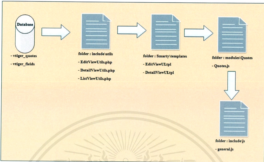
รูปที่ 4.10 ไฟล์ที่เกี่ยวข้องในการปรับปรุงการอ้างอิงใบเสนอราคา
