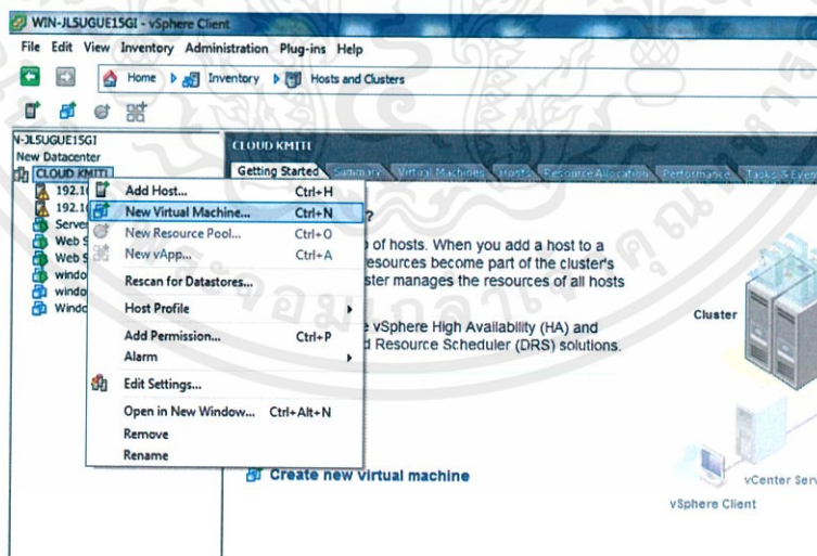
รูปที่ 4.61 หน้าจอการสร้างเครื่องเสมือน
