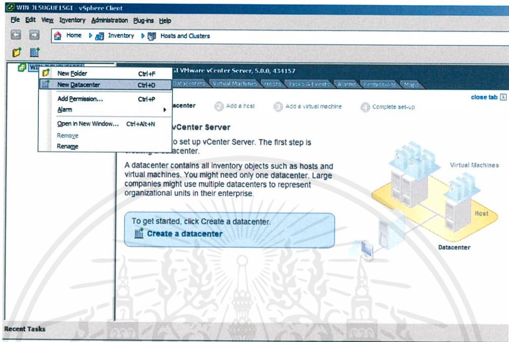
รูปที่ 3.3 การสร้าง Data Center ขั้นตอนที่ 1
