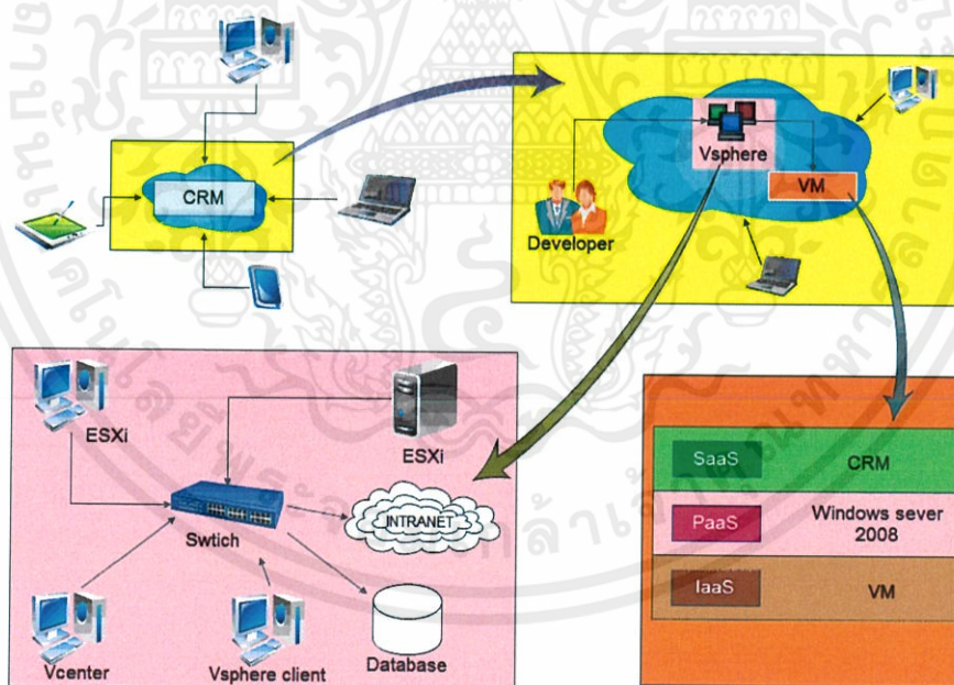
รูปที่ 3.22 สถาปัตยกรรมโดยรวมของ vTiger บนการประมวลผลแบบกลุ่มเมฆ
