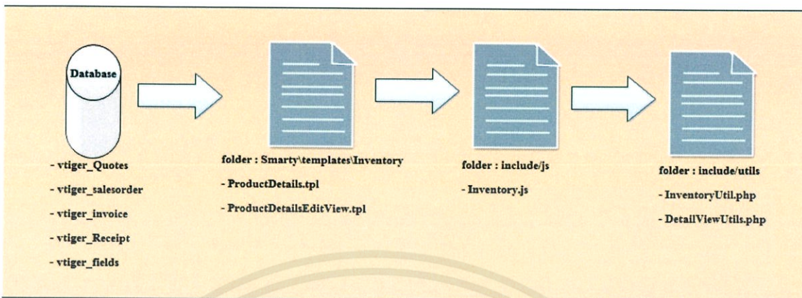
รูปที่ 4.43 ไฟล์ที่เกี่ยวข้องในการเพิ่มช่องตัวอักษรกำกับยอดเงินสุทธิ
