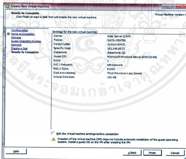
รูปที่ 4.69 หน้าจอการ Edit the virtual machine settings before completion
