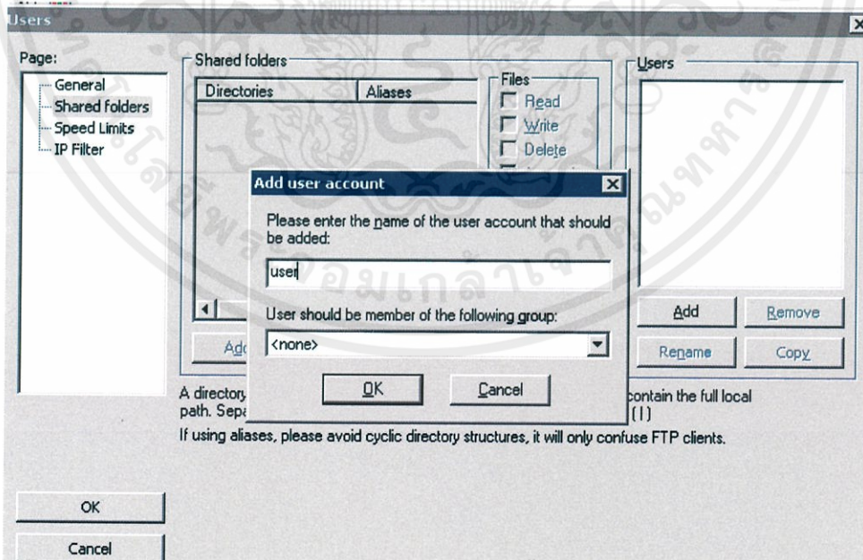
รูปที่ ๑.12 การตั้งค่า FileZilla Server ขั้นตอนที่ 1
