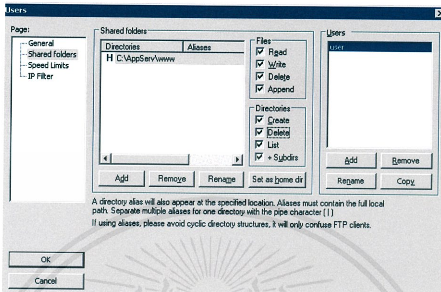
รูปที่ ๑.15 การตั้งค่า FileZilla Server ขั้นตอนที่ 4
