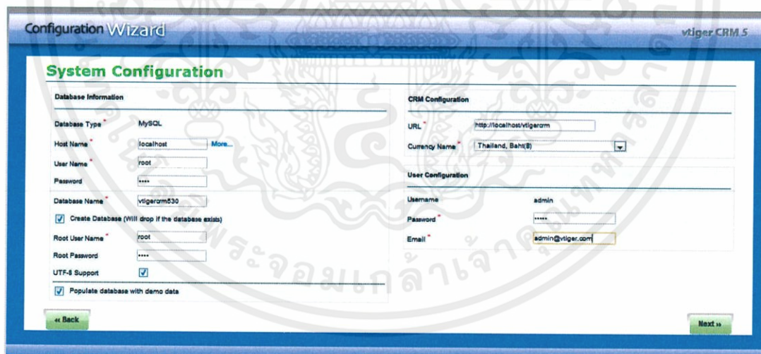
รูปที่ ข.4 หน้าจอในการกำหนดค่าต่างๆ ของระบบ
