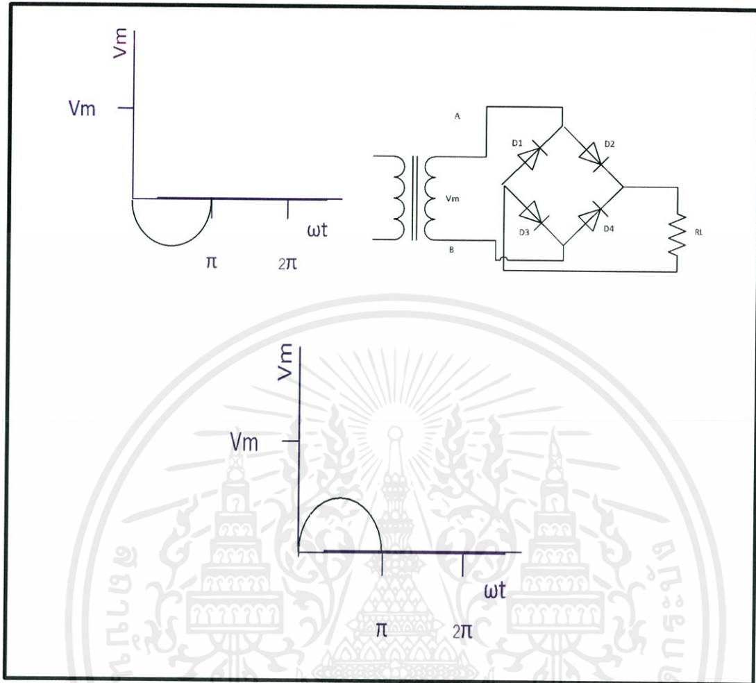
รูปที่ 2.22 (ก) การทำงานของวงจรเรียงกระแสเต็มคลื่นแบบบริดจ์เมื่ออินพุตเป็นซิกลอบ
