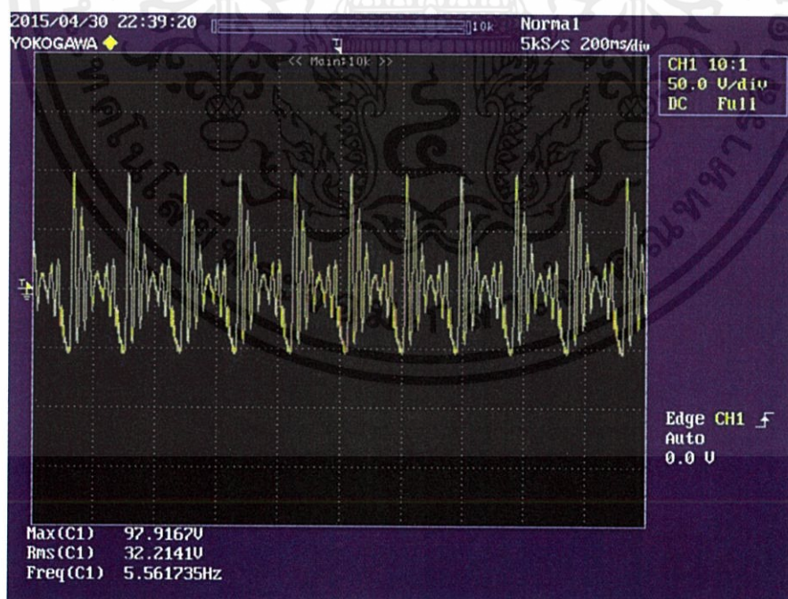
เอกสารนี้เป็นเอกสารที่สงวนไว้สำหรับการใช้งานเพื่อการศึกษาเท่านั้น ไม่อนุญาตให้นำไปใช้ประโยชน์ด้านการค้า ไม่ว่ากรณีใดๆ รูปที่ 4.7 รูปคลื่นสัญญาณแรงดันจากแผ่นเพียโซอิเล็กทริก 2 แผ่นต่ออนุกรมความถี่ 5 Hz
