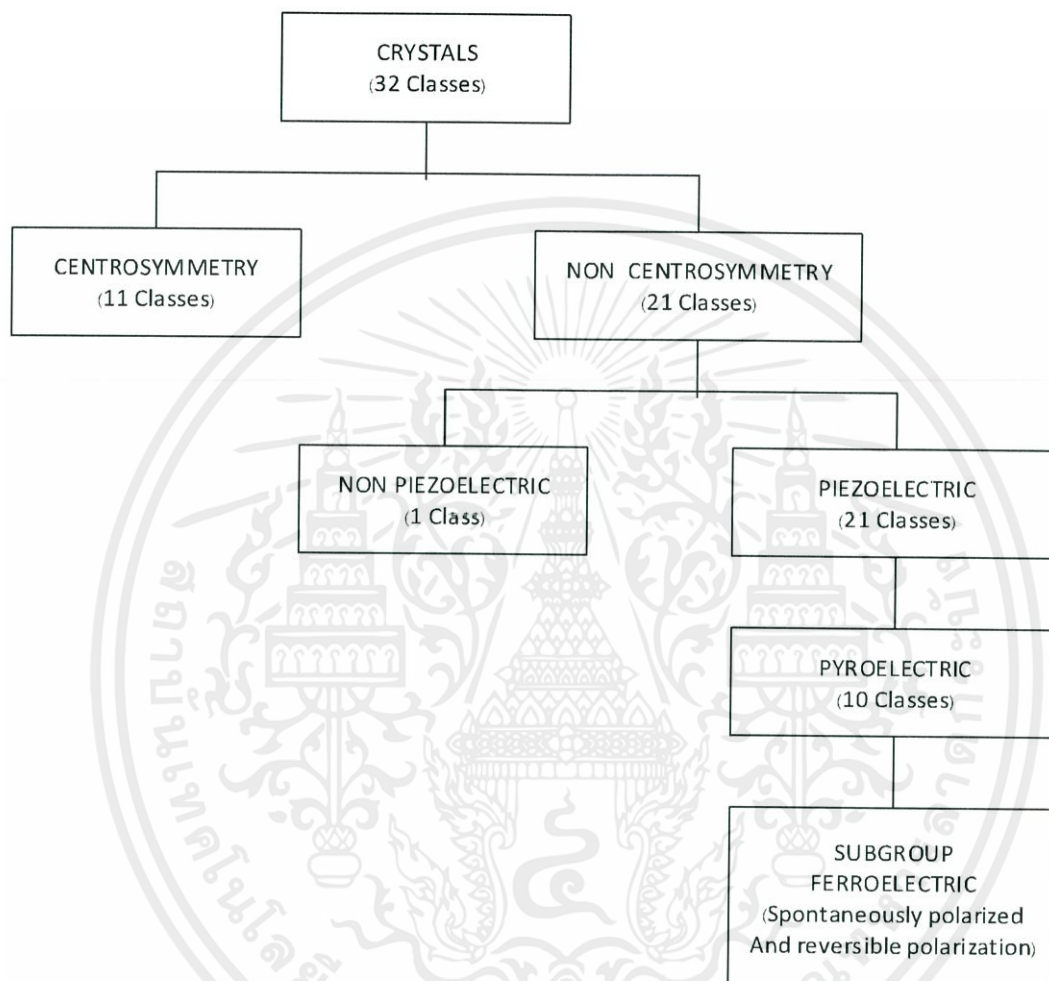
รูปที่ 2.1 ความสัมพันธ์ของการแบ่งโครงสร้างของผลึก
