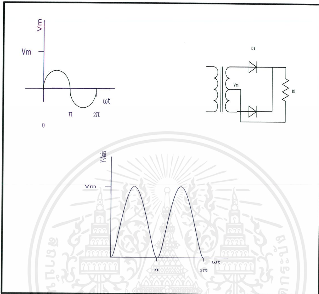
รูปที่ 2.20 (ข) การทำงานของวงจรเรียงกระแสแบบเซนเตอร์แทปเมื่ออินพุตเป็นซีกลบ
