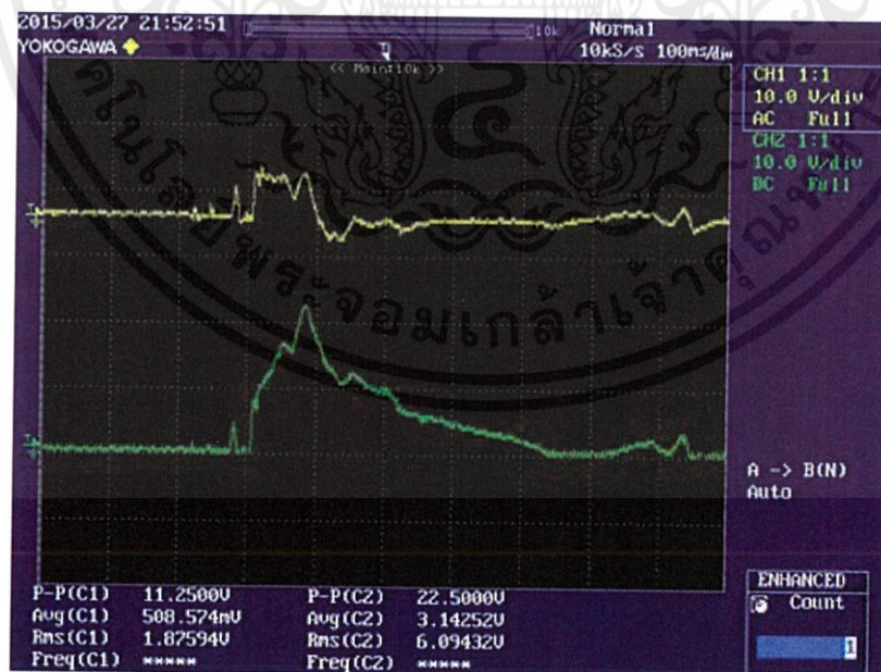
รูปที่ 4.37 รูปคลื่นสัญญาณแรงดันจากการเดินเทียบแผ่นเพียโซอิเล็กทริกจำนวน 4 แผ่น ต่อกันแบบคู่อนุกรมกันแล้วนำมาขนานกัน
