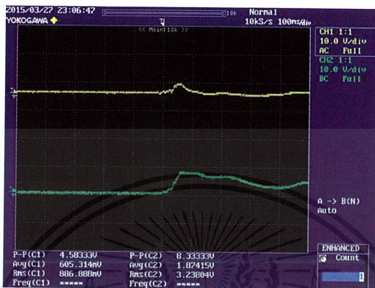
รูปที่ 4.42 รูปคลื่นสัญญาณแรงดันจากการเดินเหียบแผ่นเพียโซอิเล็กทริกจำนวน 4 แผ่น ต่อกัน แบบวงจรถนนาน
