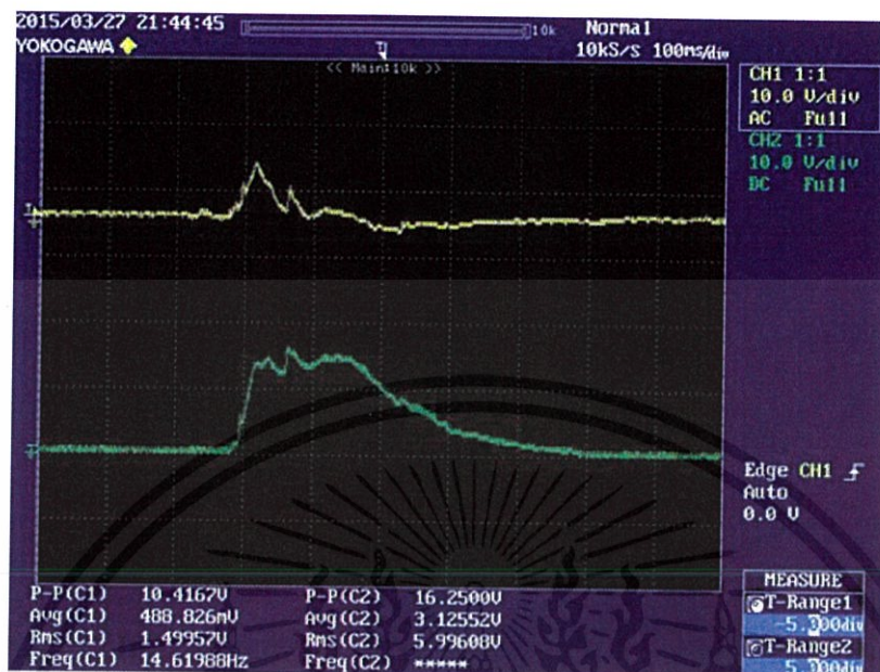
รูปที่ 4.36 รูปคลื่นสัญญาณแรงดันจากการเดินเทียบแผ่นเพียโซอิเล็กทริกจำนวน 4 แผ่น ต่อกันแบบคู่ขนานกันแล้วนำมาอนุกรมกัน
