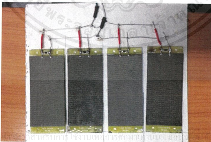
รูปที่ 4.45 การต่อวงจรขนานของแผ่น Piezoelectric
