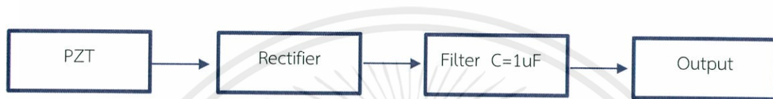
รูปที่ 5.1 ผังแสดงการทำงาน Application 2 วงจรต่อโหลด LED
