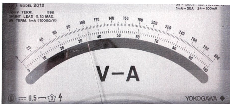
รูปที่ 4.48 ค่ากระแสที่วัดได้เมื่อผ่านวงจรขยายกระแส ซึ่งจาก V-A DC meter สามารถอ่านค่ากระแสได้ 35 mA หรือ 0.35 A
