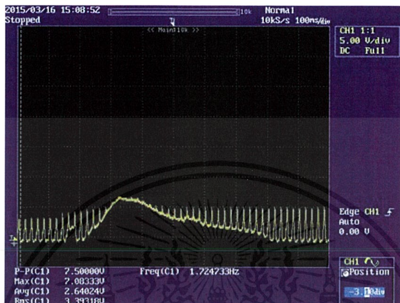
รูปที่ 4.16 รูปคลื่นสัญญาณแรงดันจากการเดินเหียบแผ่นเพียโซอิเล็กทริกจำนวน 2 แผ่นต่อวงจร อนุกรม
