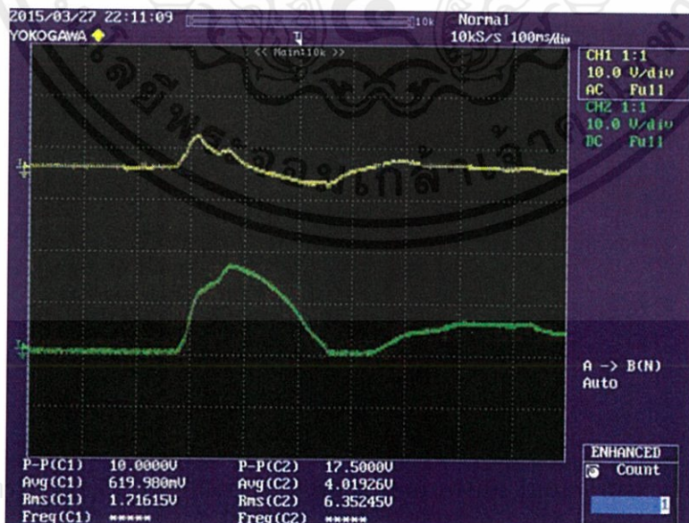
รูปที่ 4.31 รูปคลื่นสัญญาณแรงดันจากการเดินเหียบแผ่นเพียโซอิเล็กทริกจำนวน 1 แผ่น
