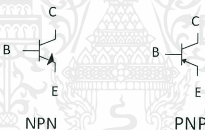
รูปที่ 2.25 โครงสร้างและสัญลักษณ์ของทรานซิสเตอร์
