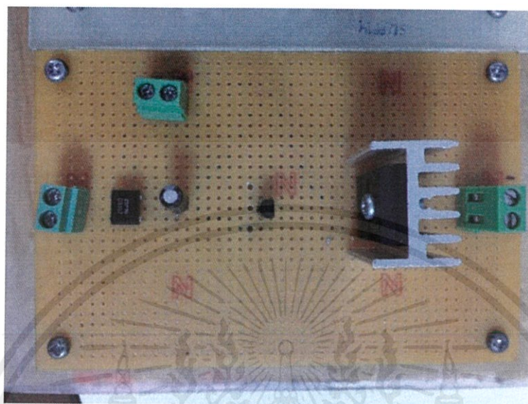
รูปที่ 4.46 อุปกรณ์ rectifier ต่อกับวงจรตัวเรียงกระแส
