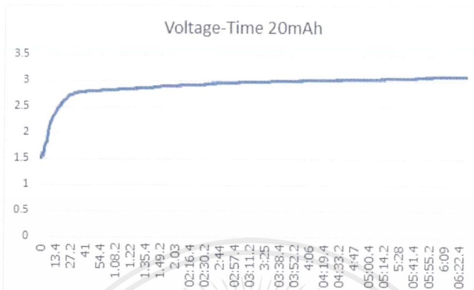
รูปที่ 4.9 กราฟคุณสมบัติการชาร์จระหว่าง แรงดันกับเวลาของแผ่นเพียโซอิเล็กทริก 2 แผ่นต่ออนุกรมขนาด 20 mAh
