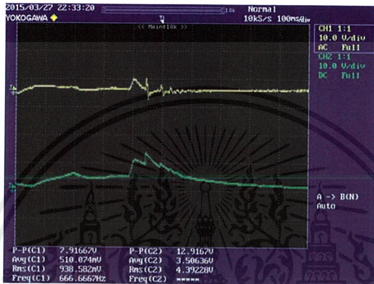
รูปที่ 4.38 รูปคลื่นสัญญาณแรงดันจากการเดินเหียบแผ่นเพียโซอิเล็กทริกจำนวน 1 แผ่น
