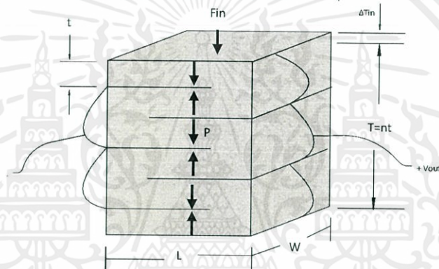
รูปที่ 2.12 Stack Generator
