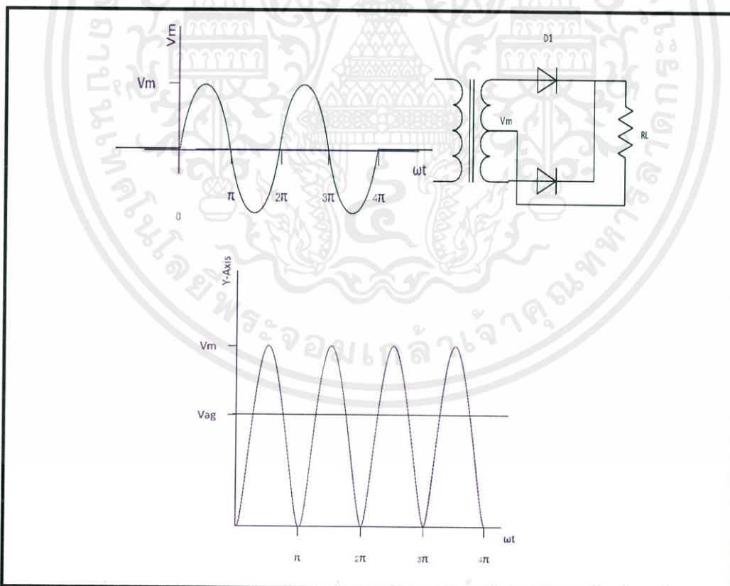
เอกสารนี้เป็นเอกสารทสงวนไว้สำหรับการใช้งานเพื่อการศึกษาเท่านั้น มิอนุญาตให้ทำซ้ำหรือเผยแพร่ในด้านการค้า ไม่ว่ากรณีใดๆทั้งสิ้น อีกทั้งยังขอสงวนลิขสิทธิ์ในเอกสารทุกครั้งที่มีการนำไปใช้ รูปที่ 2.19 วงจรเรียงกระแสเต็มคลื่นแบบเซ็นเตอร์แทป
