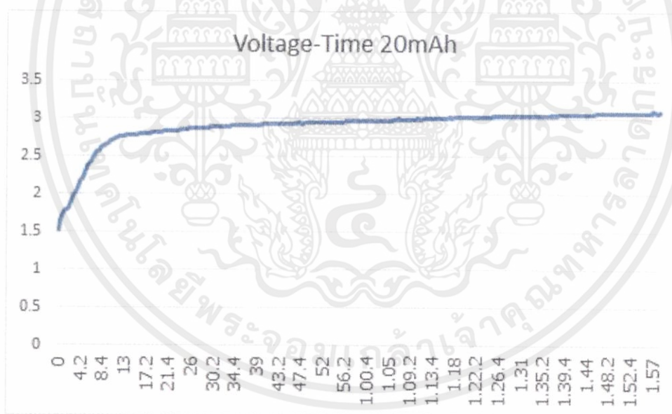
รูปที่ 4.10 กราฟคุณสมบัติการชาร์จระหว่าง แรงดันกับเวลาของแผ่นเพียโซอิเล็กทริก 2 แผ่นต่อขนานขนาด 20 mAh
