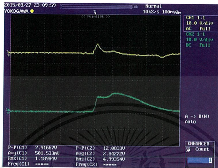
รูปที่ 4.44 รูปคลื่นสัญญาณแรงดันจากการเดินเหียบแผ่นเพียโซอิเล็กทริกจำนวน 4 แผ่น ต่อกัน แบบวงจรคู่อนุกรมกันแล้วนำมาขนานกัน
