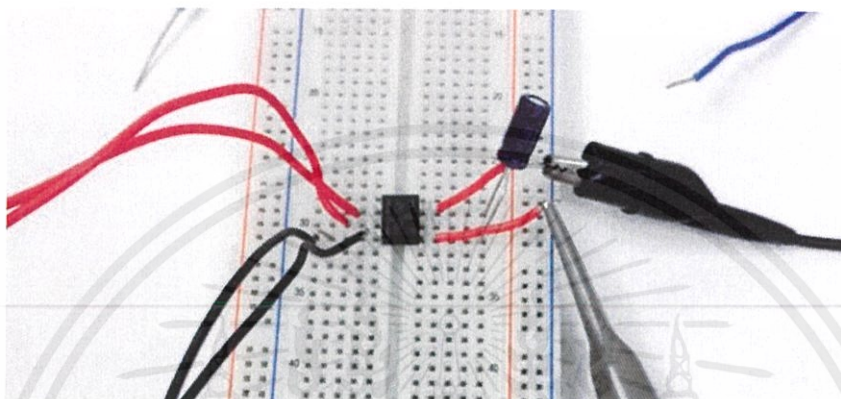
รูปที่ 4.22 การต่อ อุปกรณ์ IC bridge rectifier และ capacitor ขนาด 0.1 uF
