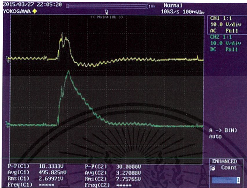
รูปที่ 4.34 รูปคลื่นสัญญาณแรงดันจากการเดินเหียบแผ่นเพียโซอิเล็กทริกจำนวน 4 แผ่น ต่อกัน แบบวงจรถูกอนุกรม
