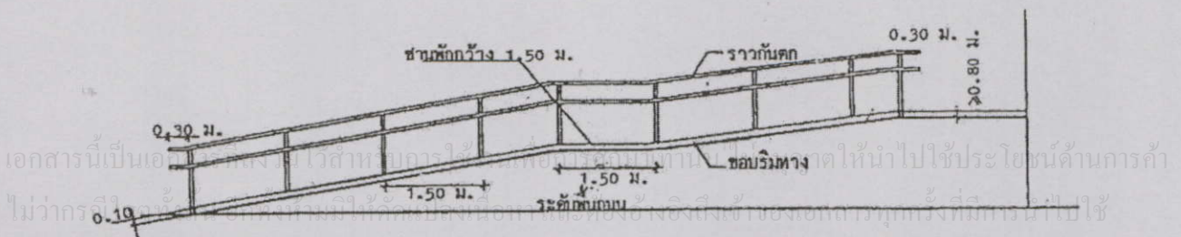
( รูปราวจับ หมายเลข 2 )
