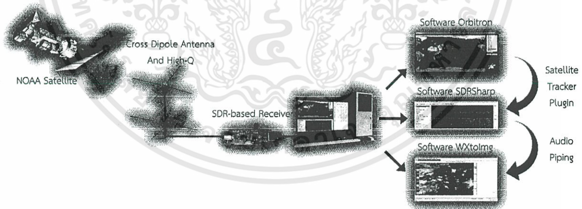
รูปที่ 1.1 Block Diagram ของระบบรับสัญญาณดาวเทียม
