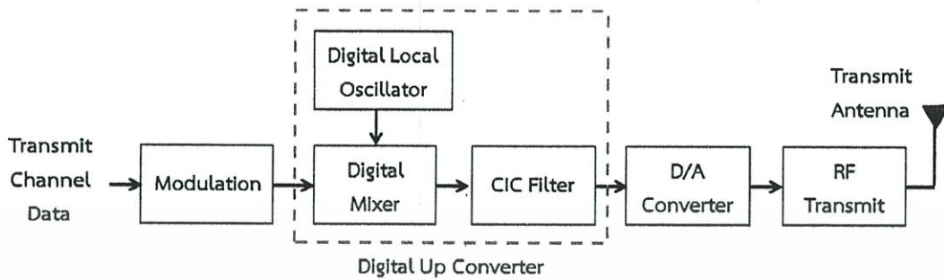
รูปที่ 2.14 Digital Up Converter
