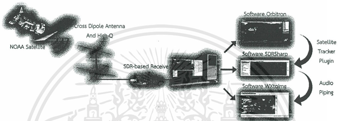
รูปที่ 3.1 Block diagram ของระบบรับสัญญาณดาวเทียม
