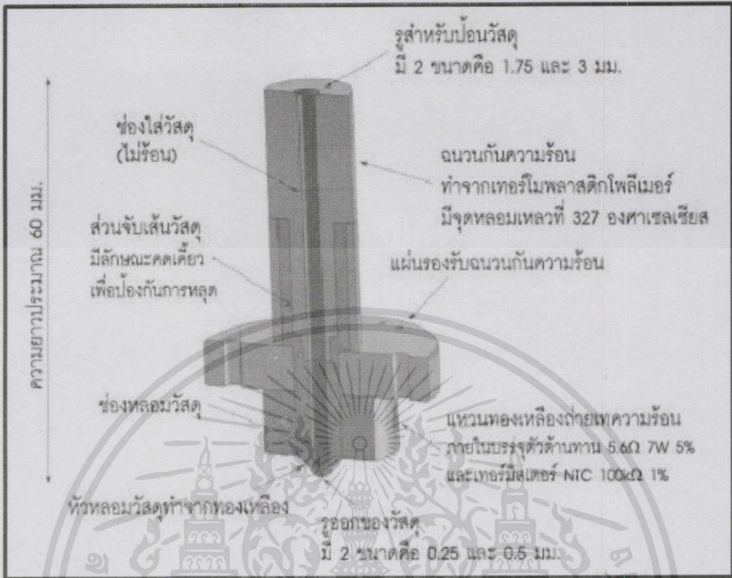
รูปที่ 2.10 โครงสร้างภายในของหัวฉีด
