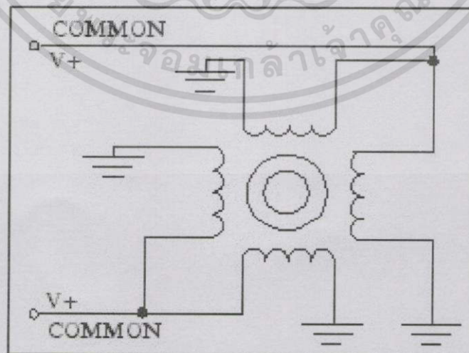
รูปที่ ข.3 ขดลวดภายในสเต็ปมิ่งมอเตอร์
