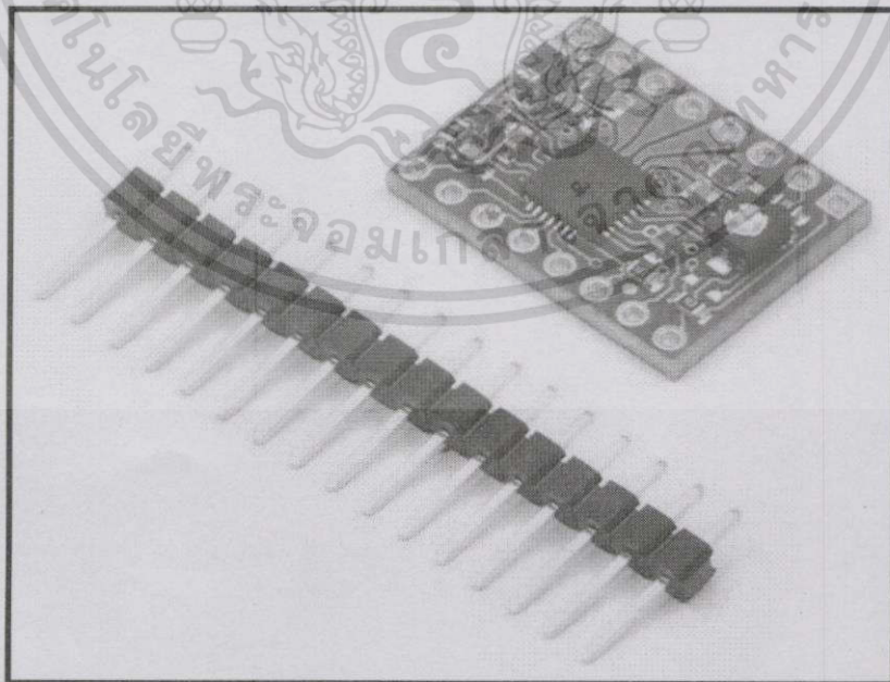
รูปที่ ก.8 Driver A4988
