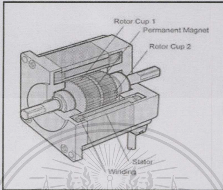
รูปที่ ข.2 โครงสร้างภายในของสเต็ปมิ่งมอเตอร์
