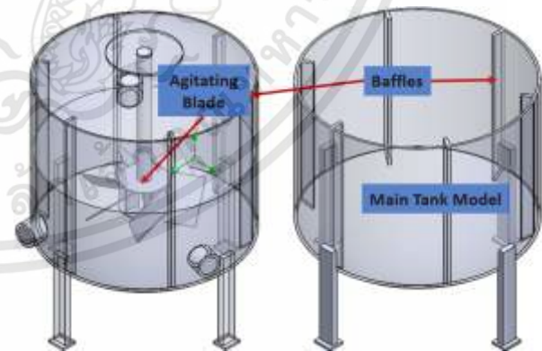
รูปที่ 3 ถังผสมที่ติดตั้ง Baffles และ ใบกวนผสม [9]
