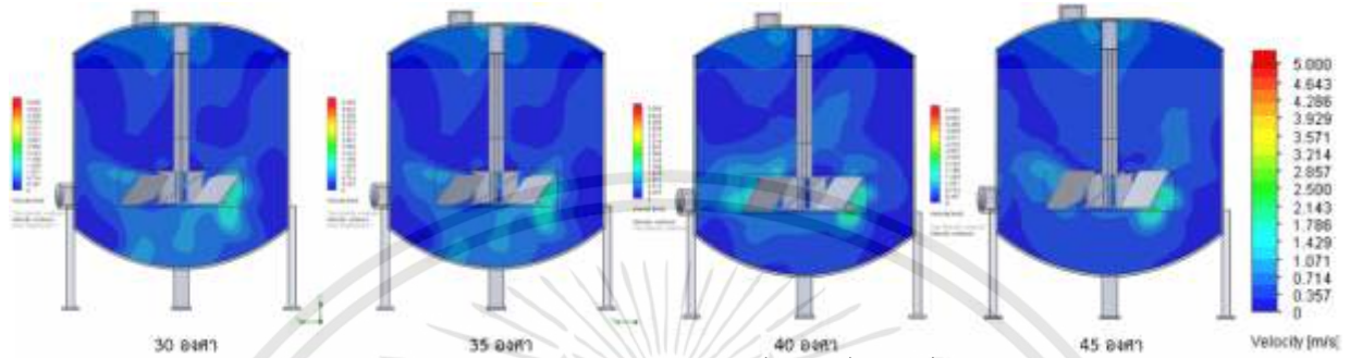
รูปที่ 5 แสดงสนามการไหลของของผสมระหว่างน้ำแอปเปิ้ลและน้ำที่เวลา 8 วินาที
