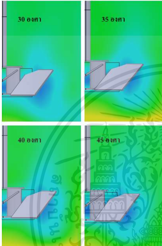
รูปที่ 10 แสดงการเปรียบเทียบความเข้มข้นในการผสมน้ำแอมป์เปลล์กับน้ำที่เวลา 8 นาที
