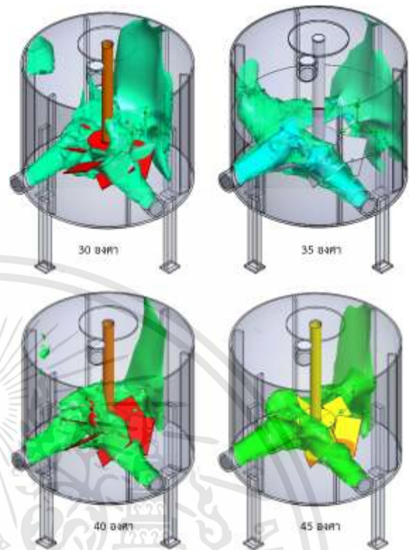
รูปที่ 11 การกระจายตัวของความเร็วที่ออกจากใบกวนผสม (Iso-Surface)
