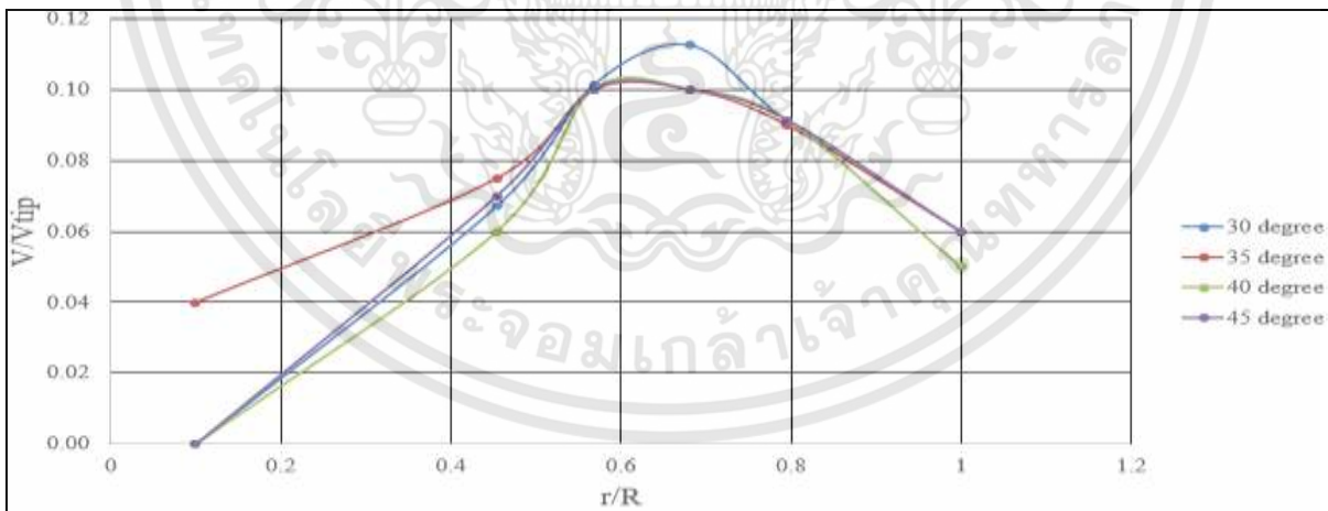
รูปที่ 9 ผลรวมของค่าความเร็ว V/V_{tip} ของมุมมองต่าง ๆ
