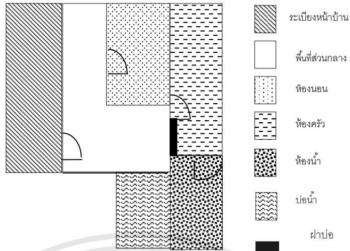
ภาพที่ 4.32 แสดงผังบ้านที่ยื่นออกไปในทะเล
