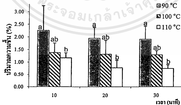
ภาพที่ 4.1 เปอร์เซ็นต์ความชื้นของผลิตภัณฑ์กล้วยแผ่นบางทอดกรอบที่ทอดภายใต้สุญญากาศที่เวลาและอุณหภูมิที่แตกต่างกัน
