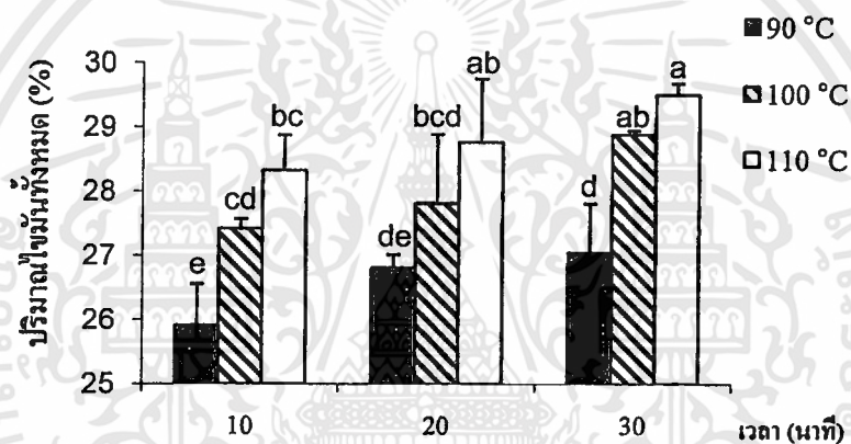
ภาพที่ 4.2 ปริมาณ ไขมันทั้งหมดของผลิตภัณฑ์กล้วยแผ่นบางทอดกรอบที่ผ่านการทอดแบบสุญญากาศ ที่เวลาและอุณหภูมิต่างกัน
