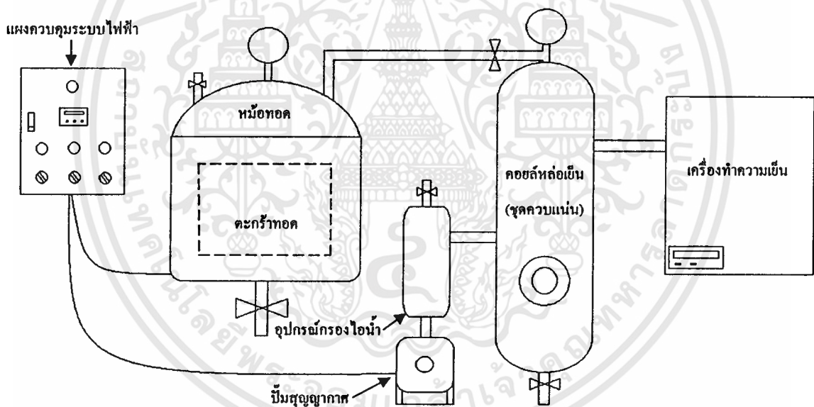
ภาพที่ 2.1 แผนผังเครื่องทอดสุญญากาศที่ใช้ในการทดลอง
