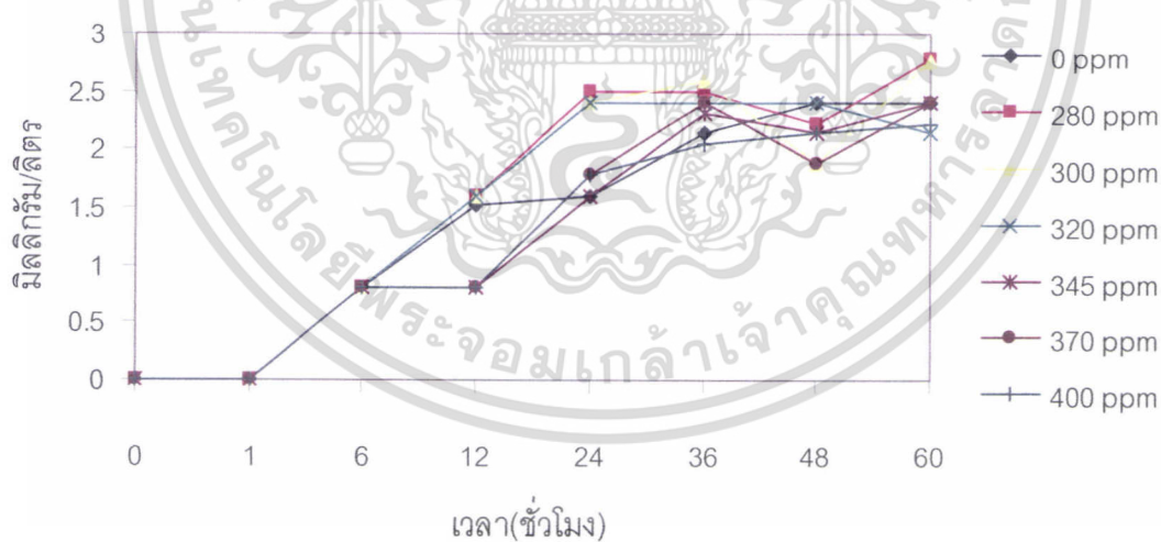
ภาพที่ 7 การเปลี่ยนแปลงปริมาณคาร์บอนไดออกไซด์ในการทดลองหาค่าความเป็นพิษเฉียบพลันของ 2-phenoxyethanol ต่อปลาสดเพศเมียภายในระยะเวลา 60 ชั่วโมง
