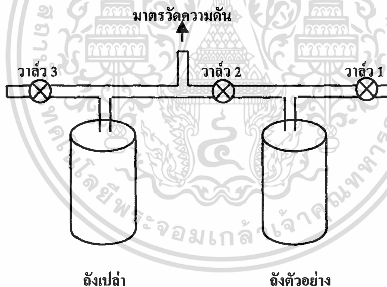
ภาพที่ 2.3 ผังส่วนประกอบของเครื่องพิคโนมิเตอร์แห้งแบบที่ 1
