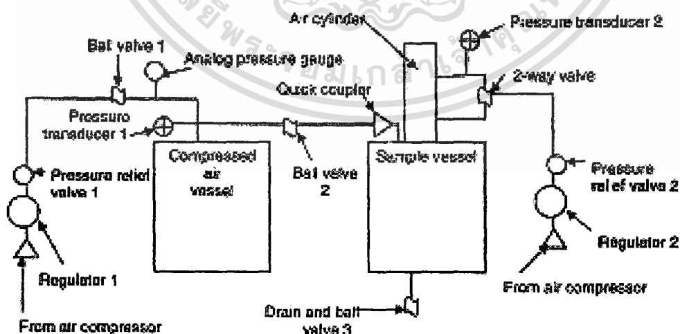
ภาพที่ 2.7 ผังเครื่องวัดความพรุนเพื่อใช้วัดปริมาตรช่องว่างอากาศอิสระของปฏิกิริยา
