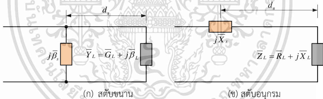
รูปที่ 2.20 ผังวงจรปรับตึงสตับ
