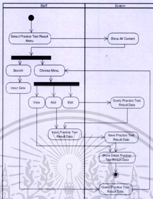
รูปที่ 4.8 แอกทिवิตีไดอะแกรมการทำงานตามยูสเคส Manage Practice Test Result Data
