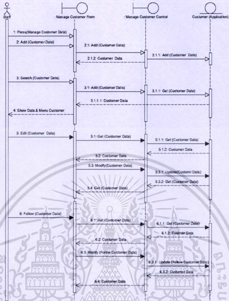
รูปที่ 4.16 ซีเควนซ์ไดอะแกรมการทำงานของ Application ตามยูสเคส Manage Customer Data
