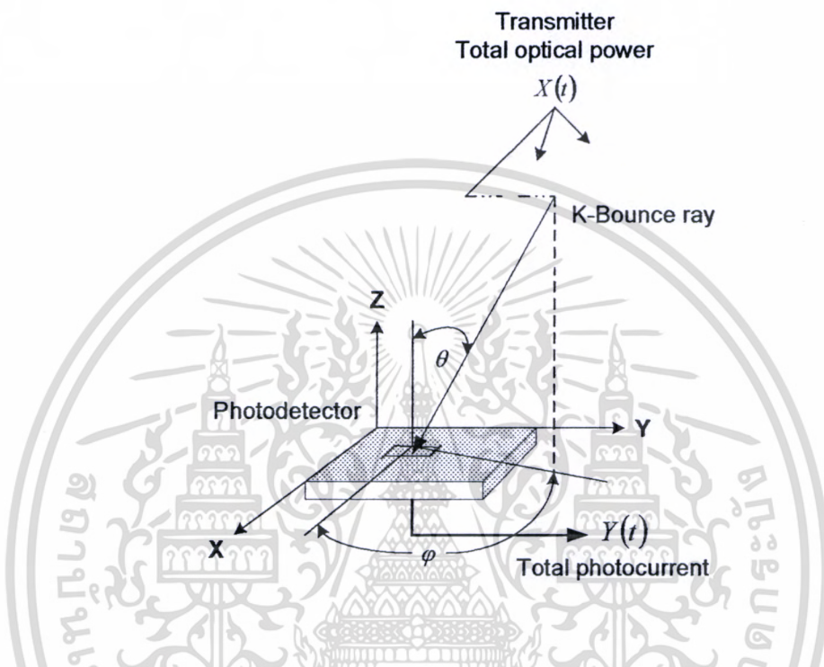
รูปที่ 2.6 แบบจำลองช่องสัญญาณอินฟราเรดที่พิจารณาในรูปของสนามไฟฟ้า
