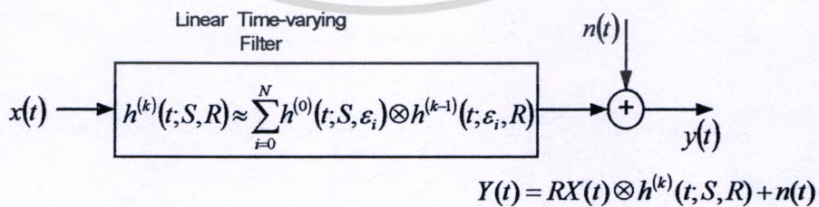
รูปที่ 2.28 แบบจำลองระบบทางคณิตศาสตร์ของช่องสัญญาณแบบ Diffuse link
