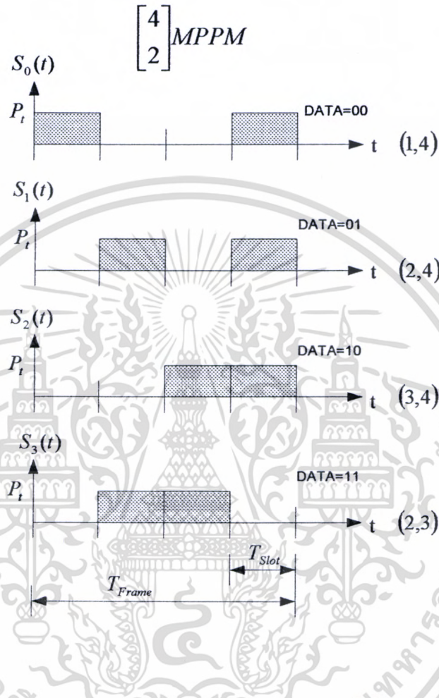
รูปที่ 3.13 การวางตำแหน่งพัลส์ลงบนเฟรมของการมอดูเลตแบบ \begin{bmatrix} 4 \\ 2 \end{bmatrix} MPPM
