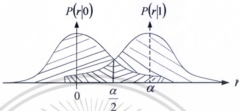
รูปที่ 4.7 ค่า PDF (Probability Density Function) ของตัวแปรแรนคอม r
