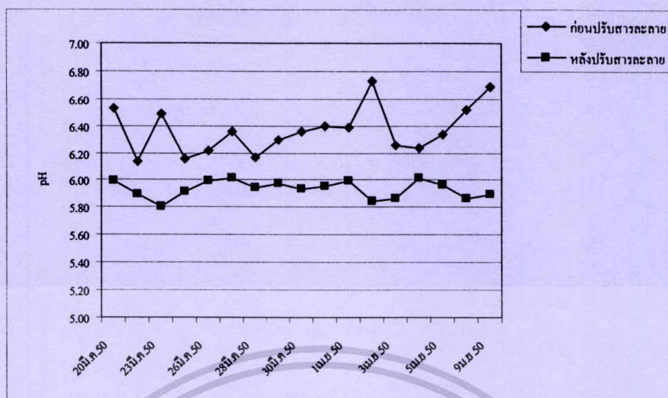
ภาพที่ ข.51 แสดงค่าความเป็นกรด-ด่าง (pH) ก่อนและหลังปรับสารละลายในบ่อปลูกที่ 1
