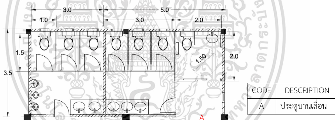
ภาพที่ 5.17 แพลนแสดงการแก้ไขห้องน้ำชั้นล่าง
