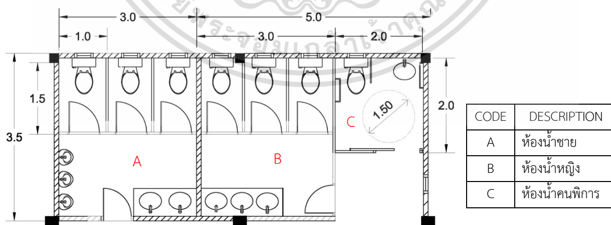
ภาพที่ 5.21 แพลนแสดงการแก้ไขห้องน้ำชั้นล่าง แยกห้องน้ำ ชาย-หญิง
