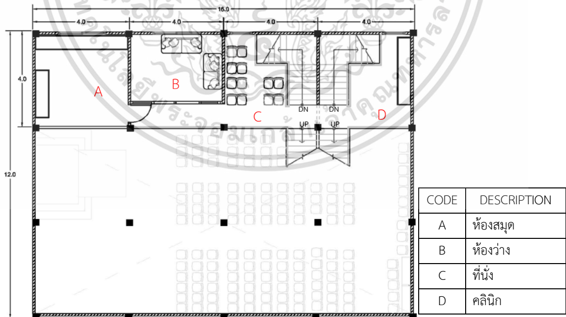
ภาพที่ 4.2 ภาพแสดงแปลนอาคารชั้นลอย
