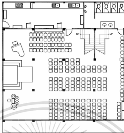
ภาพที่ 5.3 แพลนอาคารเดิม
