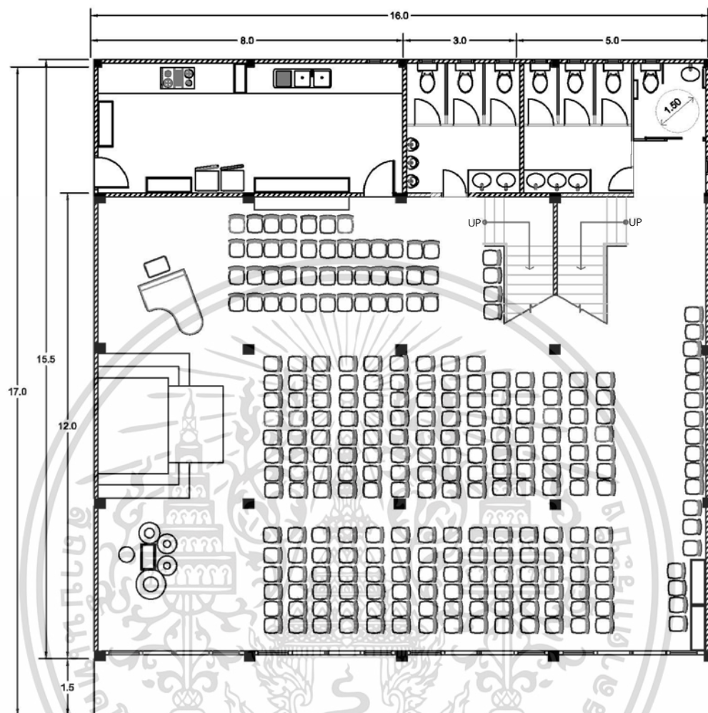
ภาพที่ 5.25 แปลนการแก้ไขชั้นล่าง
