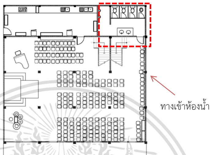
ภาพที่ 5.16 แพลนเดิมห้องน้ำชั้นล่าง
