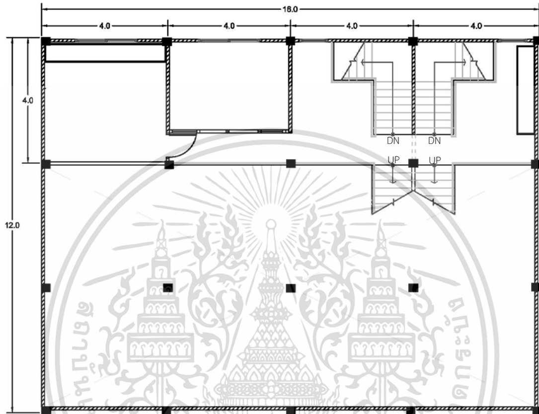
แปลนโครงสร้างอาคารชั้นลอย
