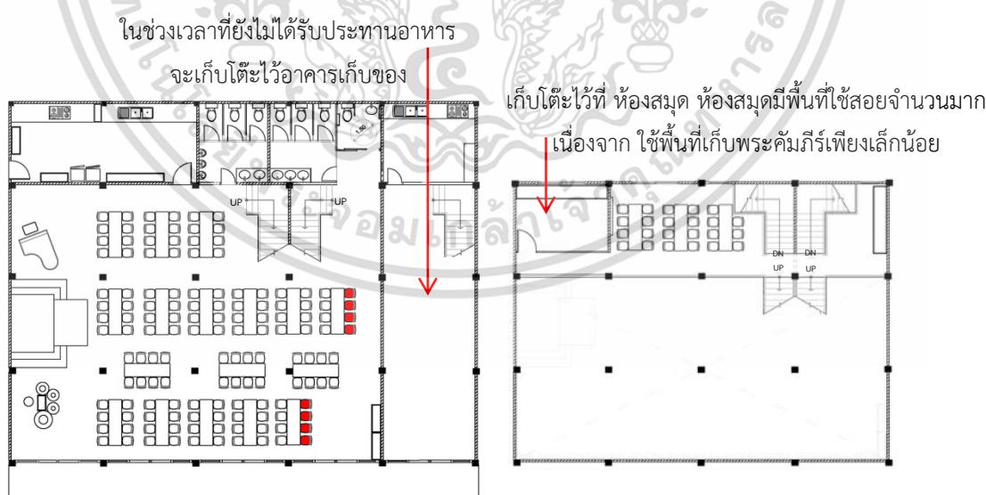
ภาพที่ 5.13 ภาพแสดงแผนการแก้ไขชั้นล่างและชั้นลอย โดยการจัดวางโต๊ะสำหรับรับประทานอาหารกลางวัน (เก้าอี้สีแดง คือพื้นที่สำหรับคนที่ใช้วีลแชร์นั่ง) โดยสามารถนั่งรับประทานอาหารได้ 159 คน จากของเดิม 80 คน
