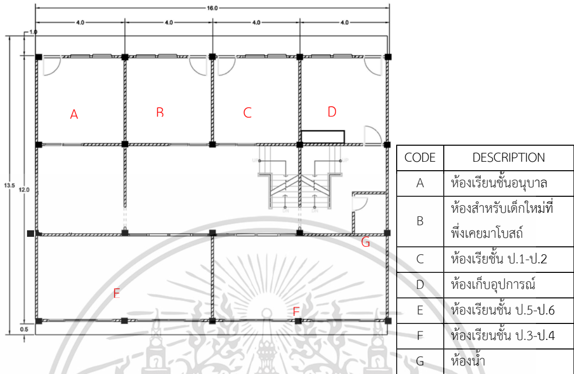
ภาพที่ 4.3 ภาพแสดงแปลนอาคารชั้นสอง
