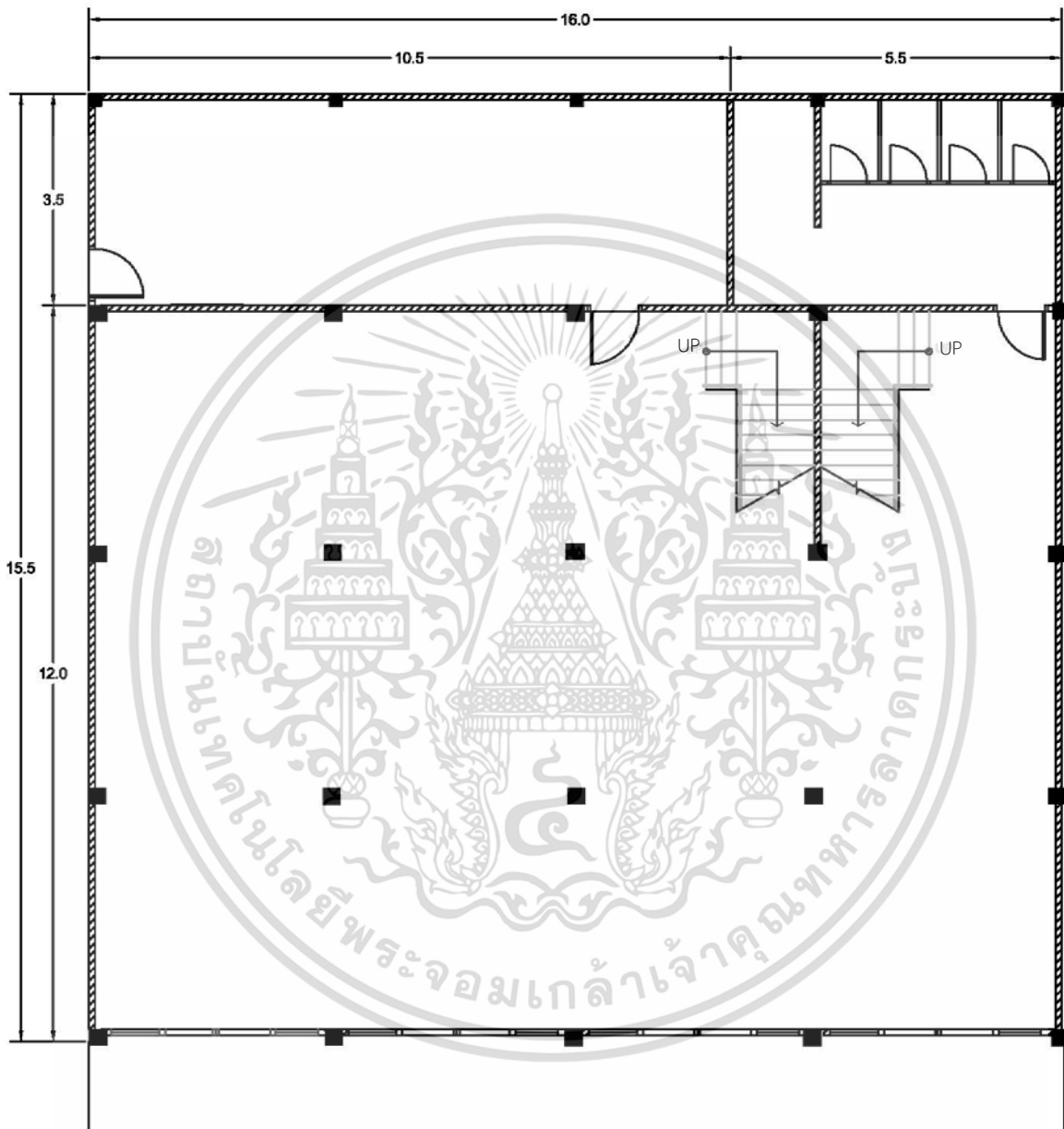
แปลนโครงสร้างอาคารชั้นล่าง
