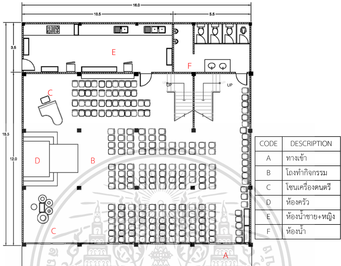
ภาพที่ 4.1 ภาพแสดงแปลนอาคารชั้นล่าง
