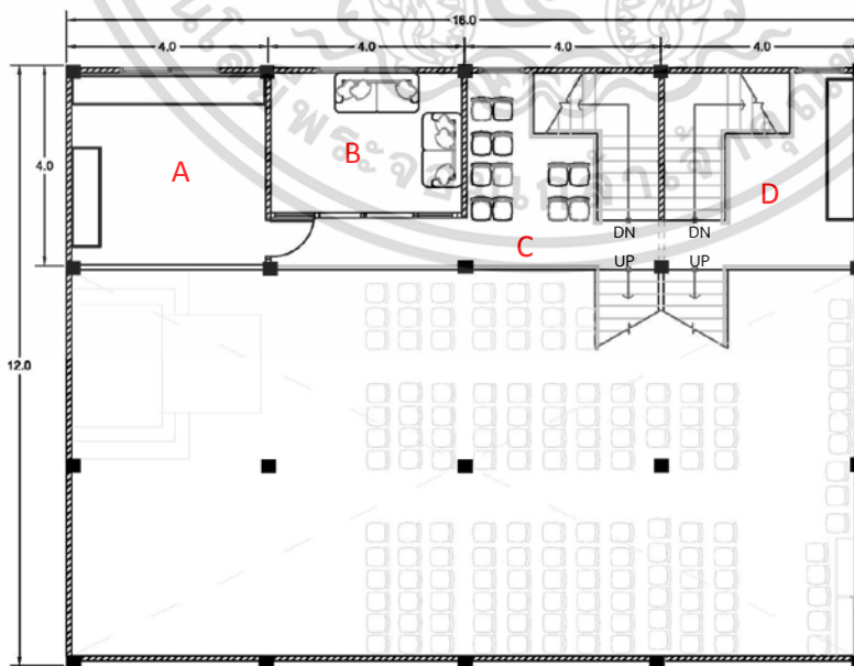
ภาพที่ 5.2 ภาพแสดง แปลนเดิมอาคารชั้นลอย
