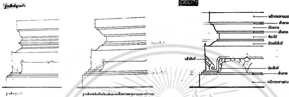
รูปที่ 2.10 รานพระอุโบสถชนิดรานสิงห์ลูกแก้ว
