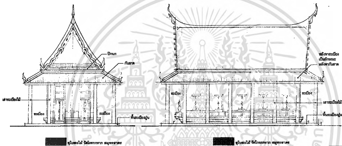
รูปที่ 2.26 ด้านหน้าและด้านข้าง อุโบสถไม้ วัดโกรงกราง จังหวัดสมุทรสาคร
