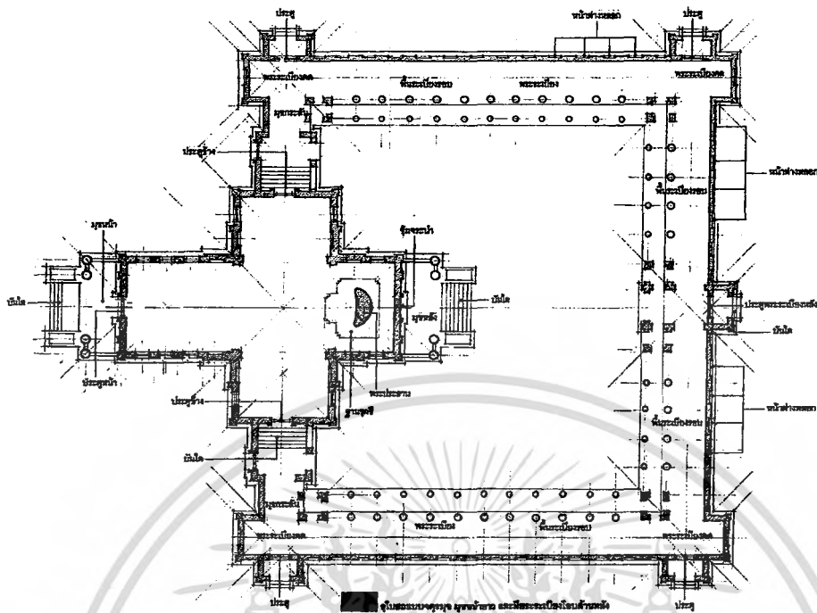
รูปที่ 2.27 ผังพื้น อุโบสถแบบจตุรमुख มุขหน้ายาว และมีพระระเบียงโอบค้ำด้านหลัง
