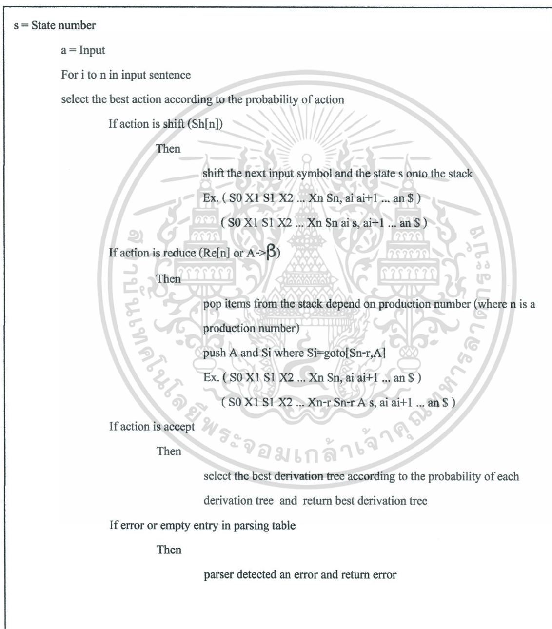
รูปที่ 3.13 แสดงขั้นตอน Parsing Process
