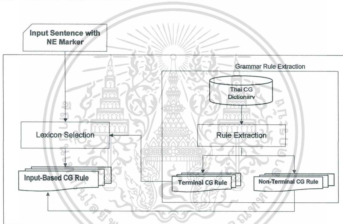
รูปที่ 3.2 แสดงขั้นตอน Grammar Rule Extraction
