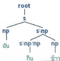
รูปที่ 3.14 แสดงต้นไม้ไวยากรณ์ที่วิเคราะห์ได้
