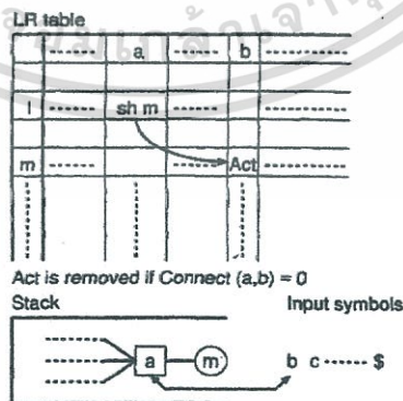
รูปที่ 3.11 แสดงการเชื่อมต่อเมทริกซ์และตาราง Parsing Table
