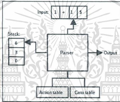
รูปที่ 2.2 แสดงตัวอย่างกระบวนการวิเคราะห์คำในประโยคแบบ LR
