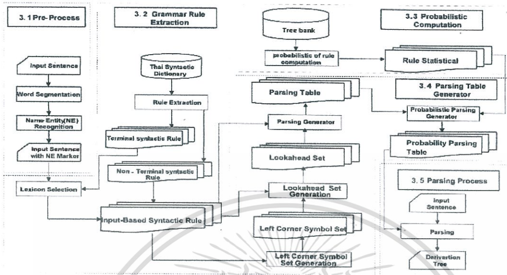
รูปที่ 2. ขั้นตอนการทำงานของระบบแก้ข้อความแบบ PGRE
