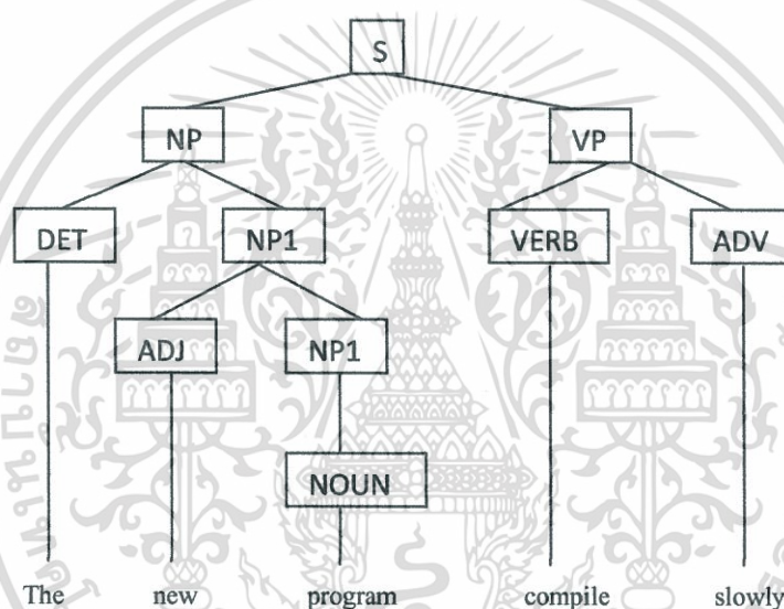
รูปที่ 2.1 แสดงต้นไม้ที่วิเคราะห์ได้
