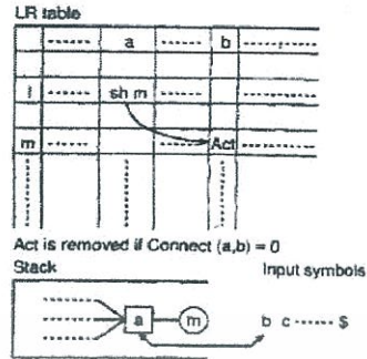
รูปที่ 3 แสดงการเชื่อมต่อเมทริกซ์และตาราง Parsing Table
