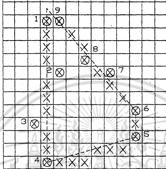
รูปที่ 4.1 แสดงขอบของข้อมูลภาพมีการเว้นและแหง และเกิดจุดเปลี่ยนแนวเส้น ที่ 2, 3, 7 และ 8 ขึ้น เมื่อหาจุดเปลี่ยนแนวเส้นโดยใช้วิธีใน หัวข้อ 3.3.1
