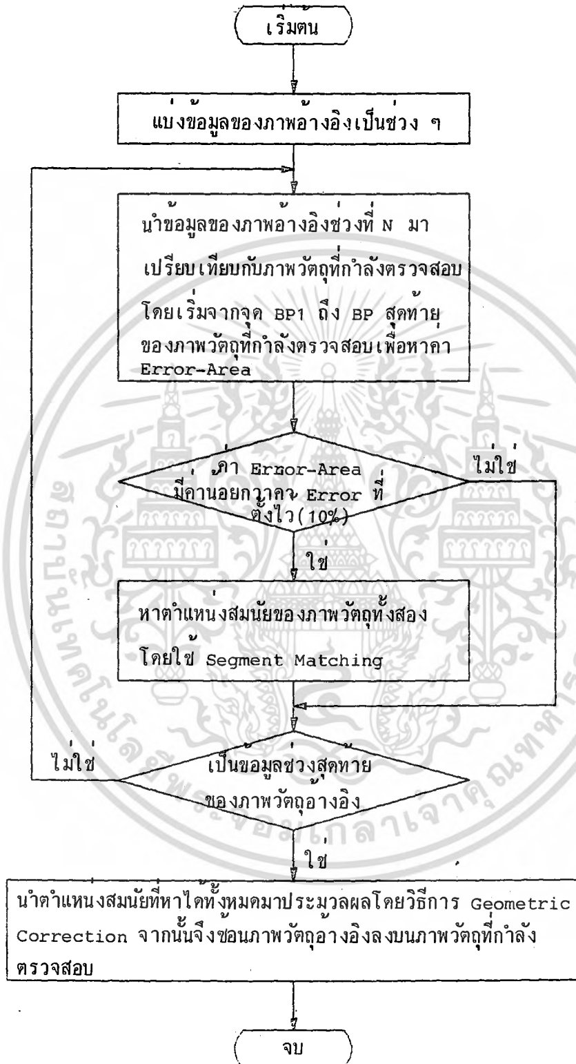
ผังที่ 5.1 ขั้นตอนการหาวัตถุที่มีบางส่วนถูกบิดเบือน
