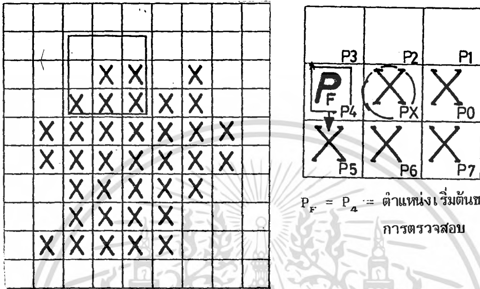
รูปที่ 2.8 แสดงตำแหน่งเริ่มต้นการกวาดรอบตารางหน้าตาต่าง ซึ่งหาได้จากการทำงานในขั้นตอนที่ 2 หรือ 5
