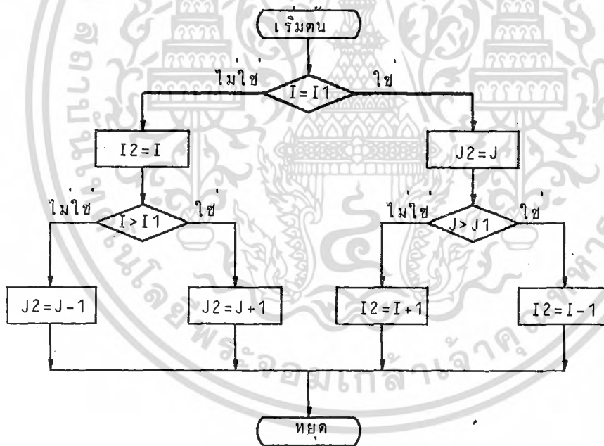
ผังที่ 2.2 แสดง Subroutine RIGHT ( I, J, I1, J1, I2, J2 )
