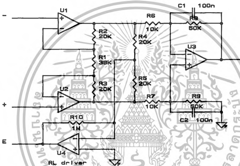
รูปที่ 3.2 วงจรขยายความแตกต่าง ประกอบด้วยออปแอมป์ 3 ตัว และ วงจร RL driver
