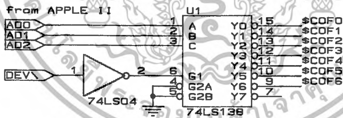
รูปที่ 4.16 วงจรสร้างพอร์ทควบคุม
