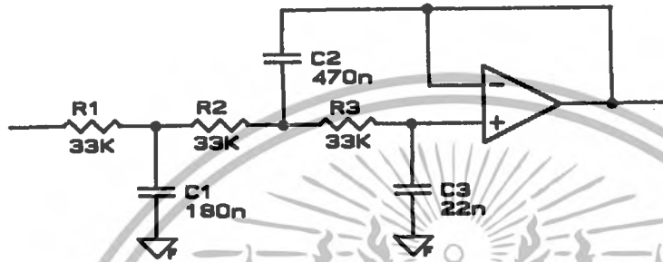
รูปที่ 3.5 วงจรกรองความถี่ต่ำกว่า 50 Hz ผ่าน
