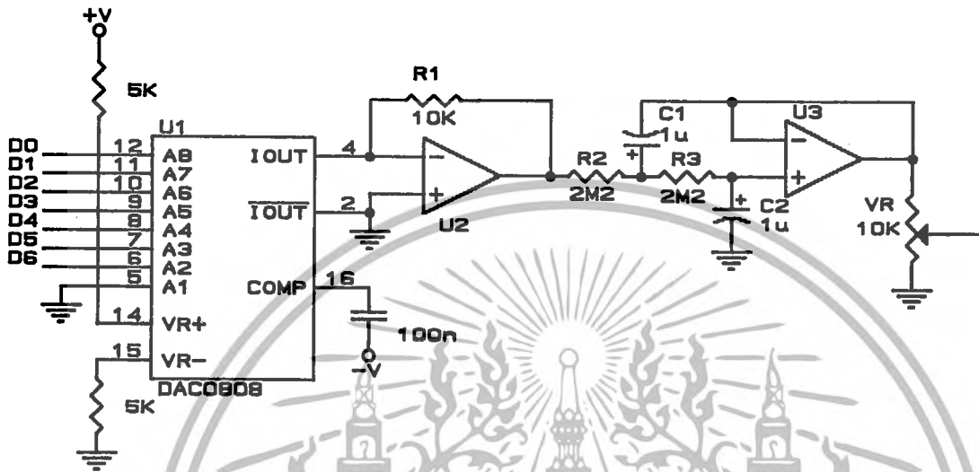
รูปที่ 3.30 วงจรแปลงสัญญาณดิจิทัลเป็นอนาล็อก
