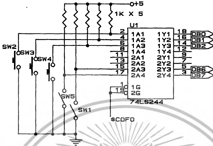
รูปที่ 4.17 วงจรสวิตช์ตั้งค่านิกัดสัญญาณเตือนและเลือกแบบแสดงผล
