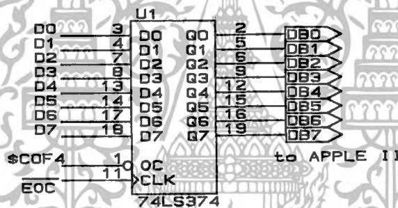
รูปที่ 4.19 วงจรรับข้อมูลจาก A/D เข้าไมโครคอมพิวเตอร์
