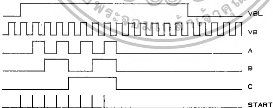
รูปที่ 4.3 ลักษณะของสัญญาณควบคุมการทำงานของ A/D
