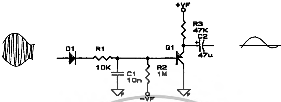
รูปที่ 3.10 วงจรแยกความถี่ต่ำ
