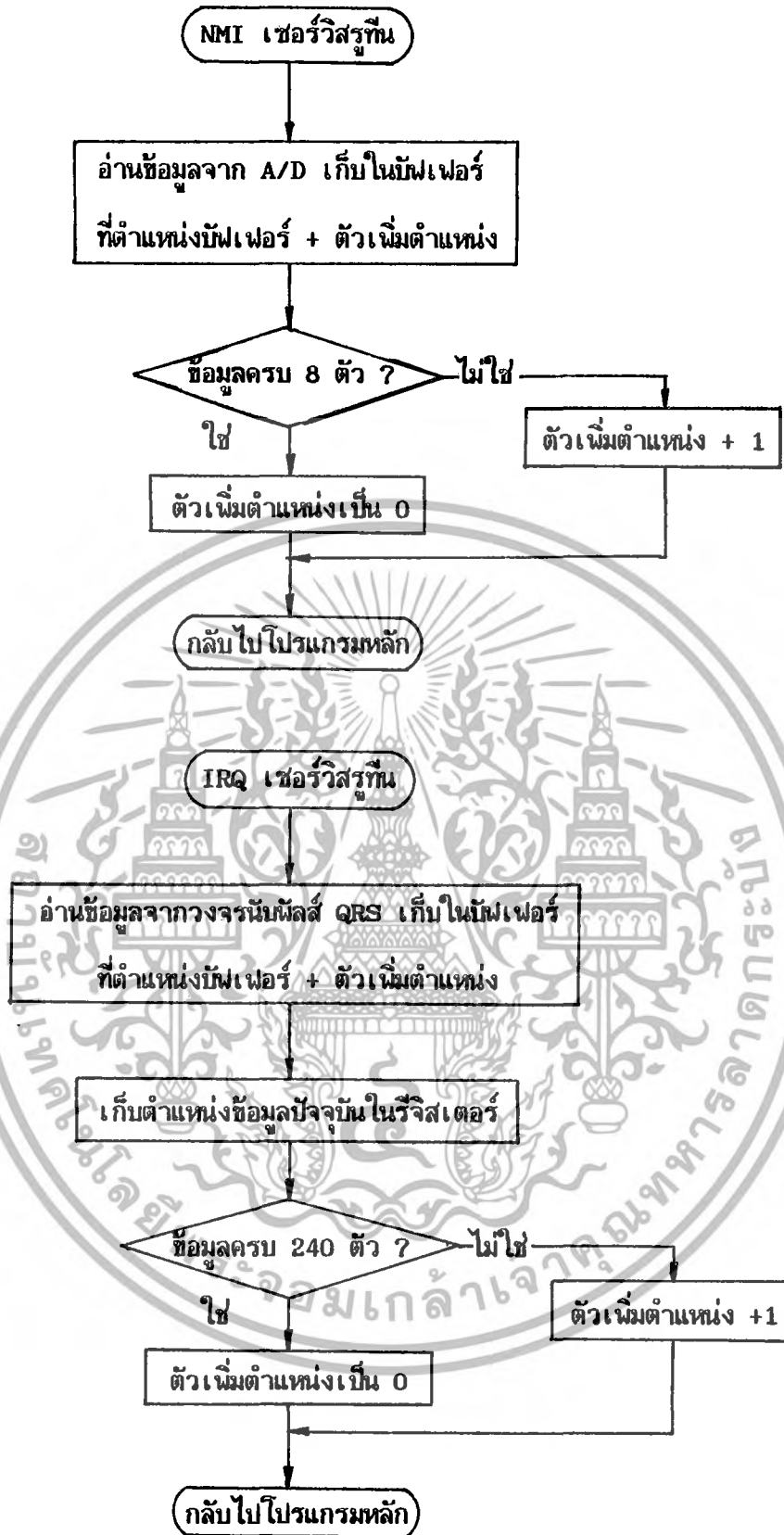
รูปที่ 4.25 โฟลว์ชาร์ทแสดงอินเทอร์รัพท์ เซอร์วิสเซอรูน
