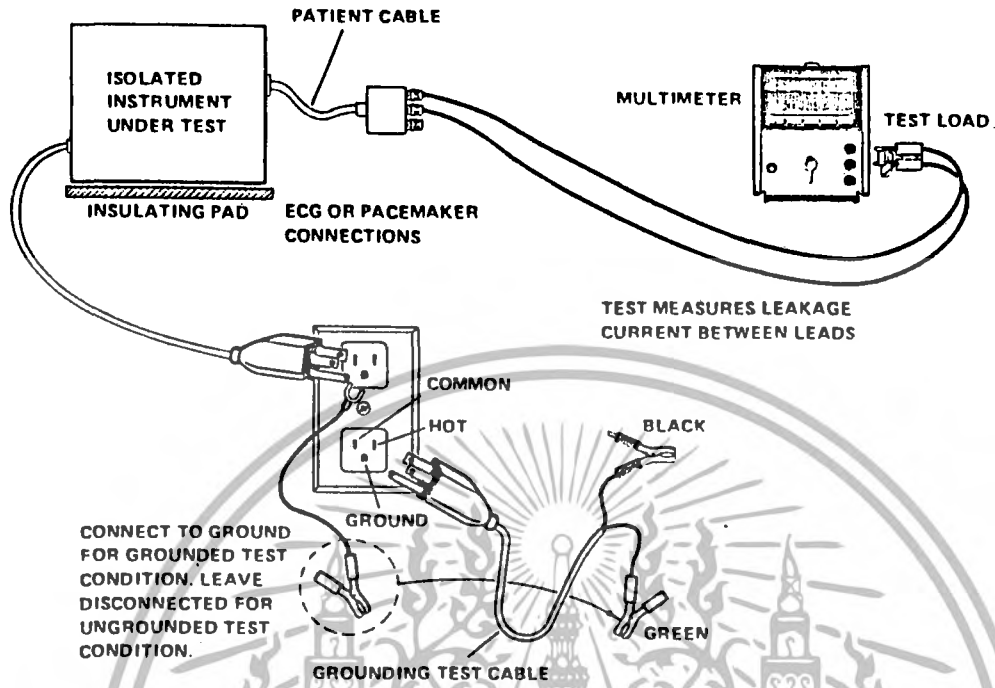
รูป ค-2 การวัดกระแสรั่วระหว่างสายรับสัญญาณ
