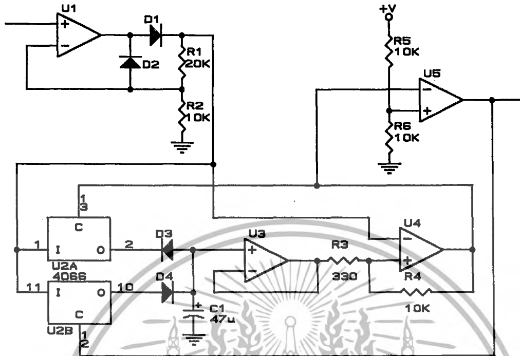
รูปที่ 3.26 วงจรตรวจจับขอบบนและขอบล่างของคลื่น
