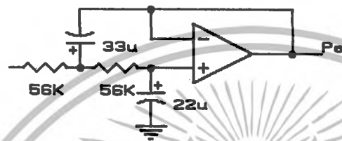
รูปที่ 3.38 วงจรกรองความถี่ต่ำผ่านลำดับสองที่ความถี่คutoff 0.3 Hz
