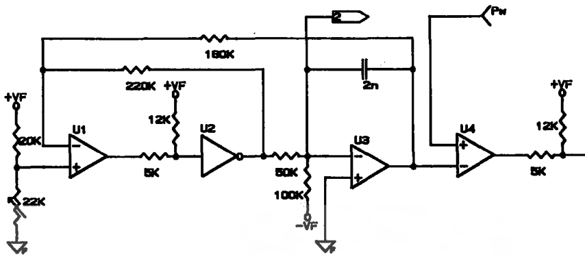
รูปที่ 3.14 แสดงวงจรพัลส์วิดท์มอดูเลเตอร์
