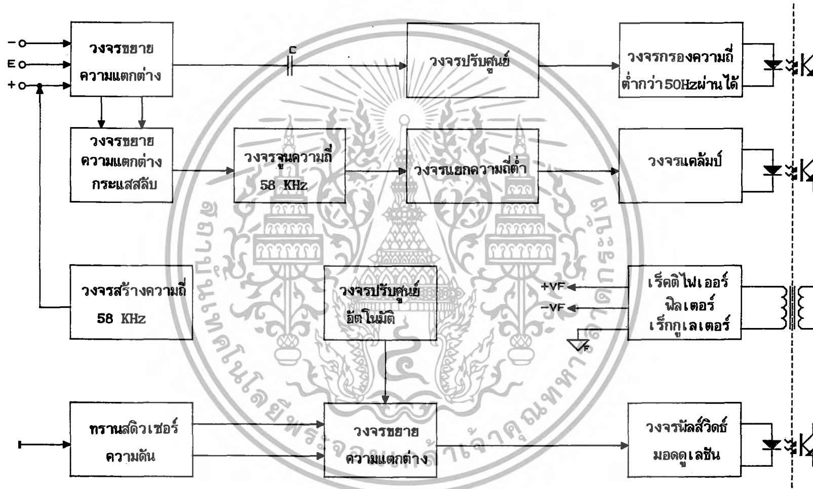
รูปที่ 3.1 แผนผังวงจรรับสัญญาณจากร่างกาย
