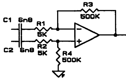
รูปที่ 3.8 วงจรขยายความแตกต่างกระแสลับ
