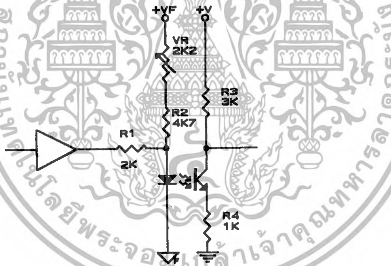
รูปที่ 3.6 วงจรส่งผ่านสัญญาณด้วยแสง
