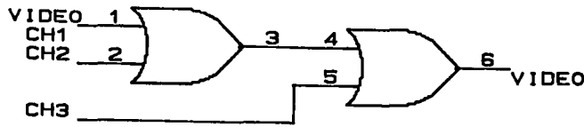
รูปที่ 4.15 วงจรรวมสัญญาณภาพทั้ง 3 ช่อง
