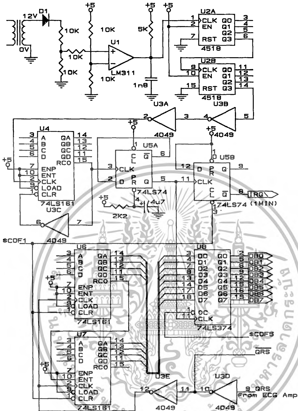
รูปที่ 4.20 วงจรสร้างฐานเวลา 1 นาทีและวงจรบีบอัด QRS
