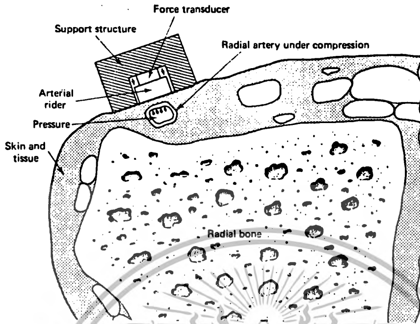
รูปที่ 1.20 การวัดแรงดันโลหิตโดยใช้หลักการของโทโมมิเตอร์
