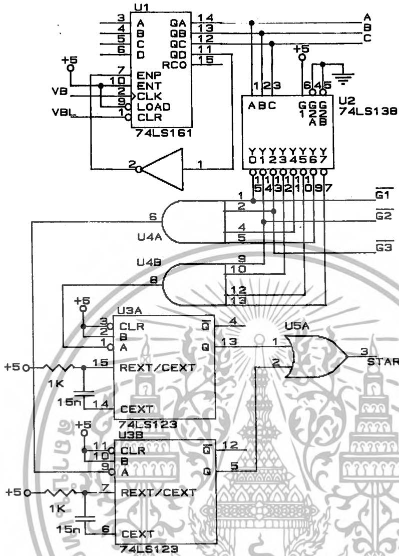
รูปที่ 4.2 วงจรควบคุมการทำงานของ A/D
