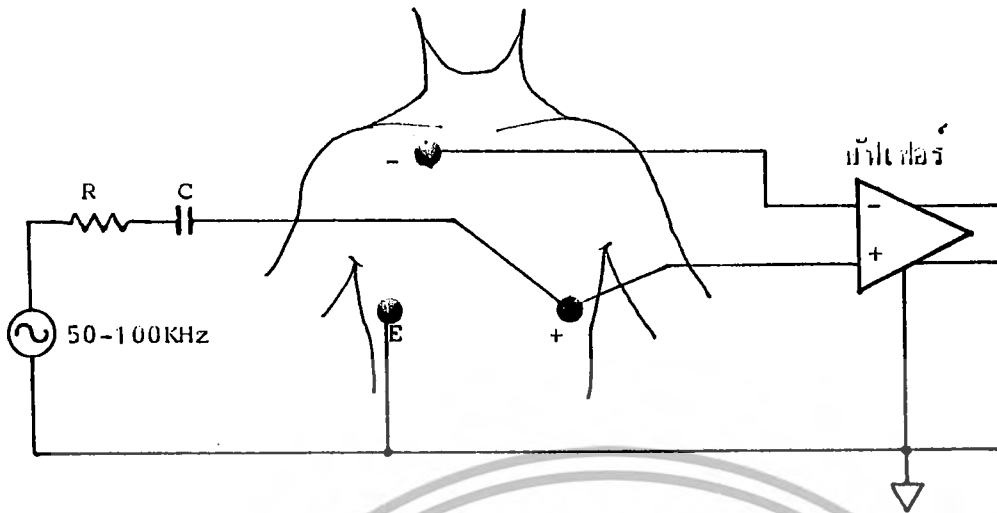
รูปที่ 1.15 แสดงการใช้โอเลคโตรดร่วมกันของการวัดคลื่นไฟฟ้าหัวใจกับการวัดการหายใจ
