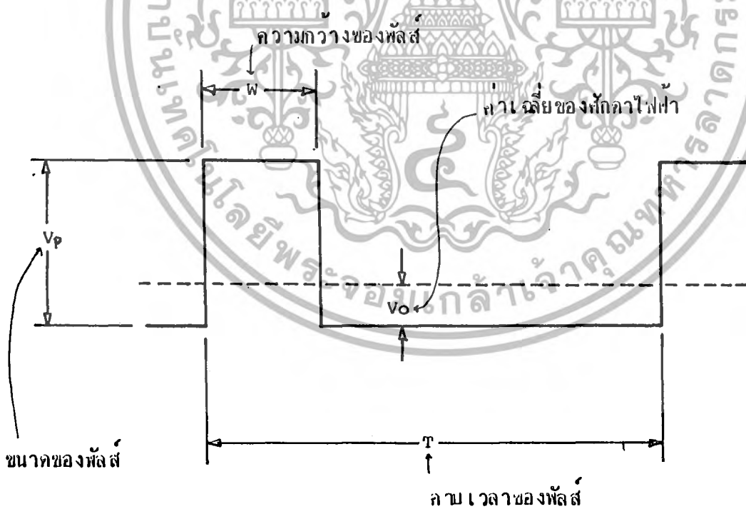
รูปที่ 3.21 แสดงหลักการแปลงความถี่เป็นสัญญาณไฟฟ้า
