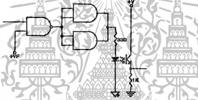
รูปที่ 3.15 แสดงวงจรส่งผ่านด้วยแสง
