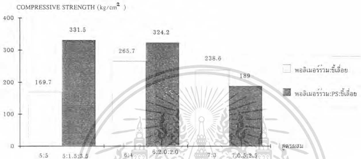
รูปที่ 5.7 แสดงการเปรียบเทียบค่าความแข็งแรงต่อแรงอัดของสูตรผสม ซีลี้อย ที่เตรียมโดยใช้ตัวทำละลาย
