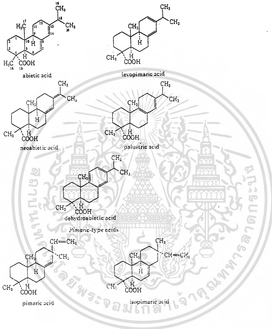
รูปที่ 2.1 แสดงโครงสร้างของเรซินแอซิด ชนิดต่าง ๆ
