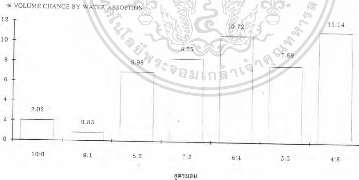
รูปที่ 5.10 แสดงค่าร้อยละการเปลี่ยนแปลงปริมาตรเนื่องจากการดูดซึมน้ำของสูตรผสม
