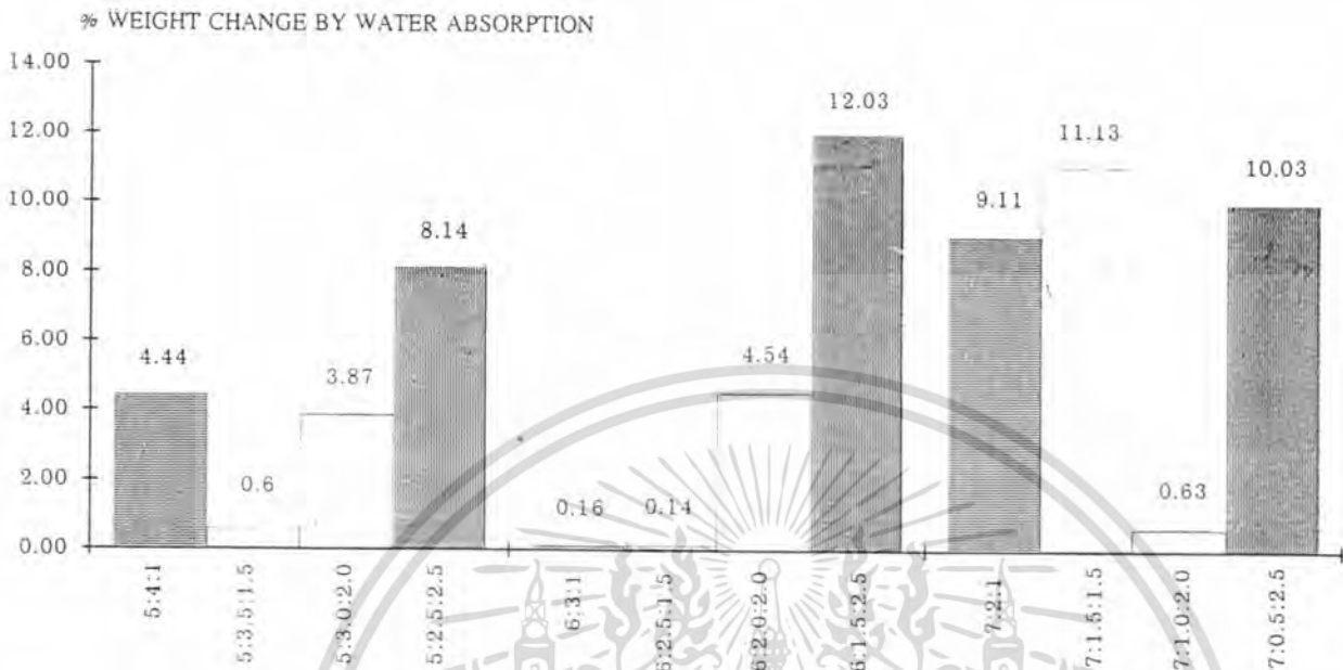
รูปที่ 5.15 แสดงร้อยละการเปลี่ยนแปลงน้ำหนักเนื่องจากการดูดซึมน้ำของสูตรผสม พอลิเมอร์รวม LDPE และ ซีล้อย
