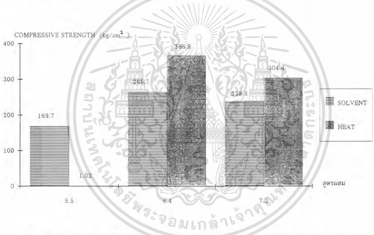
รูปที่ 5.17 แสดงการเปรียบเทียบความแข็งแรงต่อแรงอัดของสูตรผสมพอลิเมอร์รวมกับซีลี้อยที่เตรียมโดยวิธีใช้ตัวทำละลาย และวิธีใช้ความร้อน
