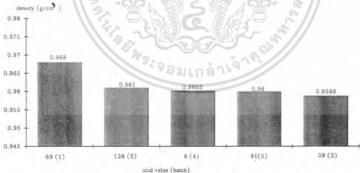
รูปที่ 5.20 แสดงค่าความหนาแน่นของน้ำมันชกเงาแบบตซ์ต่าง ๆ
