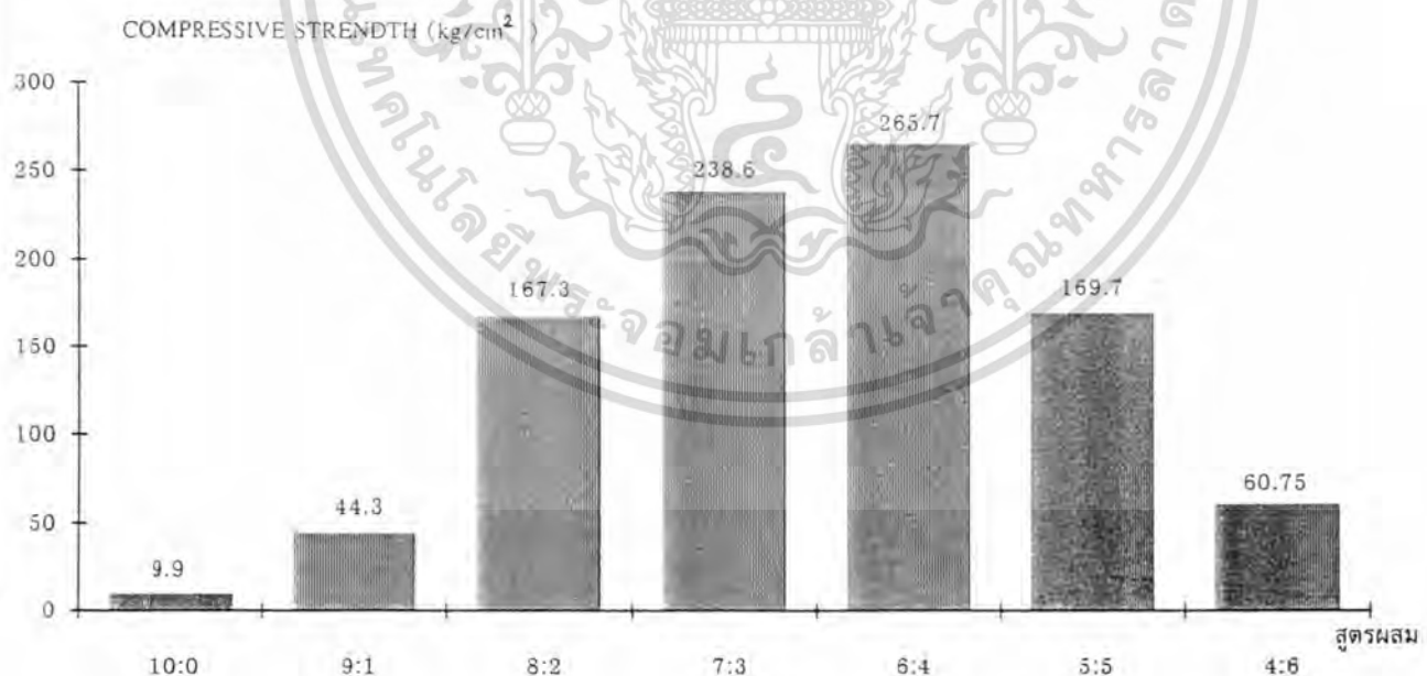
รูปที่ 5.5 แสดงความสัมพันธ์ระหว่างความแข็งแรงต่อแรงอัดกับสูตรผสม พอลิเมอร์รวมกับซีลีอีย ซึ่งเตรียมโดยวิธีใช้ตัวทำละลาย และใช้ระยะเวลาในการอบชิ้นงาน 7 วัน
