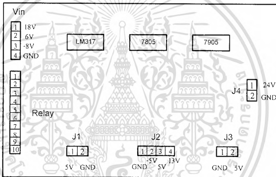
รูปที่ ก.1 แผนผังอุปกรณ์และจุดเชื่อมต่อของวงจรถงแหล่งจ่ายไฟฟ้า
