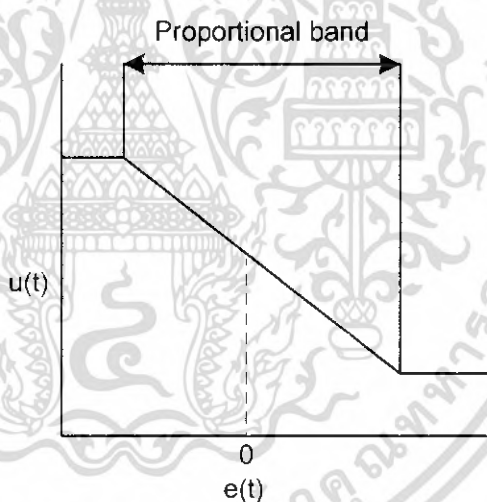
รูปที่ 2.1 การกำหนดช่วงจำกัดของเอาต์พุต
