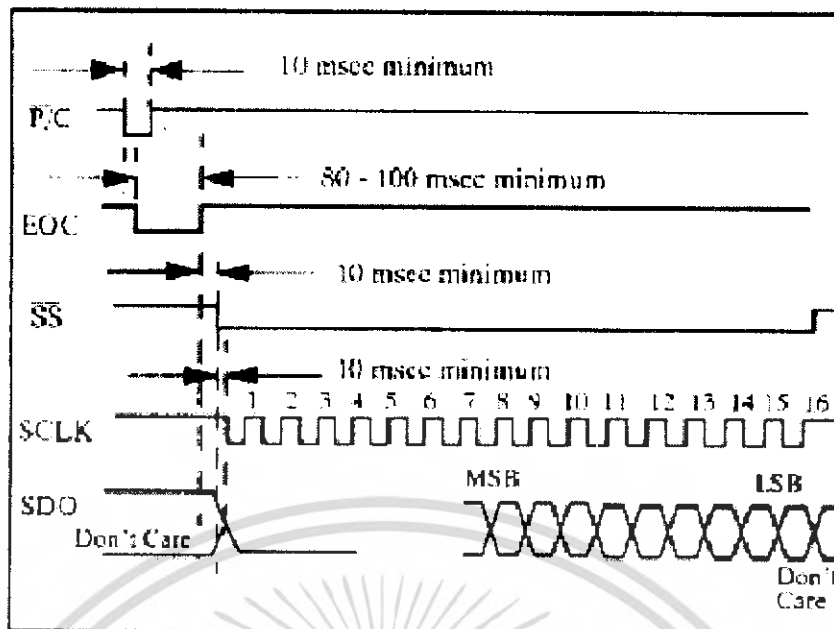
รูปที่ 2.17 ไตอะแกรมเวลาแสดงการทำงานในสถานะที่เป็นสเลฟ
