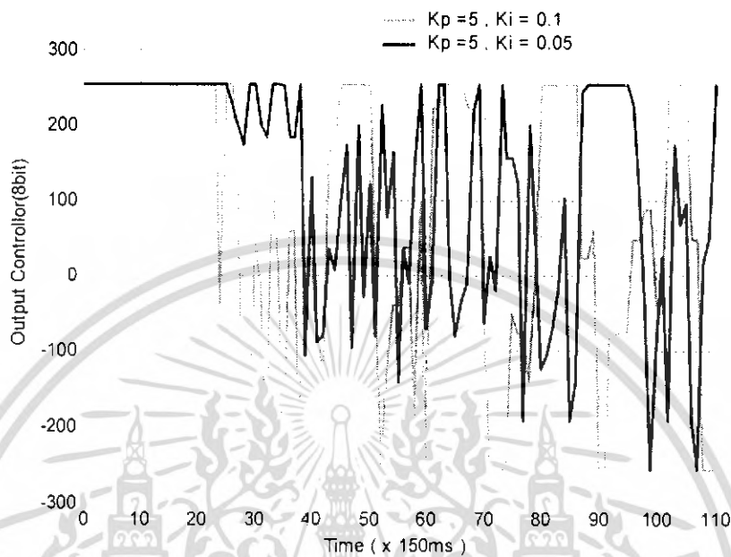
รูปที่ 4.8 สัญญาณอินพุทของมอเตอร์ในการควบคุมแบบพีไอโดยแปรค่า K_i
