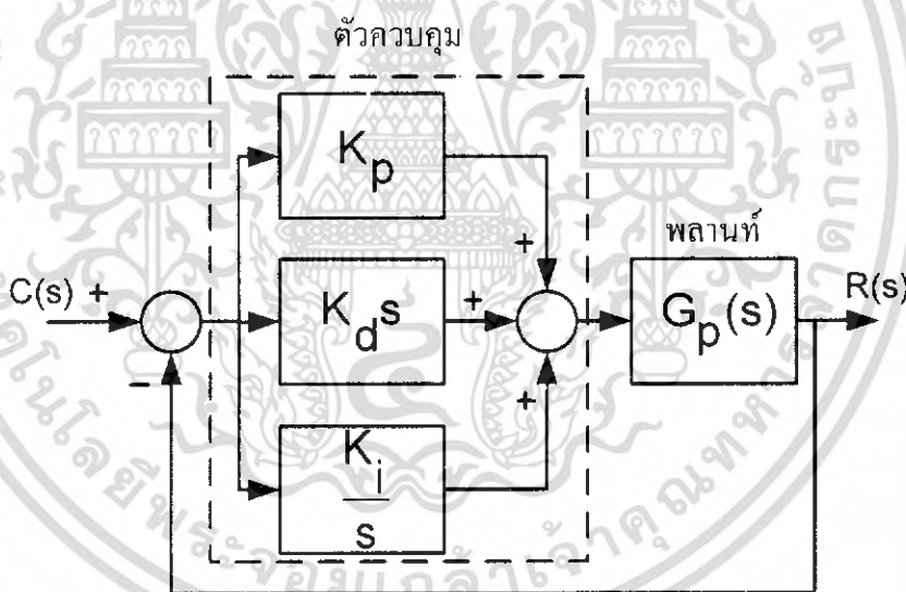
รูปที่ 2.11 บล็อกไดอะแกรมของระบบควบคุมแบบพีไอดี
