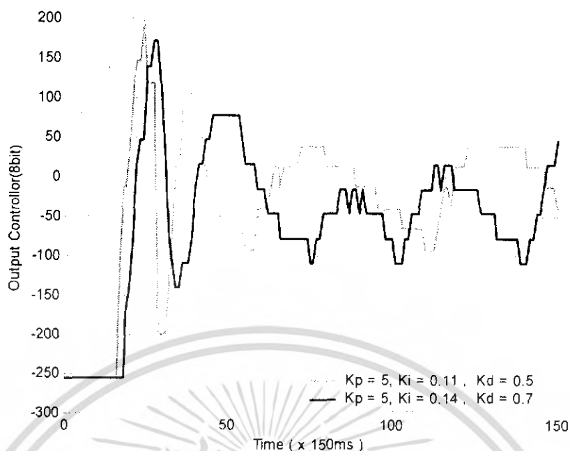
รูปที่ 4.20 สัญญาณอินพุทของมอเตอร์ในการควบคุมแบบพีไอดีโดยแปรค่า K_i และ K_d
