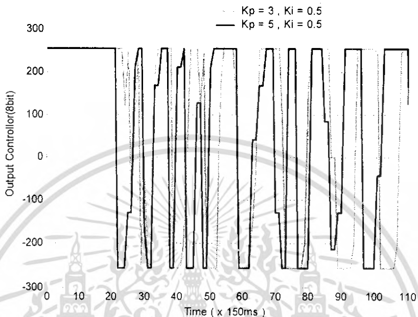
รูปที่ 4.6 สัญญาณอินพุทของมอเตอร์ในการควบคุมแบบพีไอโดยแปรค่า K_p
