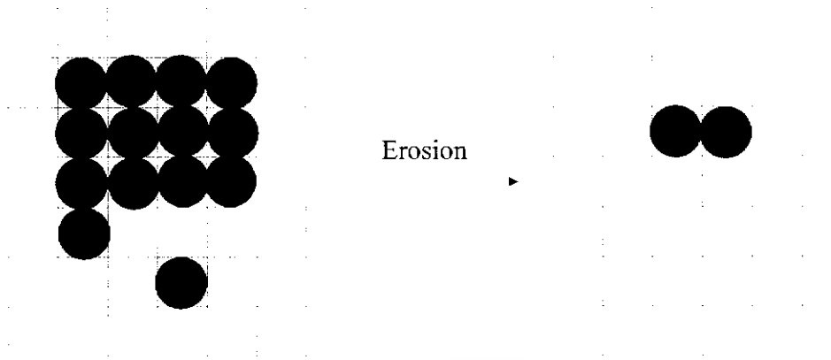
รูปที่ 2.4 การทำอีรอสัน A \ominus B
