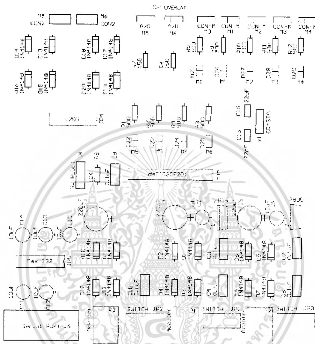
รูปที่ 3.18 อุปกรณ์ต่างๆ ภายในลายวงจร
