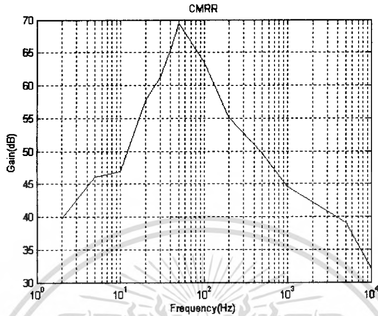
รูปที่ 4.5 กราฟแสดงค่า CMRR
