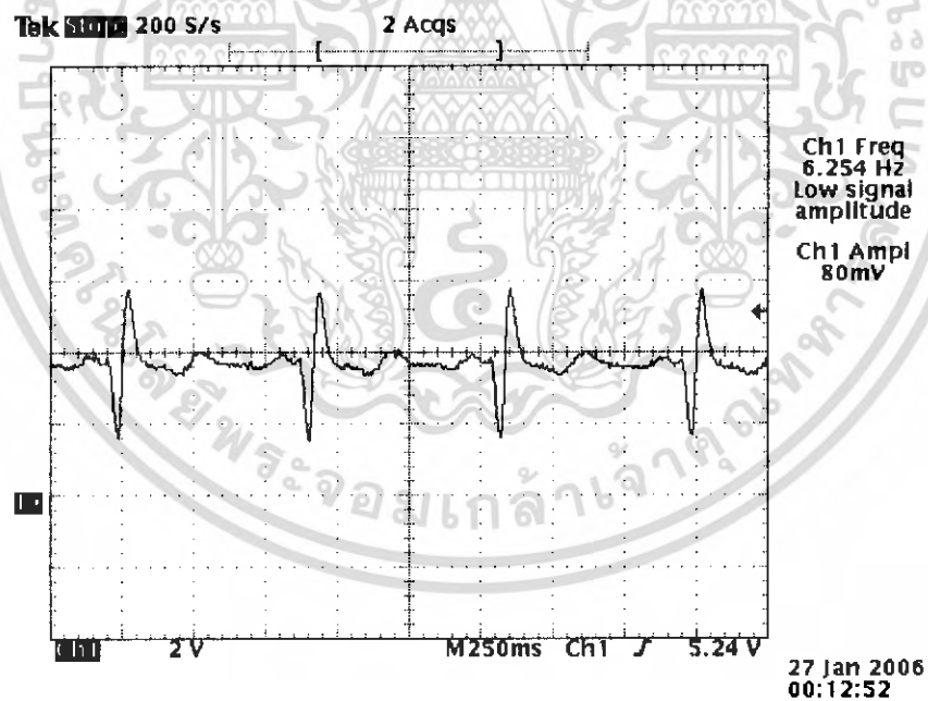
รูปที่ 4.6 รูปสัญญาณโดยใช้ออสซิลิโสมิเตอร์
