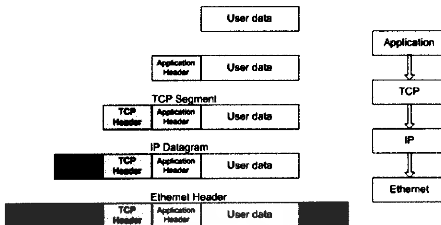
รูปที่ 2.8 ขั้นตอนการ encapsulation เมื่อข้อมูลถูกส่งผ่านโปรโตคอลต่างๆ
