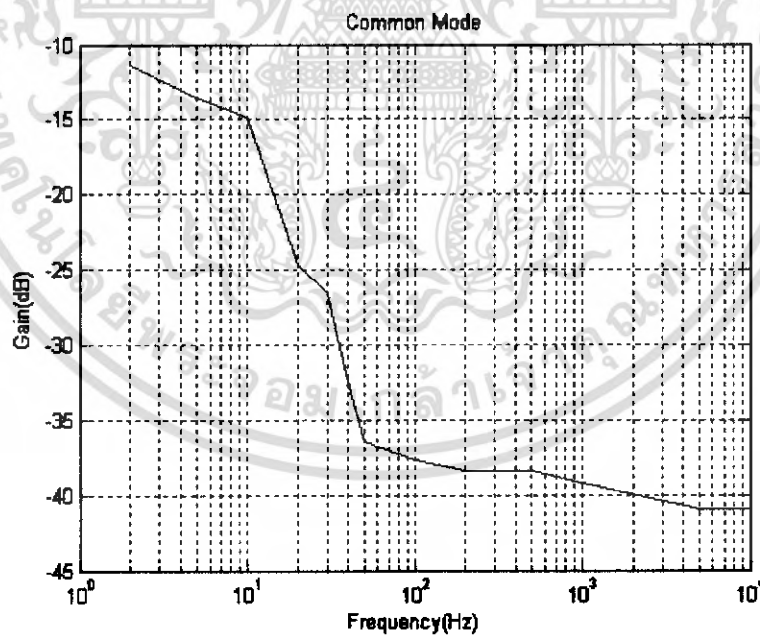
รูปที่ 4.4 กราฟแสดงอัตรขยายของวงจรขยายแบบคอมมอนโหมด
