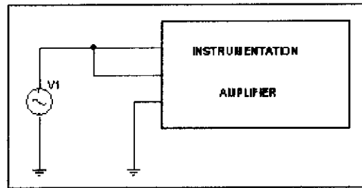
รูปที่ 4.2 วงจรที่ใช้หาอัตราขยายของวงจรขยายแบบคอมมอนโมด
