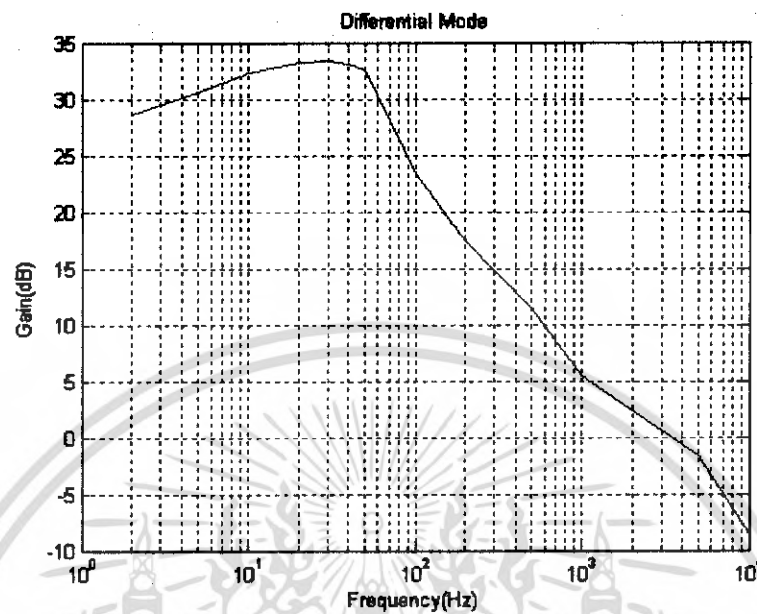
รูปที่ 4.3 กราฟแสดงอัตรขยายของวงจรเฟอเรนเชียลโหมด
