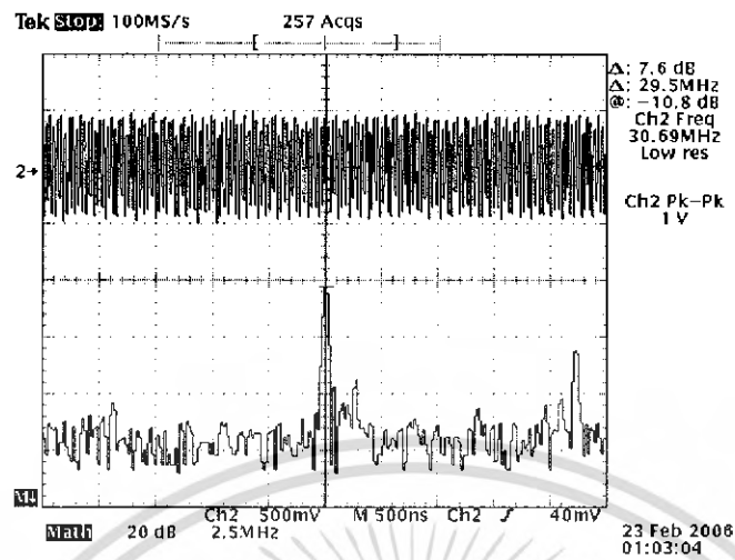
รูปที่ 4.18 สัญญาณที่ส่งออกมาจากวงจรส่งเดือนคว้นความถี่ 29 MHz
