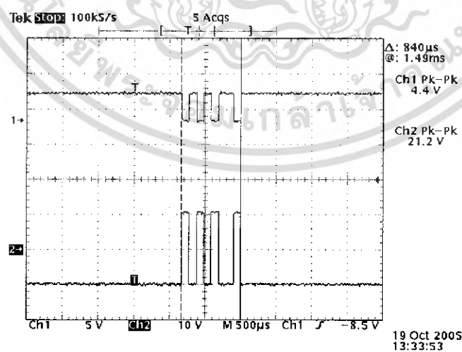
รูปที่ 4.1 สัญญาณเมื่อกดเดินหน้า ส่วนบนแสดงสัญญาณที่ออกมาจาก MAX-232
