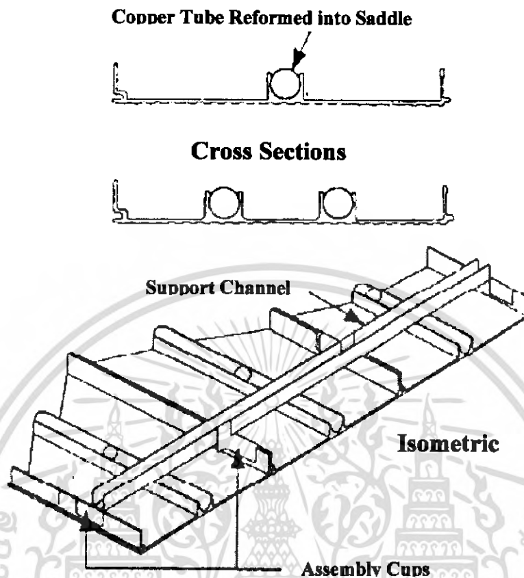
รูปที่ 3-4 แสดงส่วนประกอบของฝักคานโลหะแบบที่สาม
