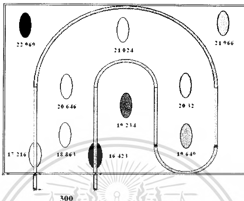
รูปที่ 5-7 ผลการทดลองที่ระยะห่างท่อแดง 300 มิลลิเมตร อุณหภูมิน้ำเข้าพลาทอน 16^{\circ}\text{C}
