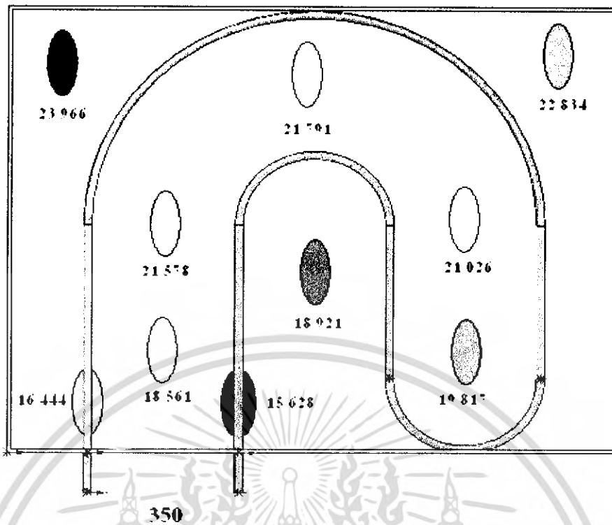
รูปที่ 5-2 ผลการทดลองที่ระยะห่างท่อทองแดง 350 มิลลิเมตร อุณหภูมิน้ำเข้าพาดาน 15^{\circ}C
