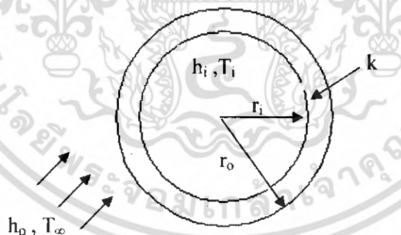
รูปที่ 3-10 ท่อกระบอกกฉนวนหุ้มฉนวน
