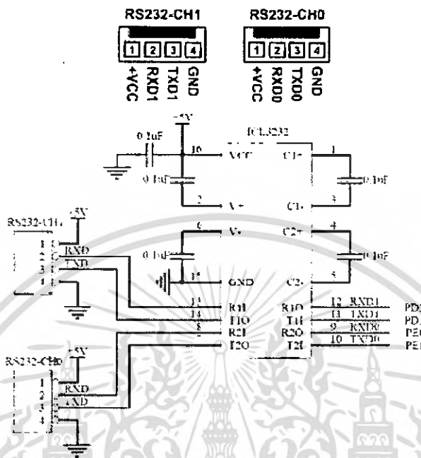
รูปที่ 2-11 แสดงวงจรขั้วต่อ RS232
