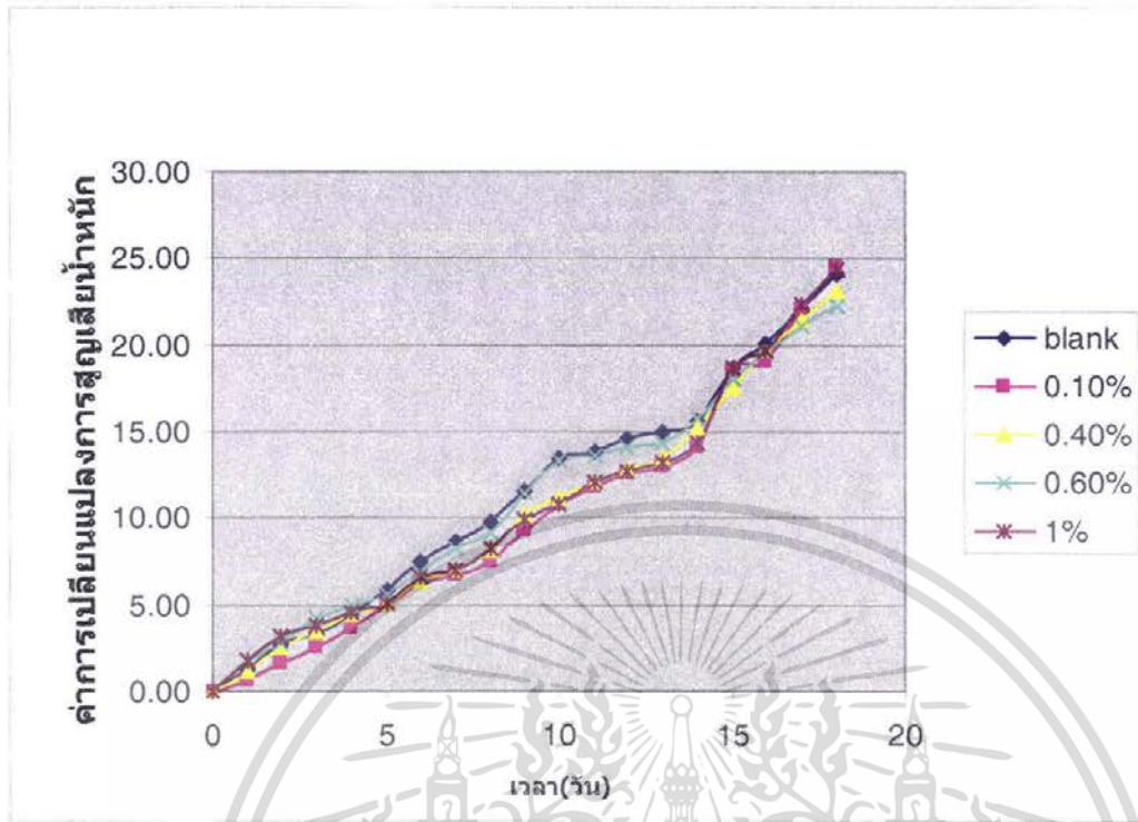
ภาพที่ 13 กราฟแสดงความสัมพันธ์ระหว่างค่าการเปลี่ยนแปลงการสูญเสียน้ำหนัก กับ วัน (ที่อุณหภูมิ 13°C)
