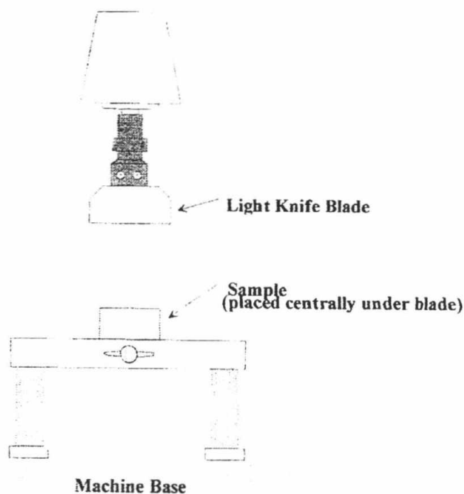
ภาพที่ 3.2 หัววัดแรงคัตชนิด hdp/bsk blade set with knife
