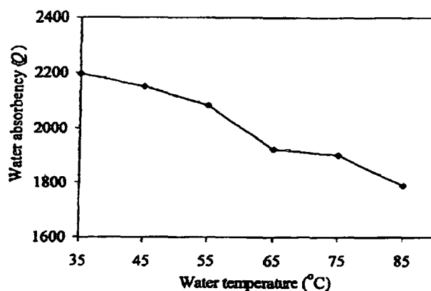
ภาพที่ 2.4 ผลของอุณหภูมิที่มีผลต่อความสามารถในการดูดซับน้ำของโพลีอะคริลิกแอซิด ที่มา: Ruthven, D.M (1984)
