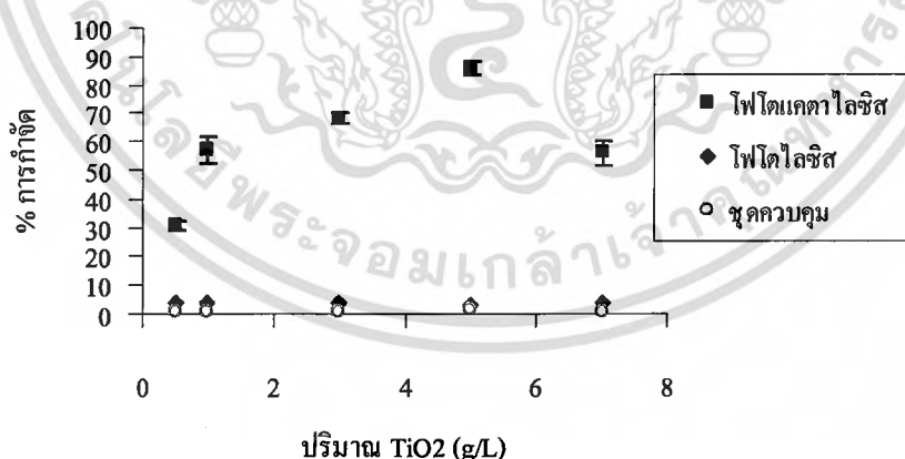
รูปที่ 4.4 กราฟแสดงเปอร์เซ็นต์การกำจัดสีข้อม RR141 ที่ปริมาณไทเทเนียมไดออกไซด์ต่างๆ
