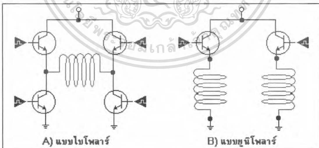
รูปที่ 2.17 วงจรการจ่ายไฟให้กับสเตปป์มอเตอร์
