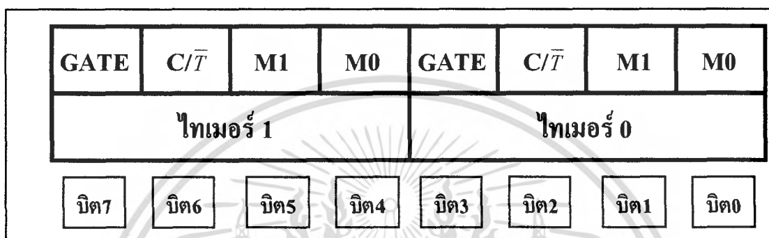
รูปที่ 2.7 รูปแบบของรีจิสเตอร์เลือกโหมดการทำงานของ ไทเมอร์/เคาน์เตอร์
