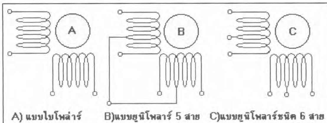
รูปที่ 2.16 การพันขดลวดบนสเตเตอร์ของสเตปป์มอเตอร์
