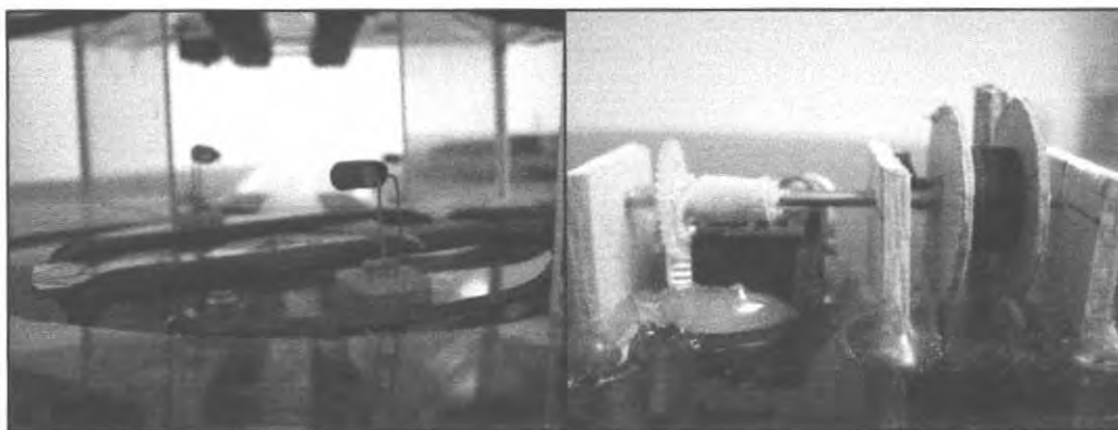
รูปที่ 3.9 ลิฟต์ยักและระบบขับเคลื่อนลิฟต์ยัก
