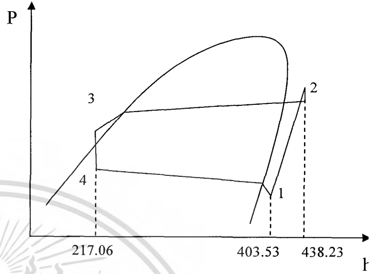
รูปที่ 4-1 กราฟค่าเอนทาลปีที่มีสภาวะมาตรฐาน ความถี่ 30 Hz
