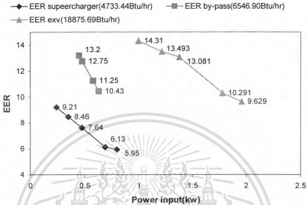
กราฟที่ 4-3 แสดงการเปรียบเทียบ ค่า EER จริงและกำลังที่ให้อจริง ระหว่างซูเปอร์ชาร์จเจอร์กับ คอมเพรสเซอร์ระบบต่างๆ
