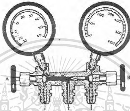
รูปที่ 3-35 แสดงภาพวาล์ว A อยู่ในตำแหน่งปิด วาล์ว B อยู่ในตำแหน่งเปิด
