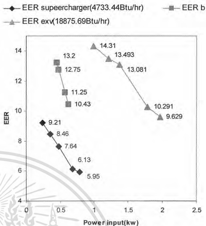
กราฟที่ 4-3 แสดงการเปรียบเทียบ ค่า EER จริงและกำลังที่ให้จริง ระหว่างซูเปอร์ชาร์จเจอร์กับคอมเพรสเซอร์ระบบต่างๆ
