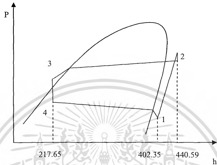
รูปที่ 4-2 กราฟค่าเอนทัลปีในสภาวะมาตรฐาน ความถี่ 35 Hz
