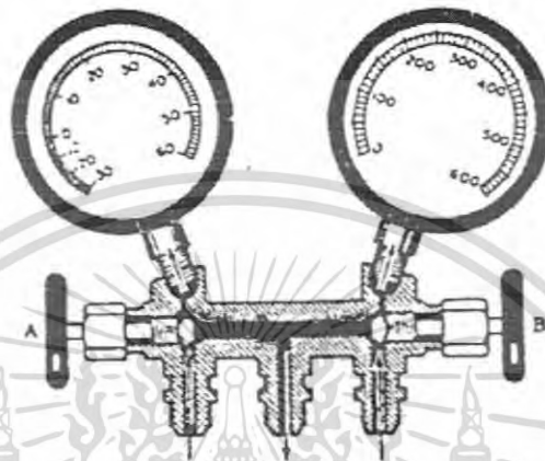
รูปที่ 3-33 แสดงภาพวาล์ว A วาล์ว B อยู่ในตำแหน่งปิดทั้งคู่
