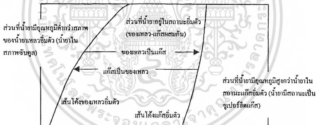
รูปที่ 2-6 แสดงโครงสร้าง P-h Diagram
