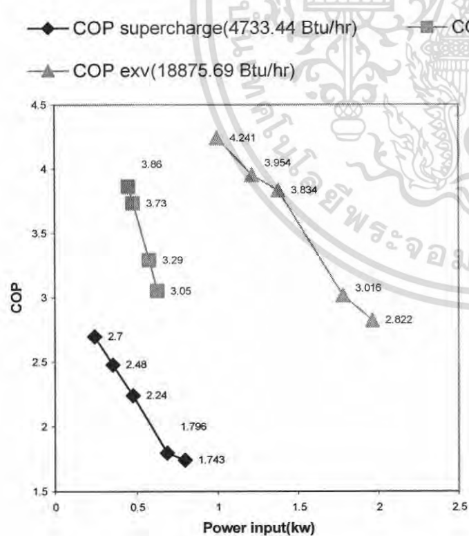
กราฟที่ 4-2 แสดงการเปรียบเทียบ ค่า COP จริงและกำลังที่ให้จริง
