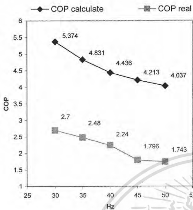
กราฟที่ 4-1 แสดงค่า COP ที่ความถี่ต่างๆ ที่สภาวะมาตรฐานของ ซูเปอร์ชาร์จเจอร์
