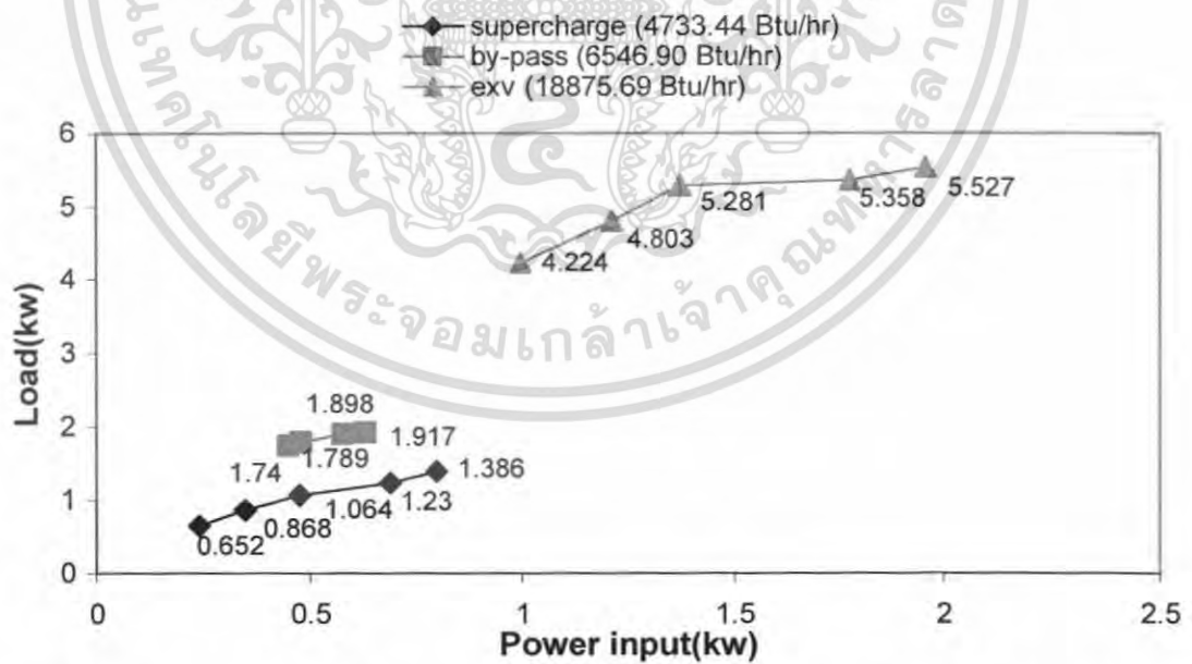
กราฟที่ 4-4 แสดงการเปรียบเทียบงานที่ให้กับภาระการทำความเย็นระหว่างซูเปอร์ชาร์จเจอร์กับ คอมเพรสเซอร์ระบบต่างๆ
