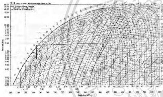
รูปที่ 2-3 P-h diagram ของสารทำความเย็น R-11
