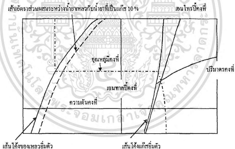
รูปที่ 2-7 แสดงโครงสร้าง P-h Diagram เส้นความดันคงที่ อุณหภูมิมิคงที่ ปริมาตรคงที่และเอนทัลปี
