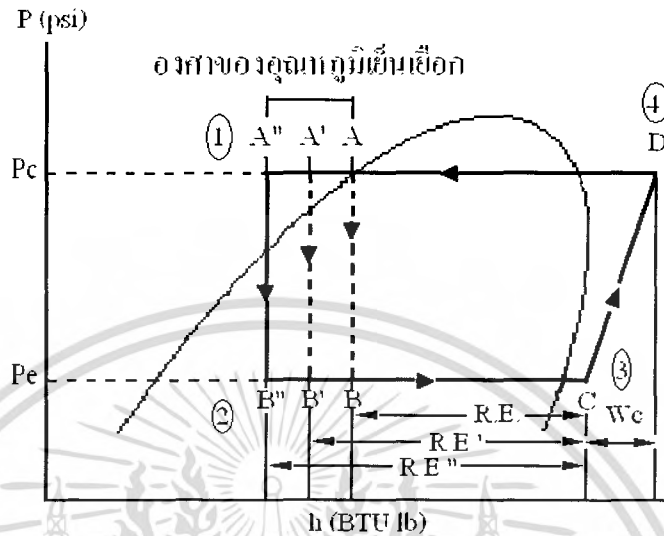
รูปที่ 2-9 แผนภูมิความดันและเอนทาลปีเปรียบเทียบวัฏจักรของเหลวอิมตัวกับต่ำกว่าของเหลวอิมตัว
