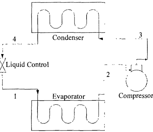
รูปที่ 2-1 แสดงระบบการอัดไอแบบธรรมดา
