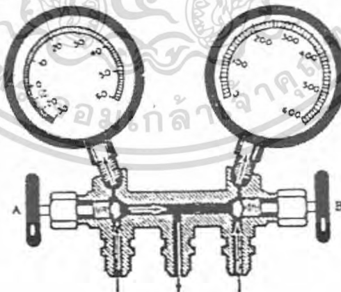
รูปที่ 3-34 แสดงภาพวาล์ว A อยู่ในตำแหน่งเปิด วาล์ว B อยู่ในตำแหน่งปิด
