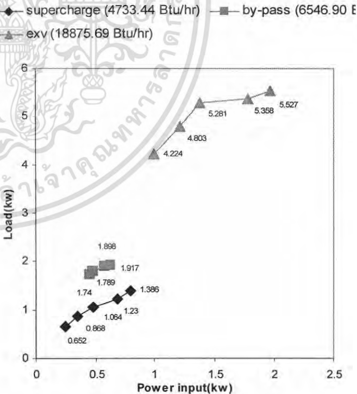
กราฟที่ 4-4 แสดงการเปรียบเทียบงานที่ให้กับภาระการทำความเย็น
