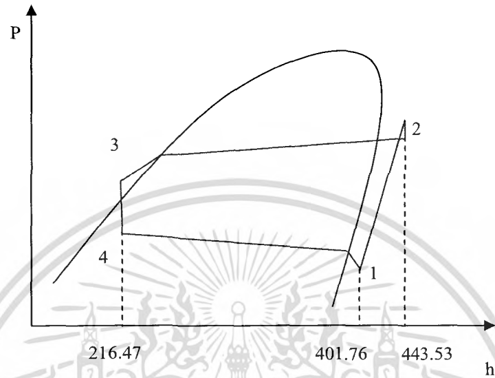
รูปที่ 4-3 กราฟค่าเอนทัลปีในสภาวะมาตรฐาน ความถี่ 40 Hz
