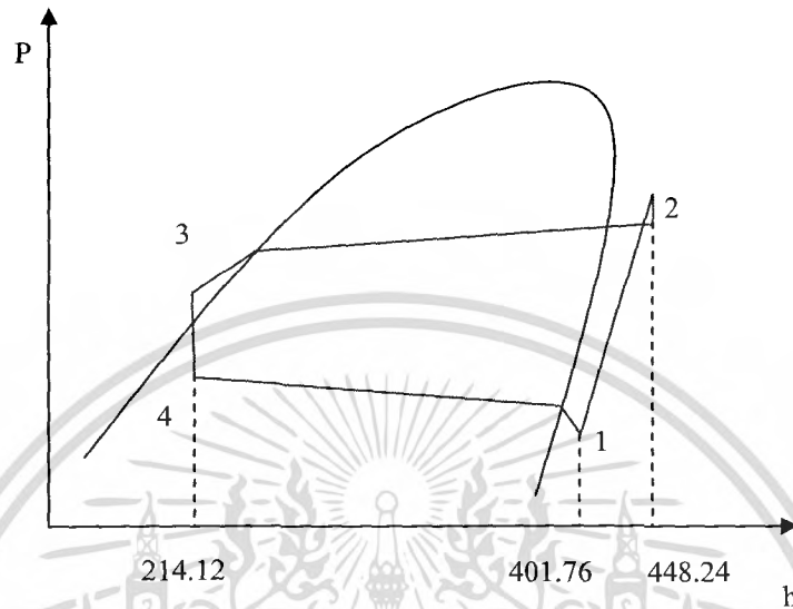
รูปที่ 4-5 กราฟค่าเอนทัลปีในสถานะมาตรฐาน ความถี่ 50 Hz
