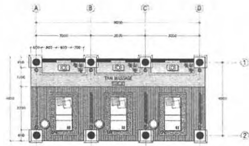
HERBAL HUT THAIMASSAGE SCALE 1 : 50
