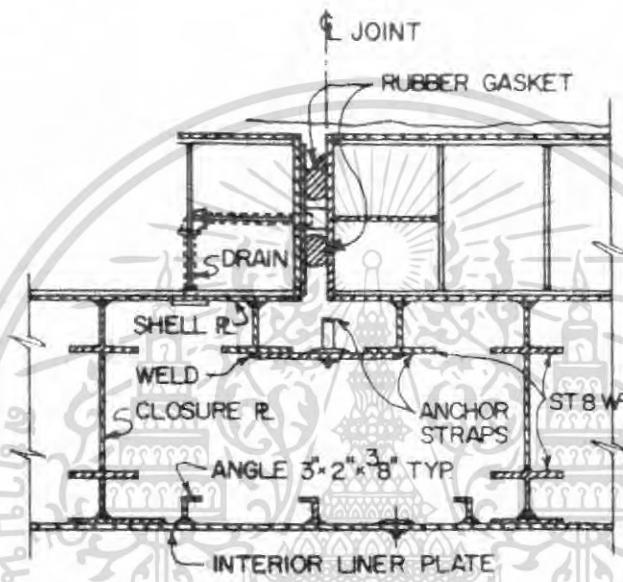
รูปภาพที่ 7.24 แสดงรอยต่ออย่างชนิดแผ่นรองคู
