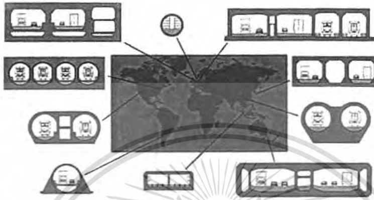
รูปภาพที่ 7.25 แสดงหน้าตัดที่หลากหลายของอุโมงค์ประกอบได้นำ
