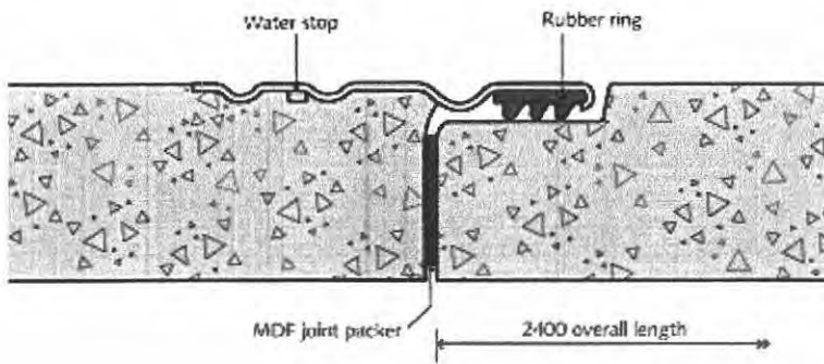
รูปภาพที่ 5.5 แสดง CS pipe joint ของการค้นท่อ
