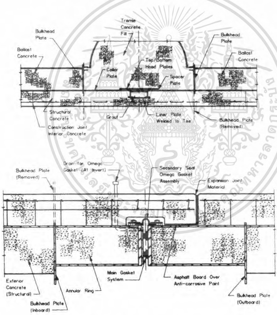
รูปภาพที่ 7.22 แสดงรายละเอียดของรอยต่อทรีมี
