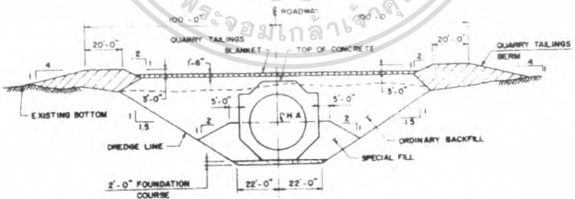
รูปภาพที่ 7.15 แสดงแนวอุโมงค์ที่ถูกขุดลอกและฉีคสารเพื่อป้องกันแนวเหนือพื้น
