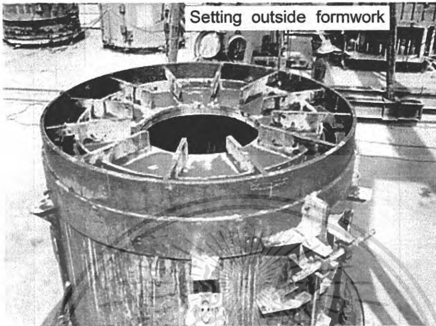
รูปภาพที่ 6. 5 แสดงแบบภายนอกที่นำมาประกบโครงเหล็ก
