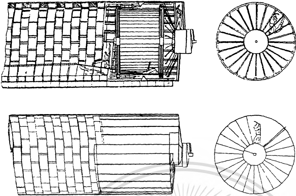
รูปถ่ายที่ 4.1 Marc Brunel's "screw" shield (1818)
