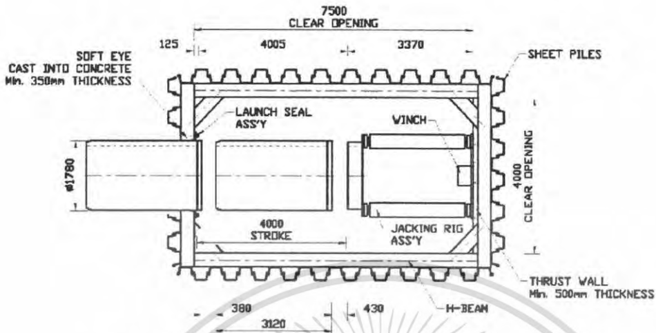
รูปภาพที่ 6.10 แสดงตัวอย่างแบบก่อสร้างบ่อคั่น
