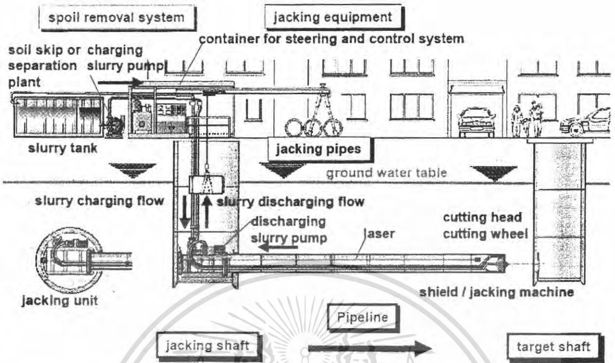
รูปภาพที่ 3.1 แสดงตัวอย่างส่วนประกอบต่างๆในการค้ำท่อ
