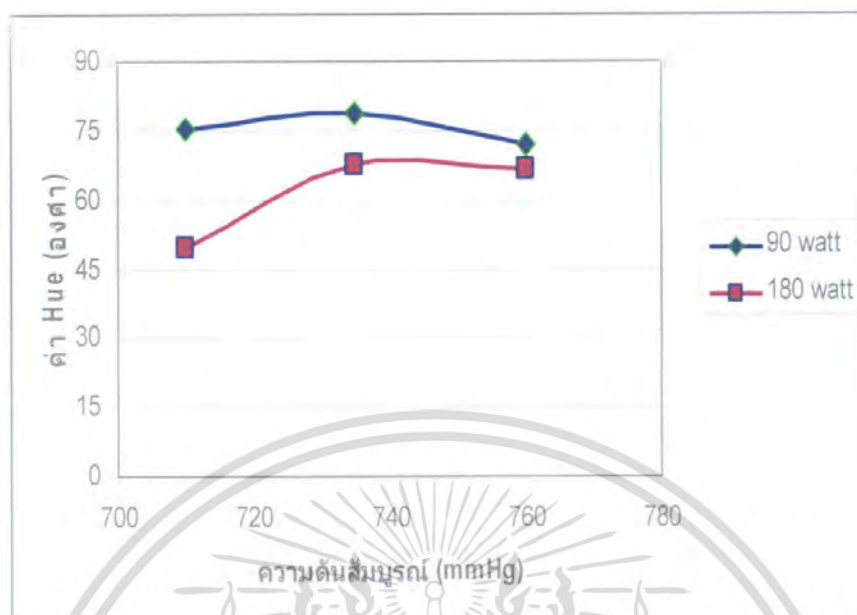
รูปที่ 4.11 กราฟแสดงความสัมพันธ์ระหว่างความดันสัมพันธ์และค่า Hue ของผลิตภัณฑ์ที่ระดับกำลังไมโครเวฟ 2 ระดับ ของตัวอย่างชุดที่ 1
