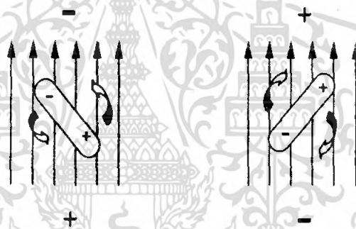
รูปที่ 2.6 การหมุนตัวของสารประกอบมีประจุเนื่องจากไมโครเวฟ ที่มา: คณาจารย์ภาควิชาวิทยาศาสตร์และเทคโนโลยีอาหาร(2543)
