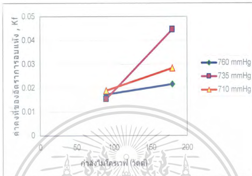
รูปที่ 4.5 กราฟแสดงความสัมพันธ์ระหว่างค่าคงที่ของอัตราการอบแห้งกับกำลังไมโครเวฟที่ระดับความดันต่างๆ ของตัวอย่างชุดที่ 1
