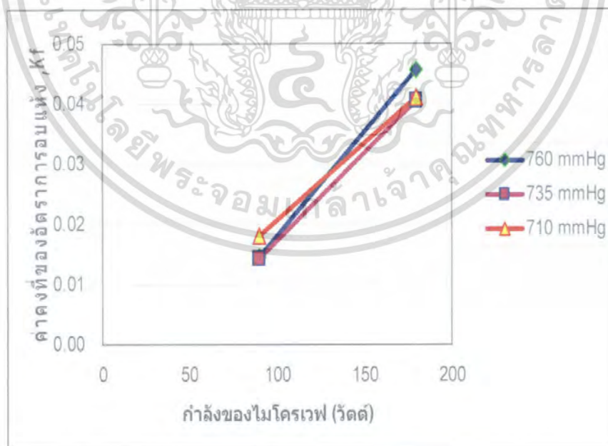
รูปที่ 4.6 กราฟแสดงความสัมพันธ์ระหว่างค่าคงที่ของอัตราการอบแห้งและกำลังไมโครเวฟที่ระดับความดันต่างๆ ของตัวอย่างชุดที่ 2
