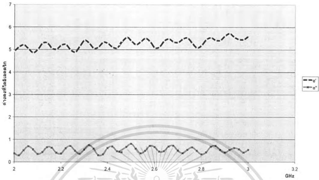
ค่าคงที่ไดอิเล็กตริก(เปลือกนอก)ของสัณฐานที่3
