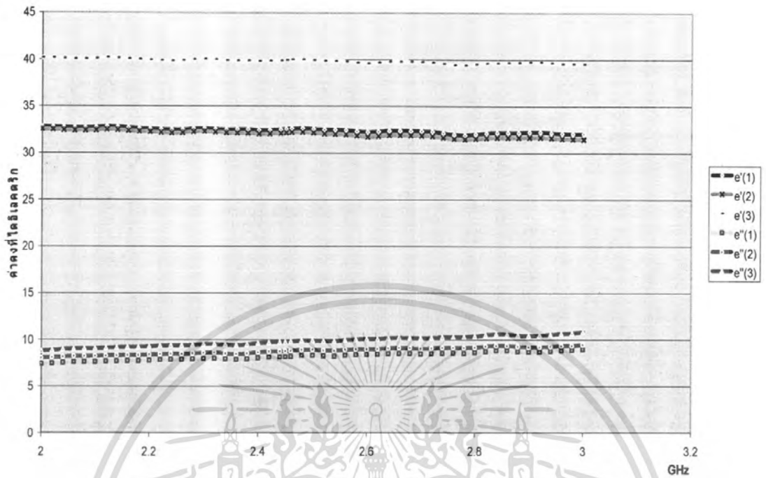
ความถี่ (ข) เนื้อส้ม กราฟแสดงค่าคงที่ไดอิเล็กตริก(เปลือกนอก)ของส้มลูกที่4
