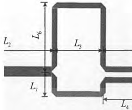
รูปที่ 3.3 ส่วนของบาลัน
