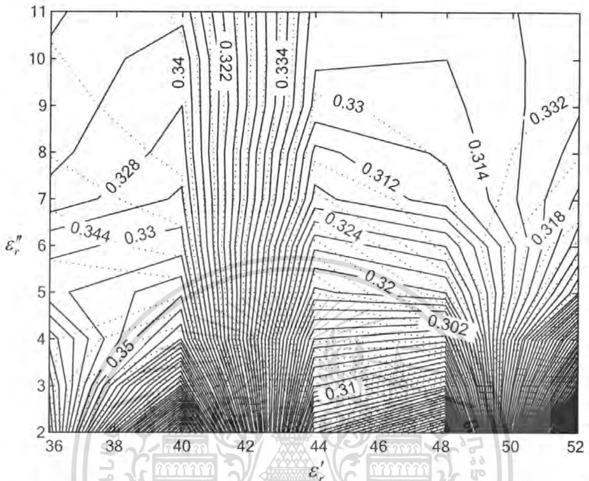
รูปที่ 4.10 กราฟเชิงพื้นผิวของขนาดการเชื่อมต่อกันของสายอากาศโคโพลบนแผ่นพิมพ์ในกรณีขนานและตั้งฉาก (จุดปะคือกรณีขนาน (...) เส้นทึบคือกรณีตั้งฉาก (-))
