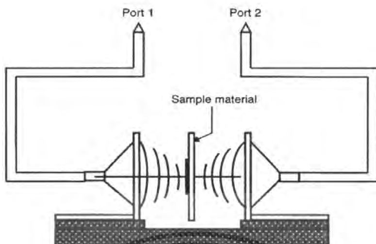
รูปที่ 2.11 เทคนิคอวกาศสว่าง โดยที่พอร์ตหนึ่งและพอร์ตสองต่ออยู่กับเครื่องวิเคราะห์ห้วงจรข่าย [4]
