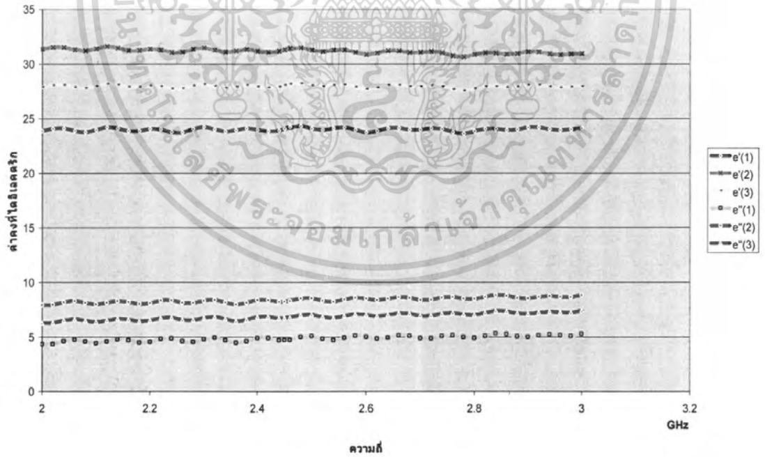
กราฟแสดงค่าคงที่ไดอิเล็กตริก(เนื้อ+เปลือก)ของสัมลุกที่4
