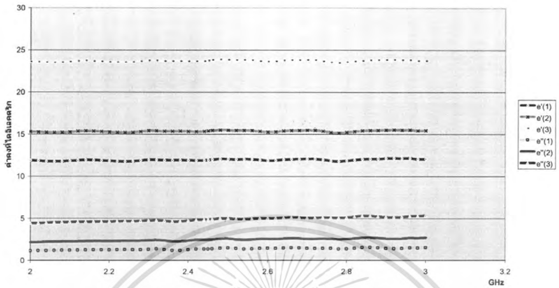
กราฟแสดงค่าคงที่ไดอิเล็กตริก(เนื้อ+เปลือก)ของสัมลุกที่5
