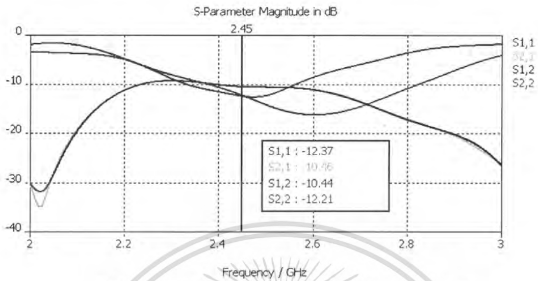
รูปที่ 3.15 ค่าความสูญเสียย้อนกลับในกรณีติดตั้งฉากที่รวมอิทธิพลของมือ
