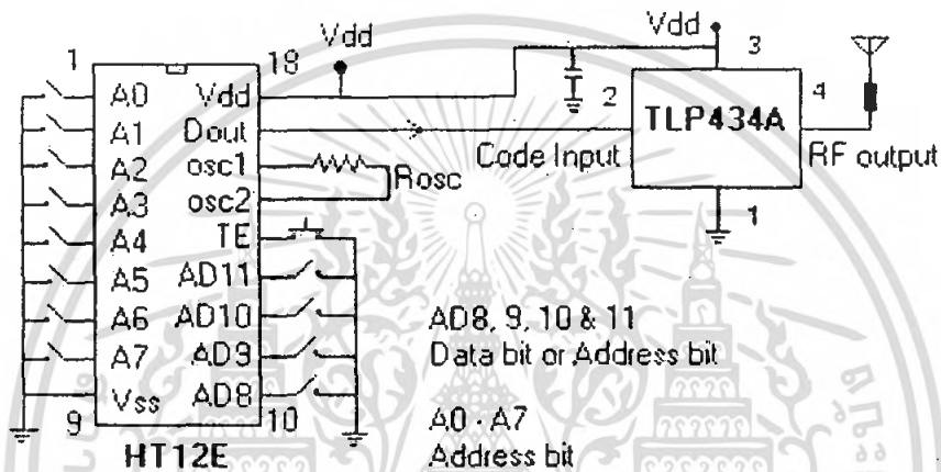
รูป 3.14 การต่อไอซีเข้ารหัสร่วมกับ โมดูล
