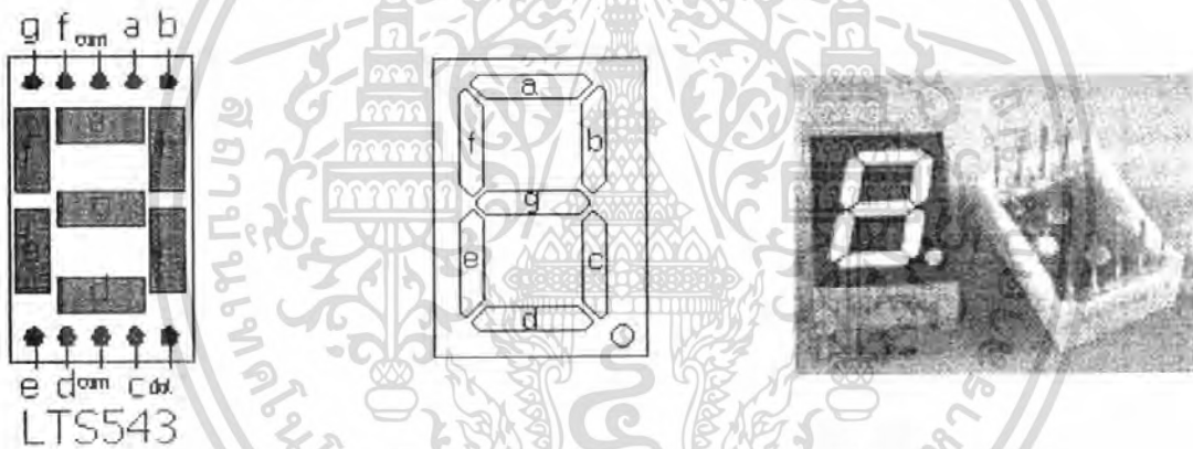
รูปที่ 3.5 แสดงการแบ่งขั้ว ส่วนทั้ง 7 ส่วนและ รูปของหลอดแสดงผล 7 ส่วน
