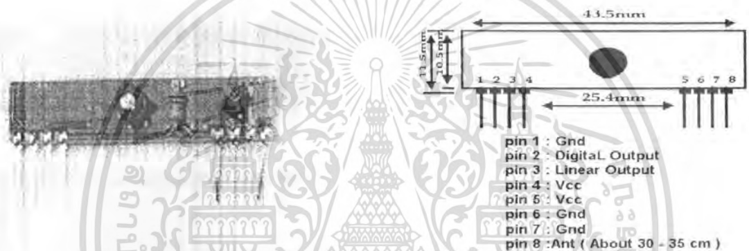
รูปที่ 3.13 รูปอุปกรณ์ของ RLP434A
