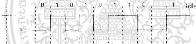
รูปที่ 2.9 แสดงการสื่อสารแบบอะซิงโครนัสที่ใช้พาริตีบิต
