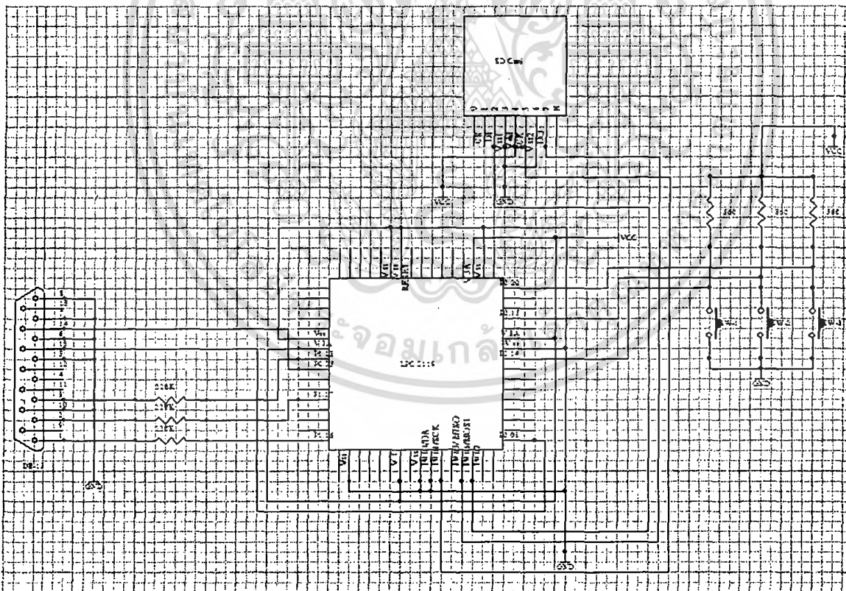
รูปที่ 3.5 วงจรการติดต่อ SD Card, DB-15 และ ARM7 เบอร์ LPC2119
