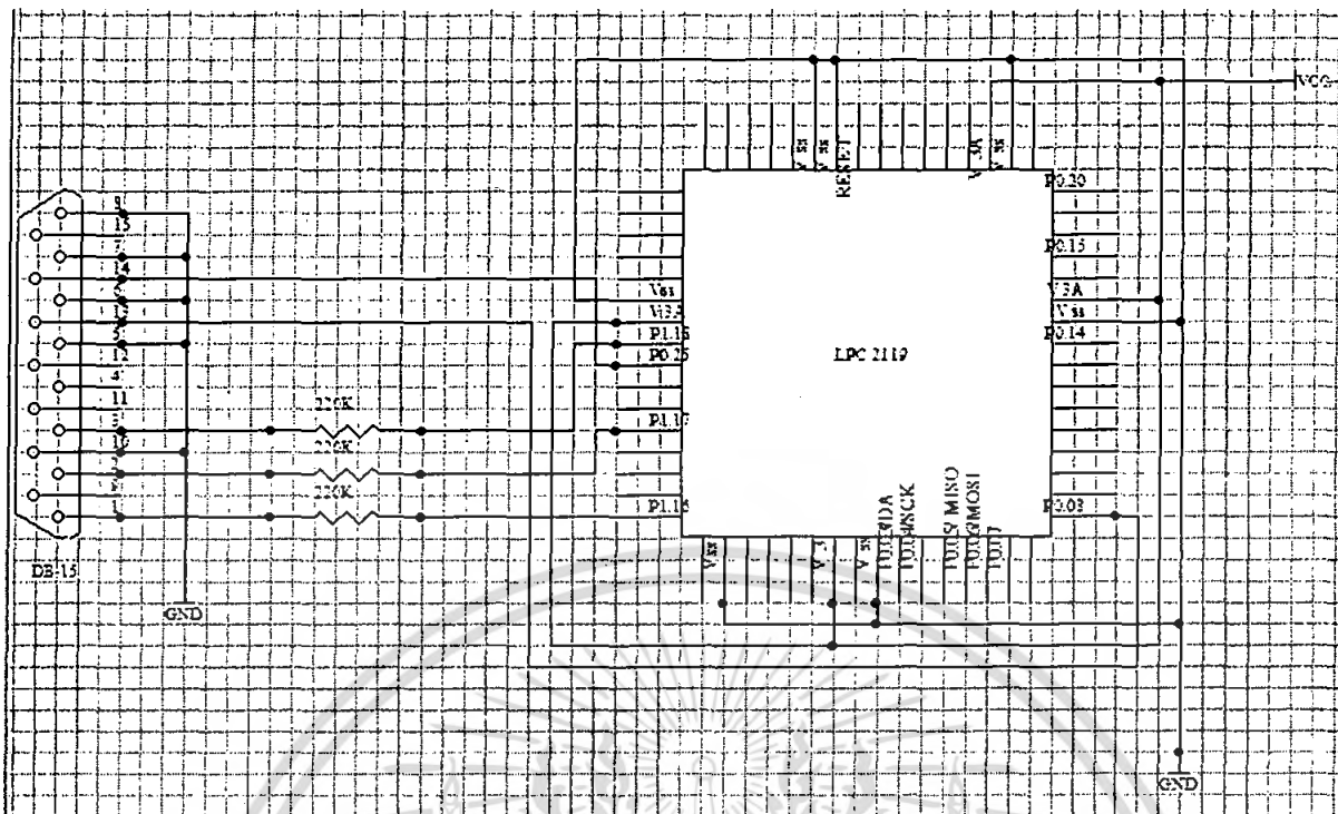
รูปที่ 3.4 วงจรการติดต่อระหว่าง DB-15 กับ ARM7 เบอร์ LPC2119
