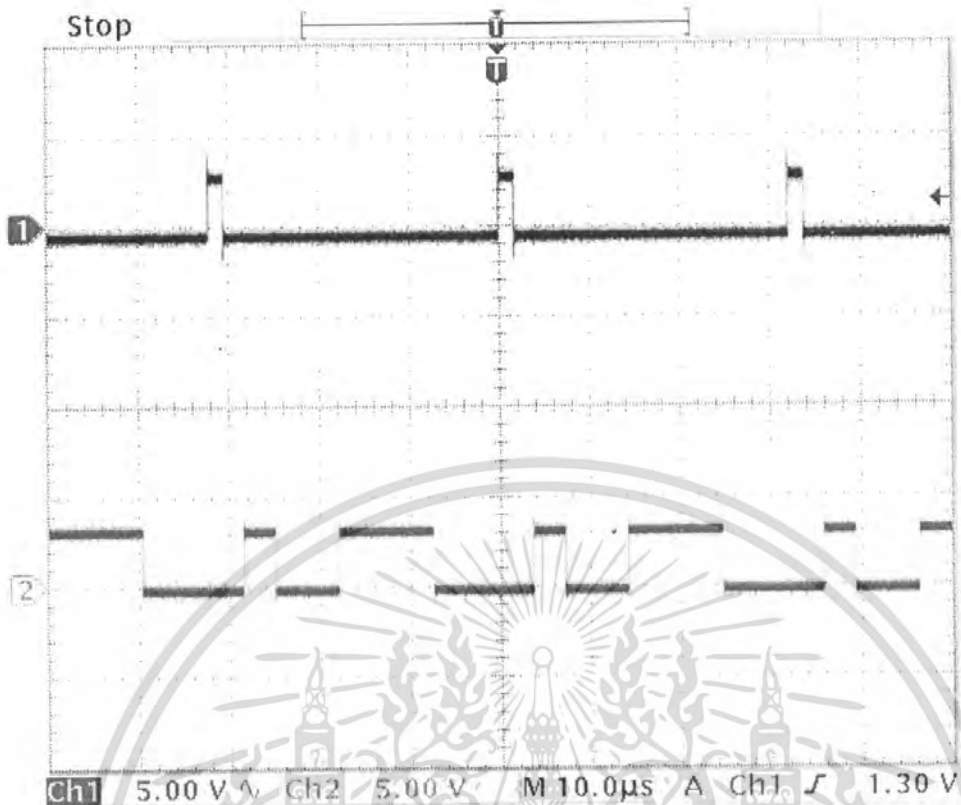
รูปที่ 4.14 รูปสัญญาณ HSync เทียบกับ Green
