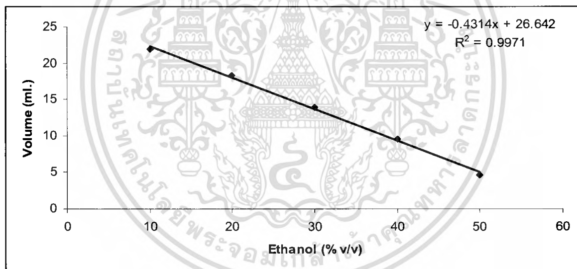
รูปที่ 4.11 จากกราฟแสดงค่า R^2 จากความสัมพันธ์ระหว่างความเข้มข้นของสารละลายมาตรฐาน เอทานอลกับปริมาตรของสารละลายโซเดียมไทโอซัลเฟต ความเข้มข้น 0.05 M
