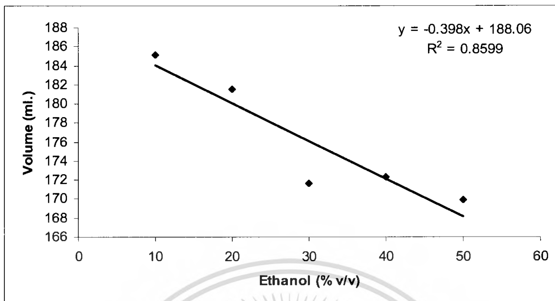
รูปที่ 4.8 จากกราฟแสดงค่า R^2 จากความสัมพันธ์ระหว่างความเข้มข้นของสารละลายมาตรฐานเอทานอลกับปริมาตรของสารละลายโซเดียมไทโอซัลเฟต ความเข้มข้น 0.01 M จากผลการทดลองแสดงค่า R^2 = 0.8599
