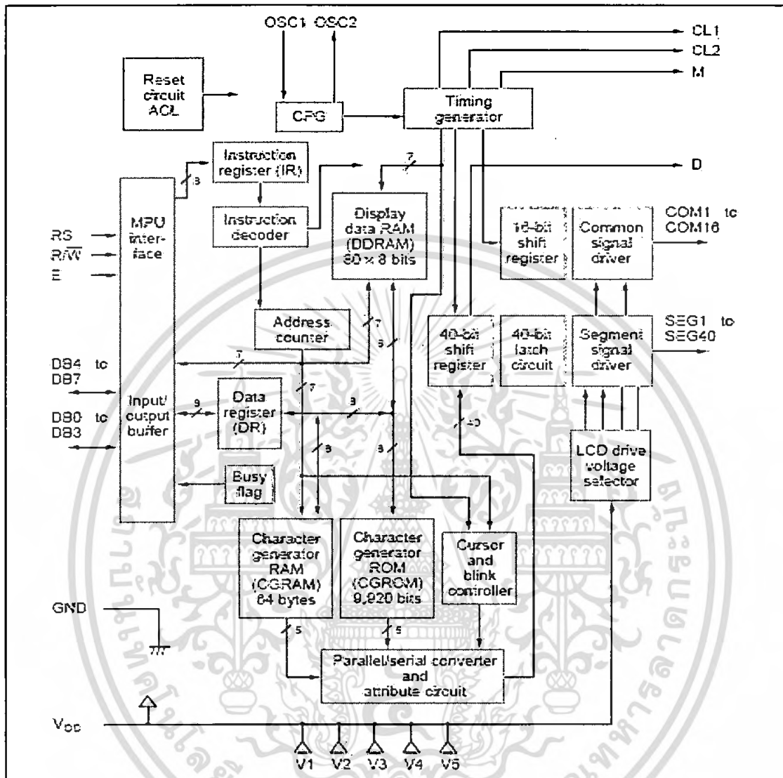
รูปที่ 3.5 แสดงไดอะแกรมการทำงานของโมดูล LCD แบบอักษร
