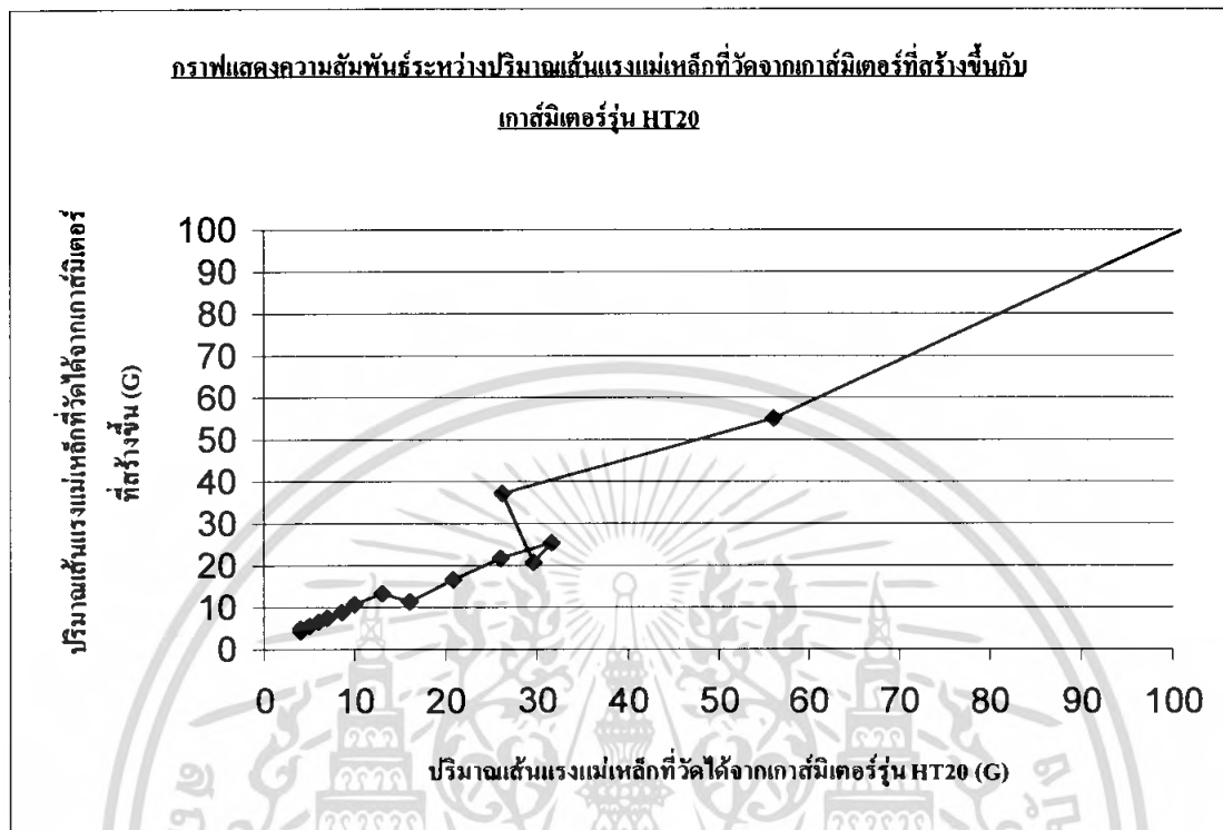
รูปที่ 5.3 กราฟแสดงความสัมพันธ์ระหว่างปริมาณเส้นแรงแม่เหล็กที่วัดได้จากแก๊สไมเตอร์ที่สร้างขึ้นกับแก๊สไมเตอร์รุ่น HT20 ช่วง 0-100 G
