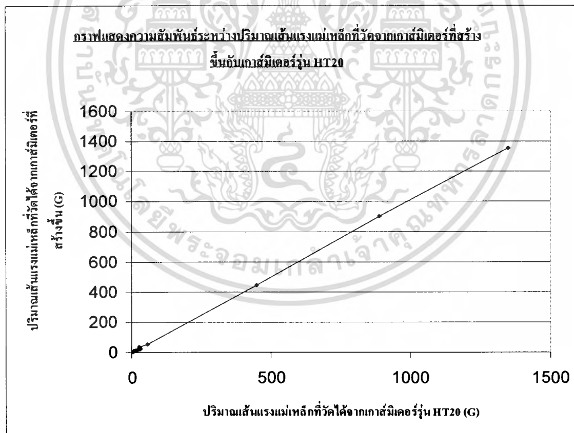
รูปที่ 5.2 กราฟแสดงความสัมพันธ์ระหว่างปริมาณเส้นแรงแม่เหล็กที่วัดได้จากเกาส์มิเตอร์ที่สร้างขึ้นกับเกาส์มิเตอร์รุ่น HT20
