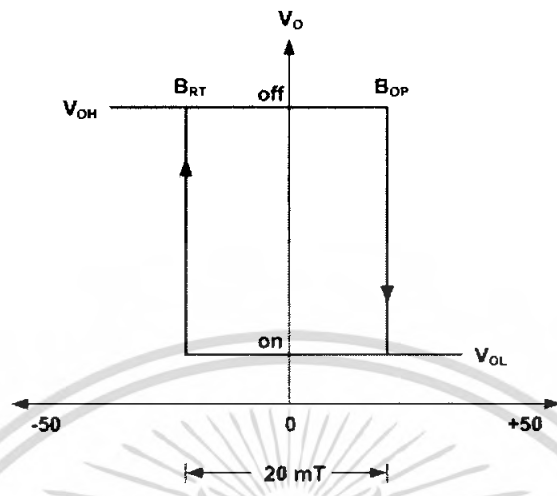
รูปที่ 2.6 การตอบสนองแรงดันเอาต์พุตกับสนามแม่เหล็กของฮอลล์ชนิดแลตซ์
