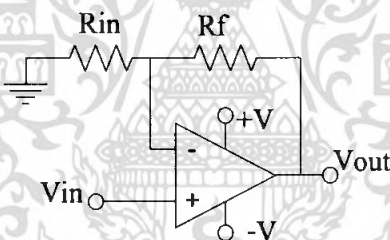
รูปที่ 4.4 วงจรขยายแบบไม่กลับเฟส (Non inverting Amplifier)
