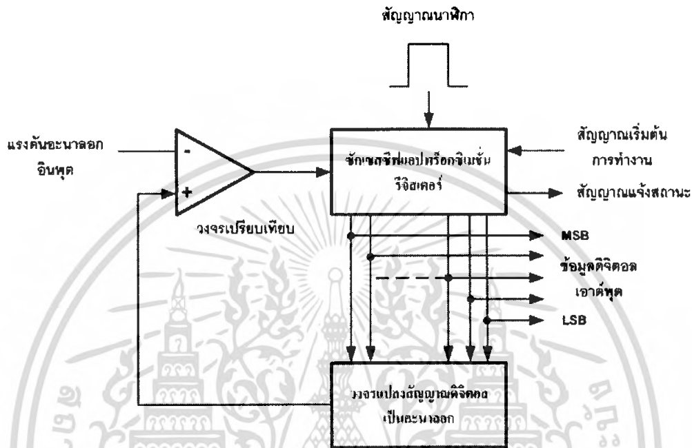
รูปที่ 3.3 แสดงไคอะแกรมการทำงานของวงจร ADC แบบซิกเซตซีฟแอฟหรือกิมเมชั่น
