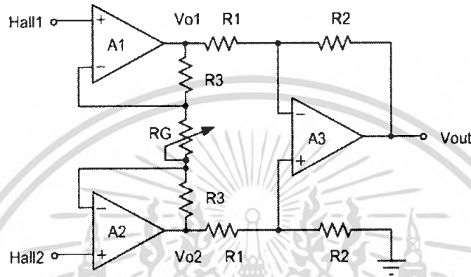
รูปที่ 4.2 วงจรขยายสัญญาณอินสทรูเมนต์แบบใช้ออปแอมป์ 3 ตัว
