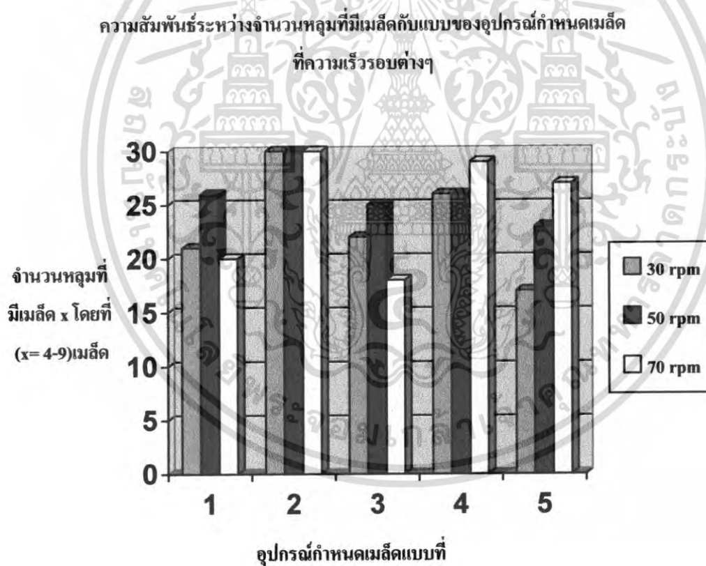
รูปที่ 4.17 กราฟแสดงความสัมพันธ์ระหว่างจำนวนหลุมที่มีเมล็ดกับแบบของอุปกรณ์กำหนดเมล็ดที่ความเร็วรอบต่างกัน
