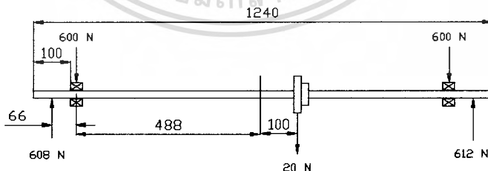
รูปที่ 3.6 แสดงแบบของเพลาลับ
