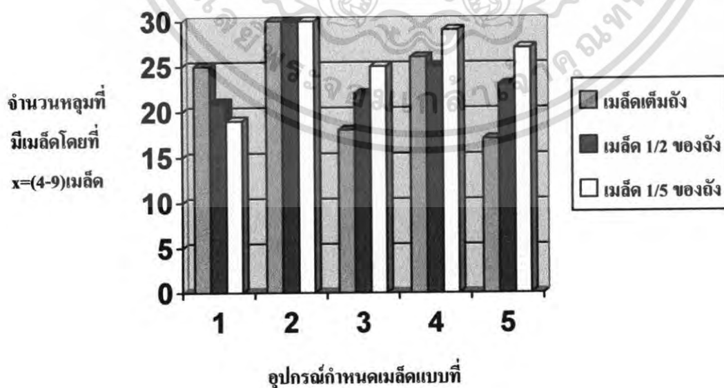
รูปที่ 4.11 กราฟแสดงความสัมพันธ์ระหว่างจำนวนหลุมที่มีเมล็ด x_{-1}^{+2} กับแบบของอุปกรณ์กำหนดเมล็ดในเอกสารนี้เป็นเอกสารที่สงวนไว้สำหรับการใช้งานเพื่อการศึกษาเท่านั้น ไม่อนุญาตให้นำไปใช้ประโยชน์ด้านการค้า ไม่ว่ากรณีใดๆ ทั้งสิ้น อีกทั้งห้ามมิให้ตัดแปลงเนื้อหา และต้องอ้างอิงถึงเจ้าของเอกสารทุกครั้งที่มีการนำไปใช้
